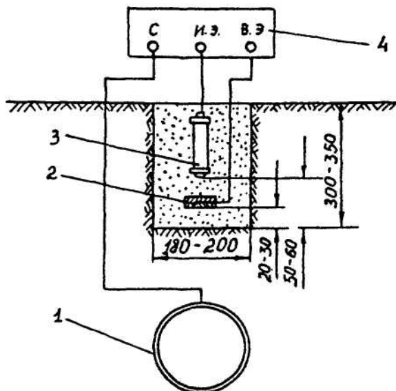
Рис. 4.7.2 Схема измерения поляризационного потенциала на нестационарных КИПах
