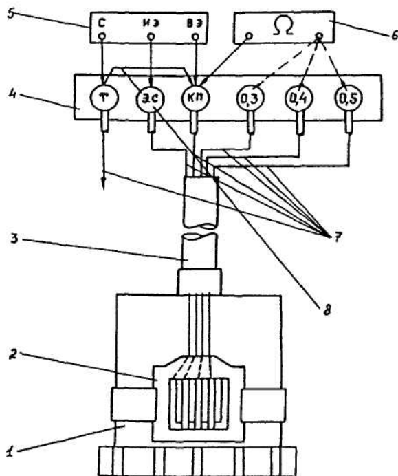
Рис. 03 Схема контроля электропроводимости индикаторов и измерения поляризационного потенциала трубопровода при установке блока индикаторов на стационарном электроде сравнения
