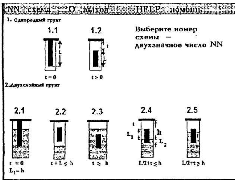
Рис. С1. К программе CAG: схема возможных расположений вертикального анода в однородном (1.1, 1.2) и двухслойном грунтах (2.1 - 2.5) для выбора расчетного варианта
