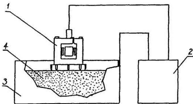
Рис. 4.4.1 Схема измерения переходного электрического сопротивления электродов сравнения
