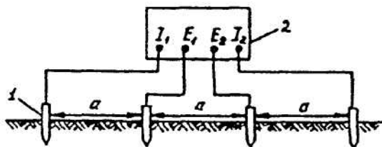
Рис. 4.2.1 Схема определения удельного сопротивления грунта
