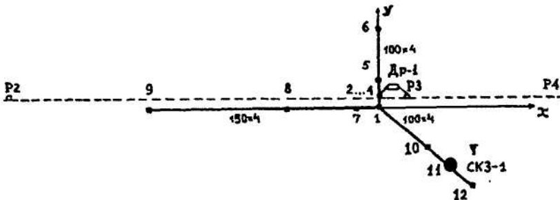
Рис. PI. Схема трубопроводов и рельсового пути к примеру расчета ЭХЗ по программе АРМ ЭХЗ-6П
