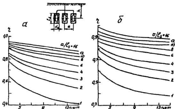
Рис. У1. Зависимость коэффициента использования ( \gamma ) анодов группы ГА от количества ( n ) анодов в группе и отношения a/l_3 межанодного расстояния ( a ) к длине ( l_3 ) комплектного анода
