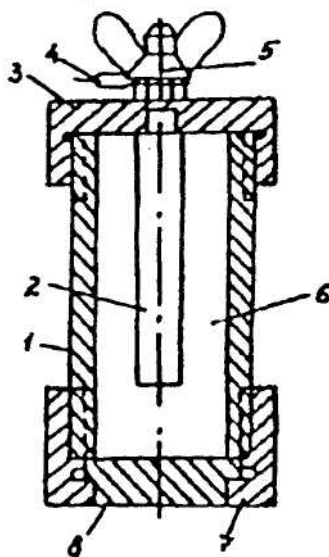
Рис. 4.2.3 Переносной медносульфатный электрод сравнения
