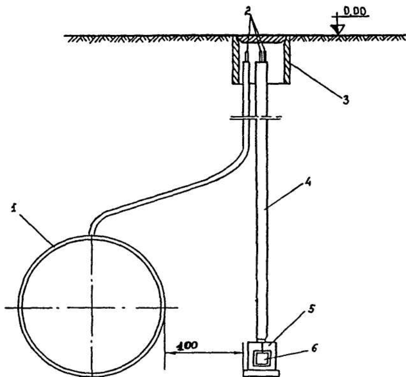
Рис. 4.3.1 Устройство стационарного контрольно-измерительного пункта с медносульфатным электродом сравнения длительного действия
