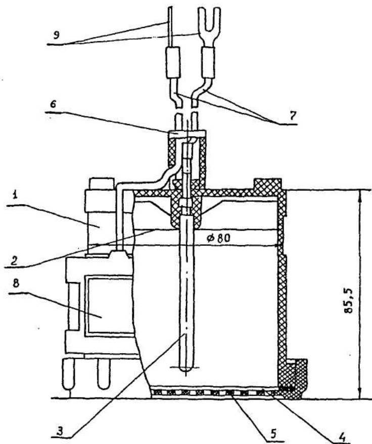
Рис. III. Стационарный медносульфатный электрод сравнения типа ЭНЕС-1 и ЭСН-МС
