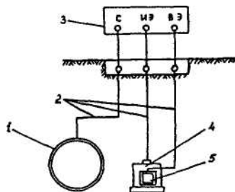
Рис. 4.7.1 Схема измерения поляризационного потенциала на стационарных КИПах
