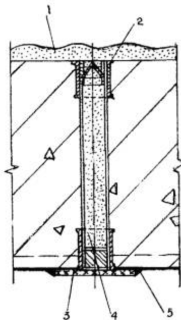
Рис. 4. Заделка отверстий для нагнетания бентонитового раствора труб диаметром 2000 мм:
