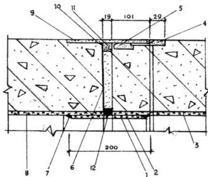
Рис. 2. Конструкция стыка труб диаметром 1200 и 1500 мм:
