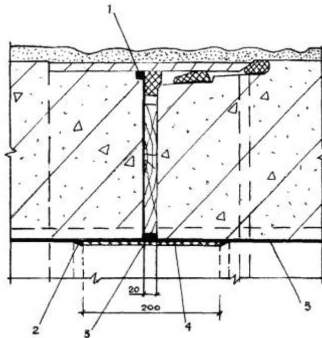
Рис. 3. Конструкция стыка труб диаметром 2000 мм:
