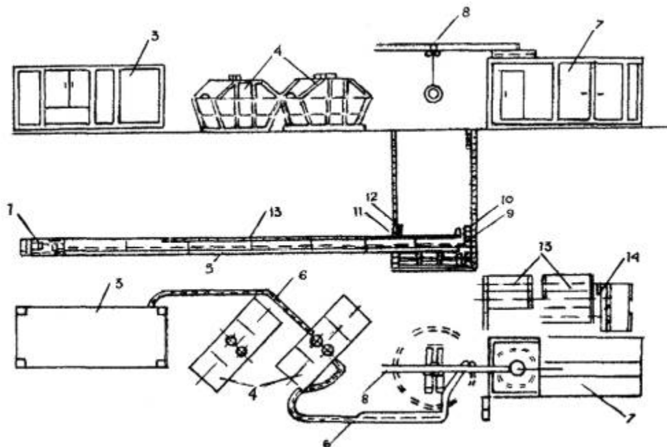
Рис. 5. Конструкторско-технологическая схема МТПК 1-го вида для прокладки труб диаметром от 250 до 600 мм (фирма «Нозль») с пневмотранспортировкой разработанной породы:
