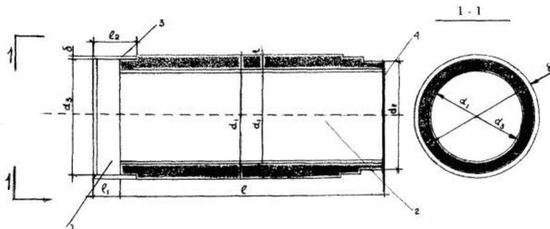
Рис. 1. Форма и принципиальная конструкция железобетонной трубы с внутренней полиэтиленовой оболочкой:
