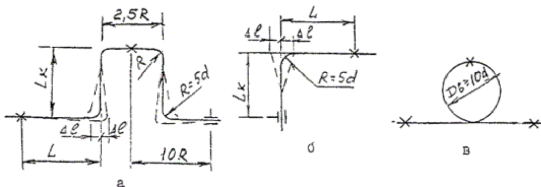
Рис. 4. Устройство компенсаторов:
