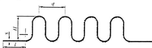
Рис. п.4.1. Гибкий элемент компенсатора
