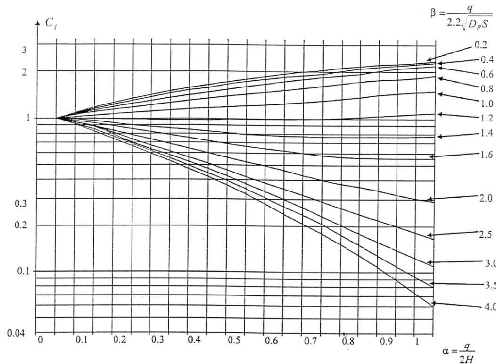
Рис. п.4.4. Графики для определения коэффициента C_f
