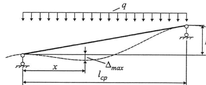
Рис. п.1.1. Схема прогибов трубопровода под равномерно-распределенной нагрузкой
