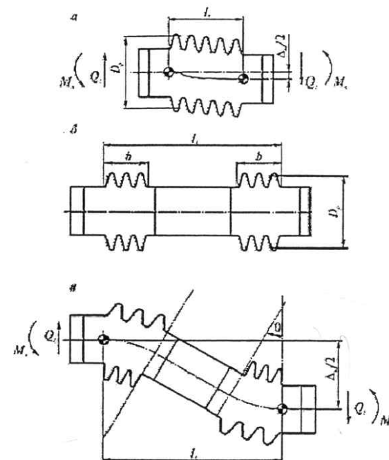
Рис. п.4.3 Схемы сдвиговых компенсаторов: а- без промежуточной вставки, б – с промежуточной вставкой-трубой
