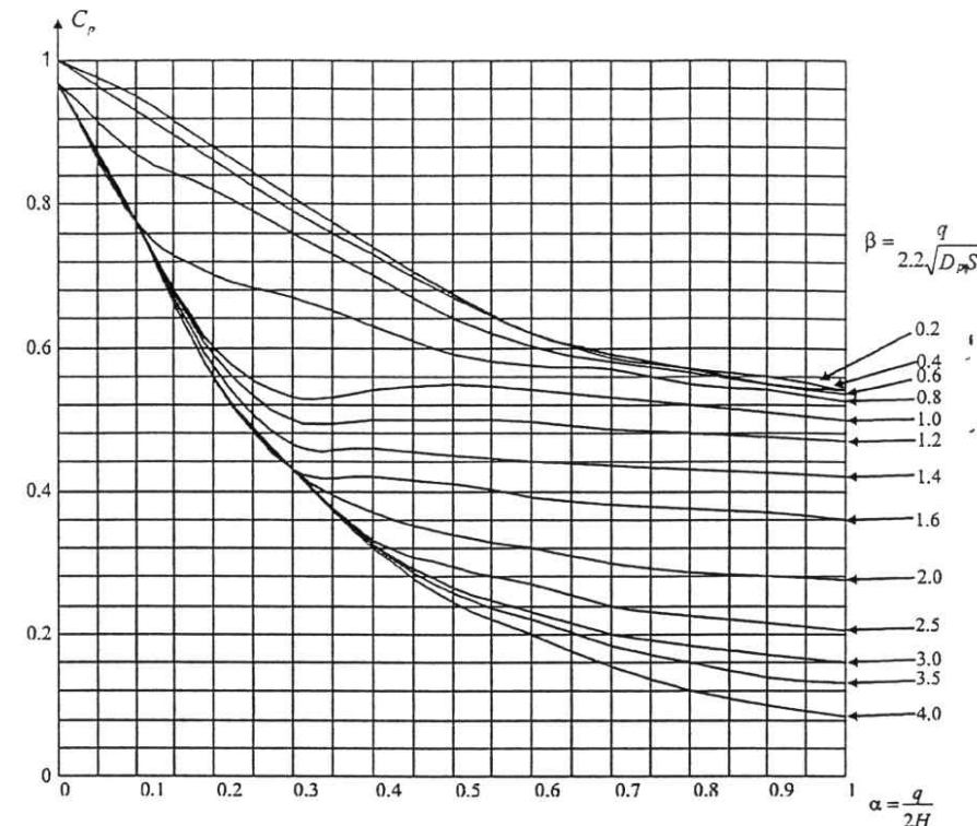
Рис. п.4.6. Графики для определения коэффициента C_p
