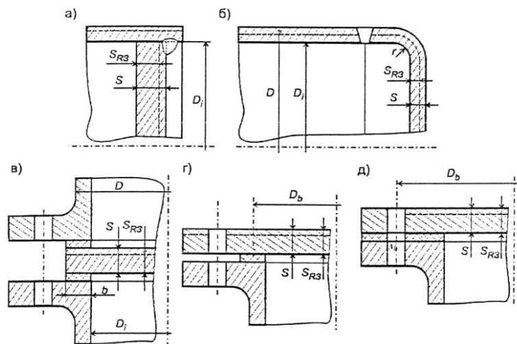
Рис. 3.4. Круглые плоские заглушки: а – внутритрубная; б – торцевая; в – межфланцевая; г, д – фланцевая
