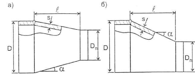
Рис. 3.2. Переходы: а - концентрический, б - эксцентрический
