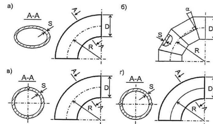
Рис. 3.1. Отводы: а - гнутый; б - секторный; в, г - штамповарной
