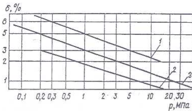
Рис. 4. Зависимость допускаемой степени неравномерности давления \delta в газопроводах.
