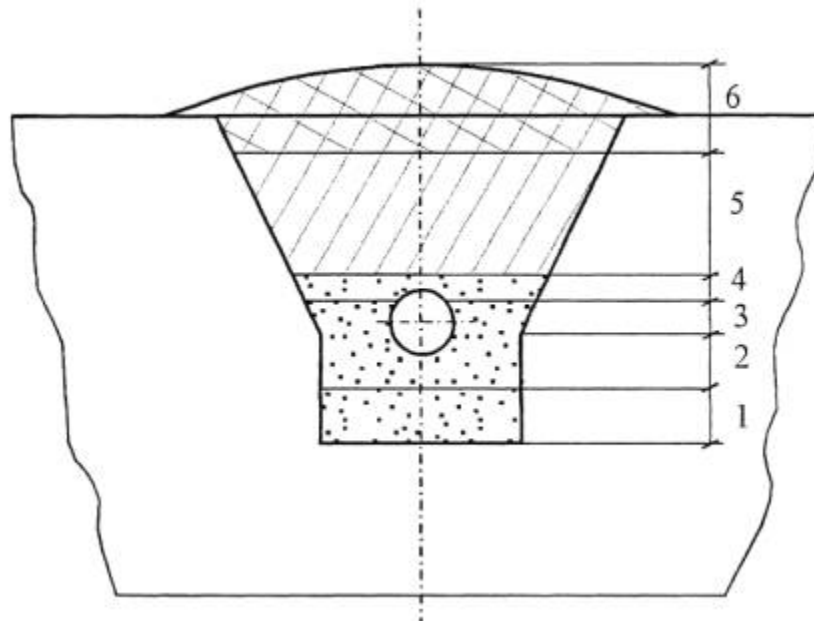
Рис. 7.3. Поперечное сечение траншеи с уложенным трубопроводом на слабонесущих грунтах
