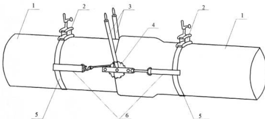
Рис. 12.1. Схема сборки раструбных и муфтовых соединений
