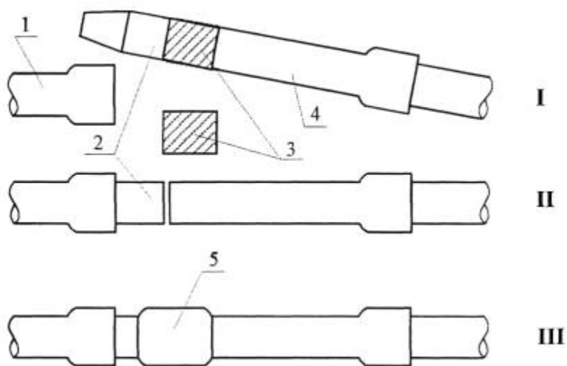
Рис. 12.3 Три этапа ликвидации «захлеста»
