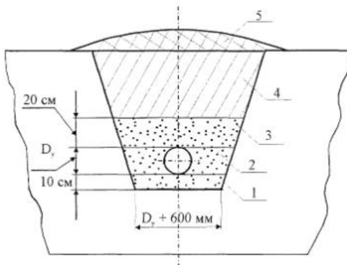
Рис. 7.1. Прокладка стеклопластикового трубопровода по суходолу (в сухом грунте)
