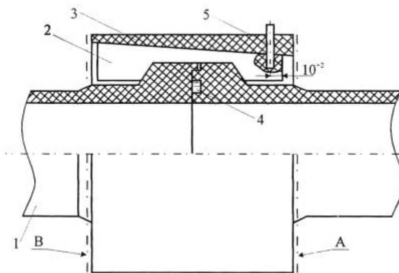
Рис. 12.2. Сборка бугельного стыка
