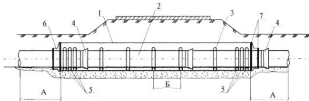
Рис. 7.4. Конструкция перехода трубопровода через дорогу в защитном кожухе
