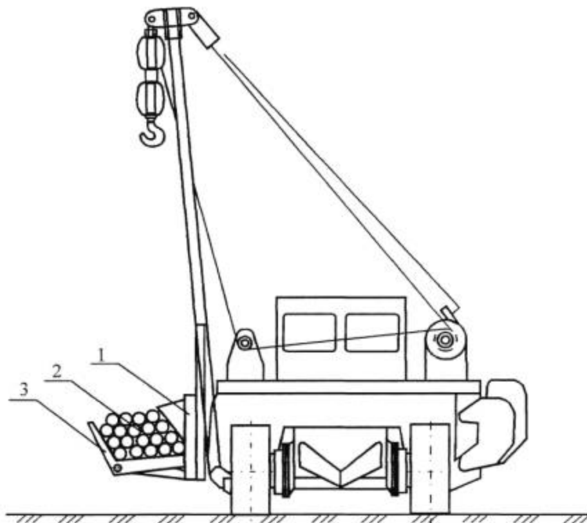
Рис. 11.1. Трубоукладчик с боковыми опорами
