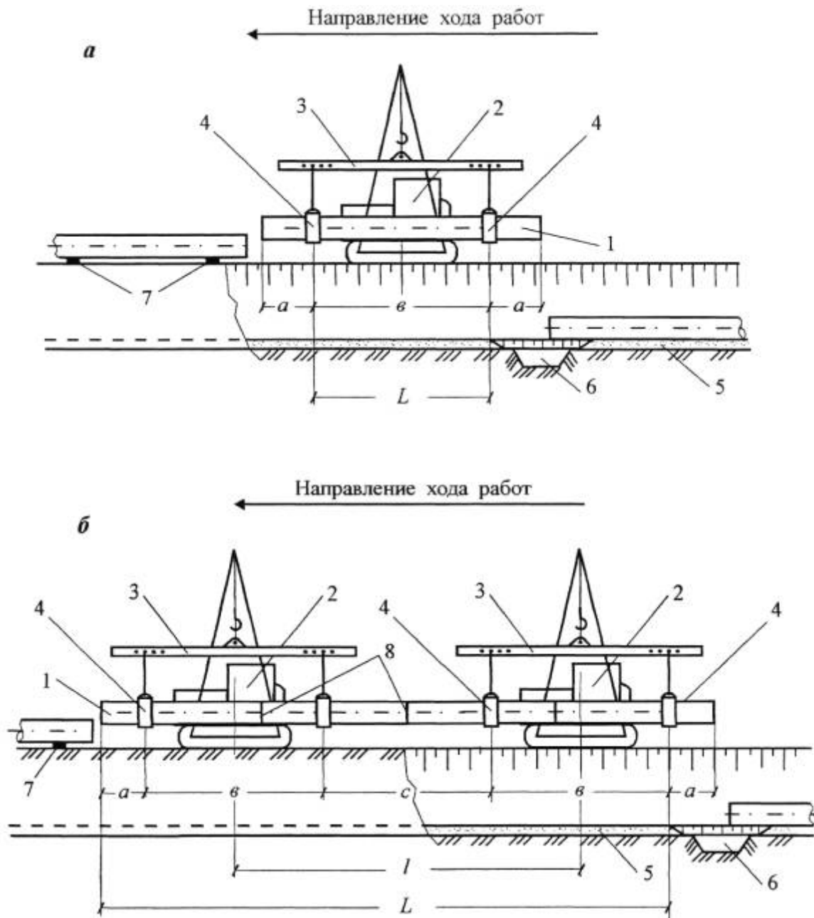
Рис. 14.1. Технологическая схема опускания одиночных труб и секций при строительстве трубопроводов из стеклопластиковых труб
