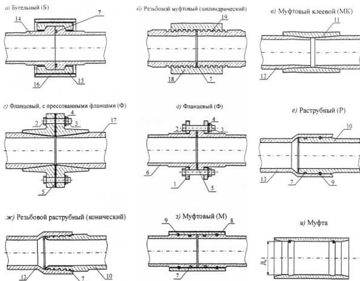
Рис. 5.1. Конструкции соединений стеклопластиковых труб
