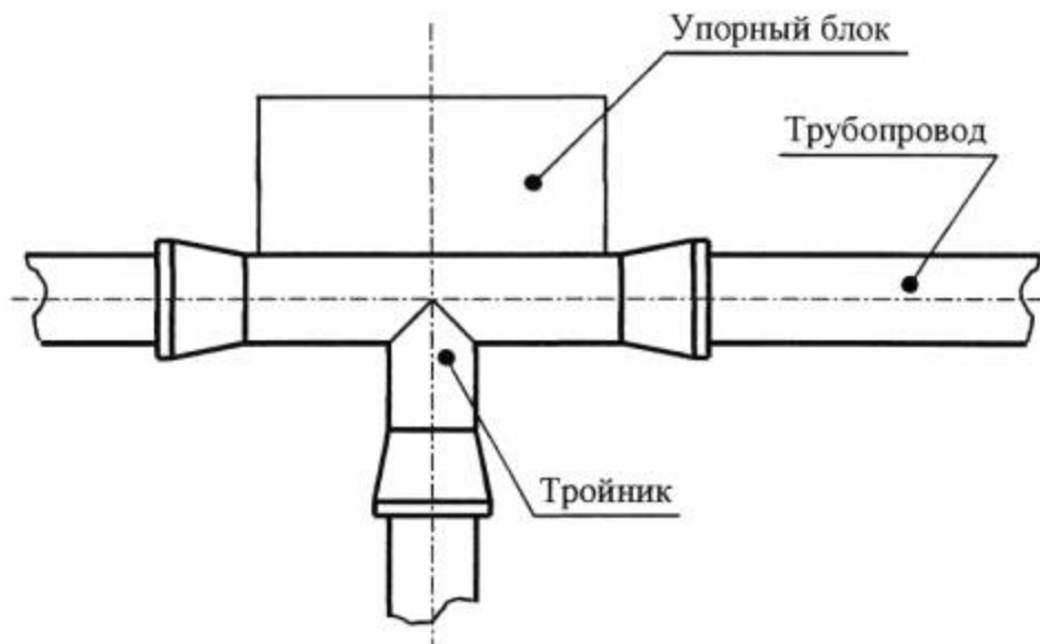
Рис. 7.2. б. Упорный блок тройника
