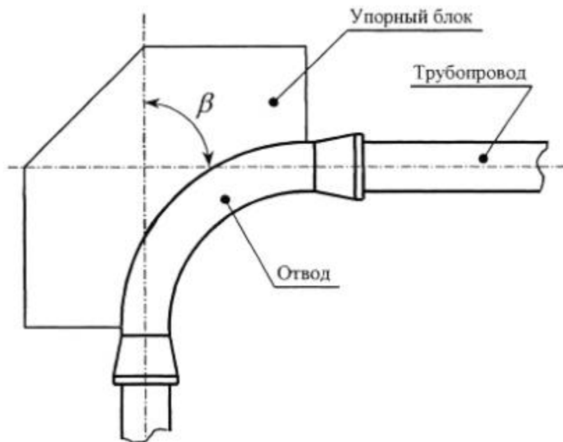
Рис. 7.2. а. Упорный блок отвода
