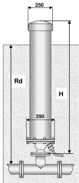
Надземная установка
