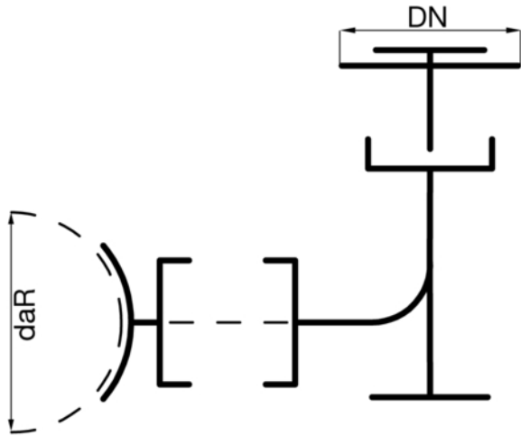
Боковое соединение
