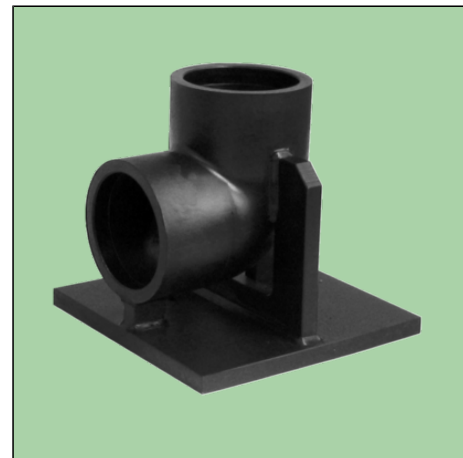
ELGEF® Plus MMN-Колено на опоре да 90
