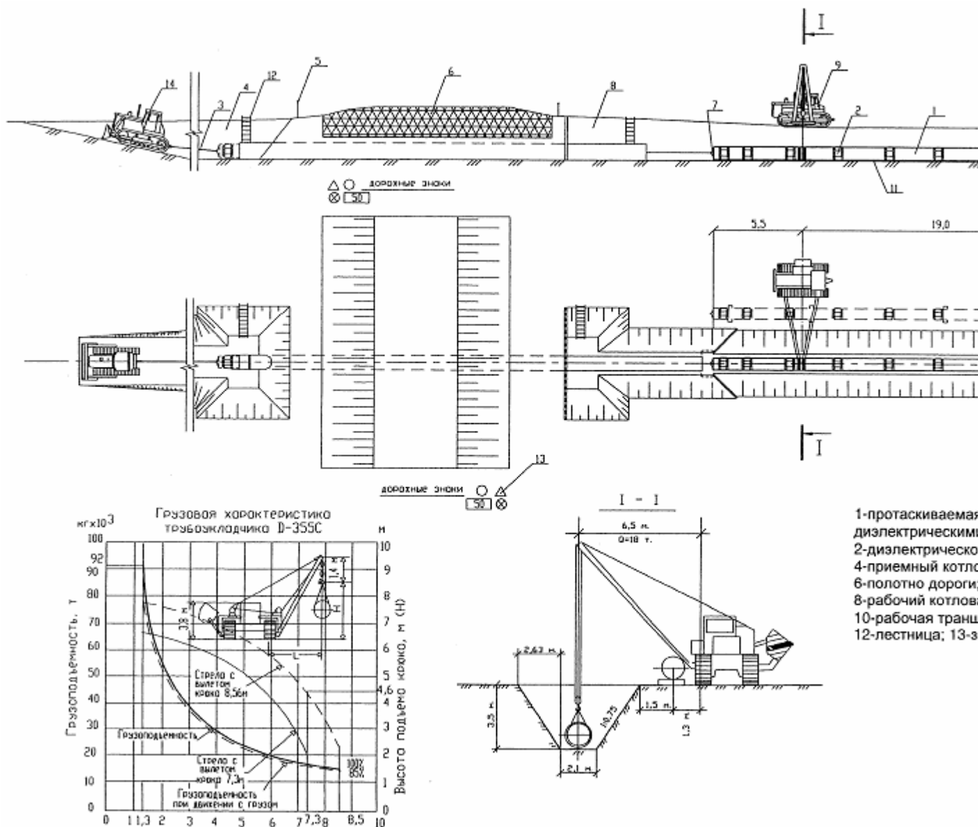
Рис. 10. Схема протаскивания рабочей плети трубопровода в защитный кожух
