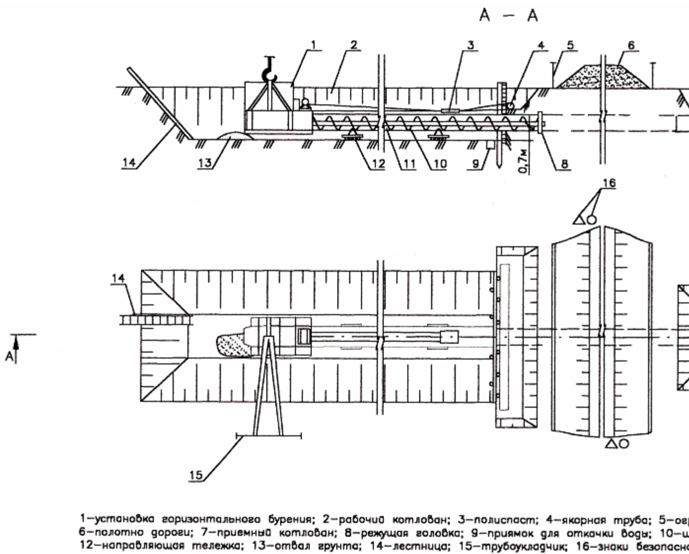
Рис.2. Схема котлованов для сооружения перехода методом горизонтального бурения
