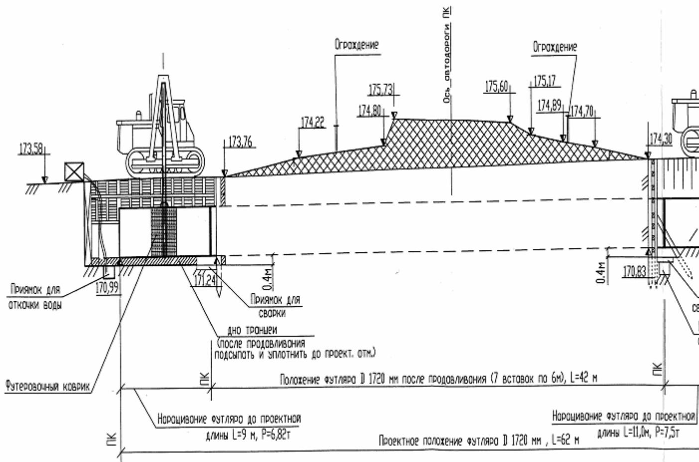
Рис.8. Нарращивание защитного кожуха (футляра)
