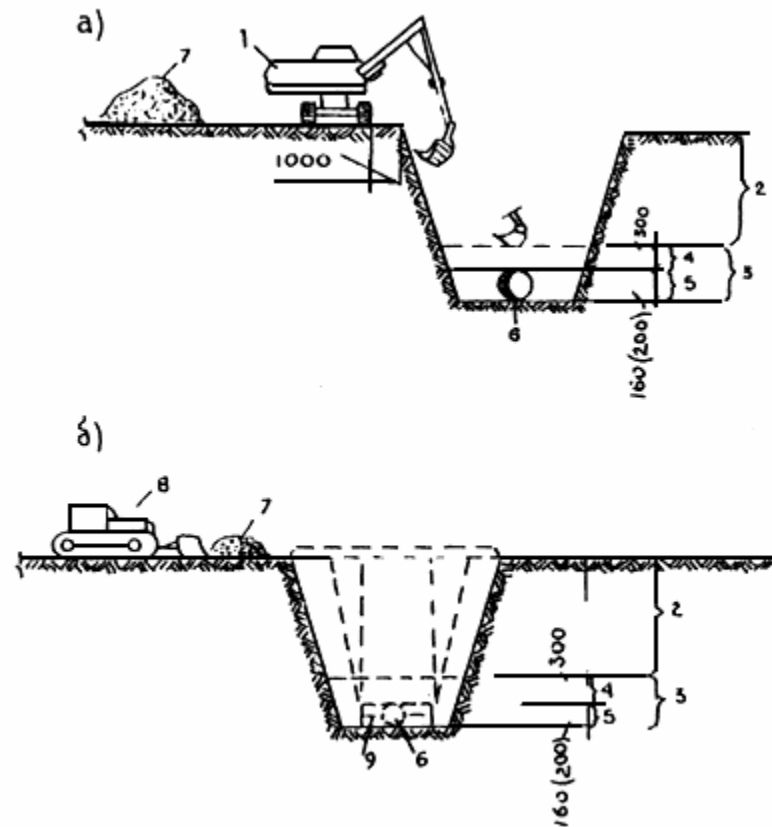
Рис.2. Схема организации работ по засыпке траншей: а) экскаватором-планировщиком; б) бульдозером;
