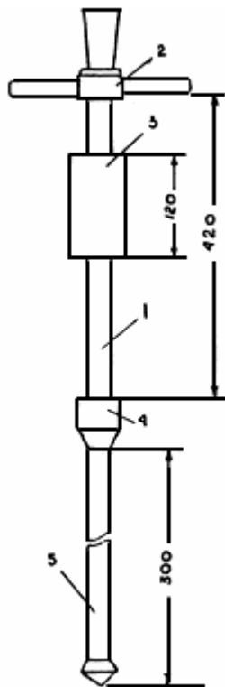
Рис.1. Прибор ДПУ для контроля плотности грунта
