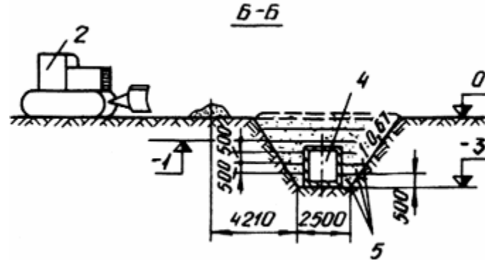
Рис.10. Схема обратной засыпки и разравнивания грунта бульдозером от отм. -1 до отм. 0
