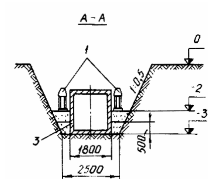
Рис.11. Схема уплотнения связного грунта II группы электротрамбовками
