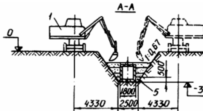
Рис.5. Схема обратной засыпки и разравнивания грунта экскаватором-планировщиком ЭО-3332А от отм. -2,5 до отм -1 1 - экскаватор-планировщик ЭО-3332А; 2 - бульдозер ДЗ-42; 3 - автомобиль-самосвал ЗИЛ-ММЗ-3555; 4 - коллектор; 5 - зона разравнивания грунта вручную
