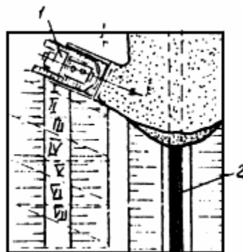
Рис.4. Обратная засыпка траншеи грунтом при помощи бульдозера:
