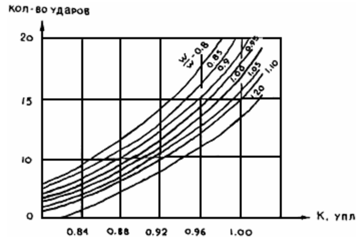
График 2. Определение коэффициента уплотнения супесей
