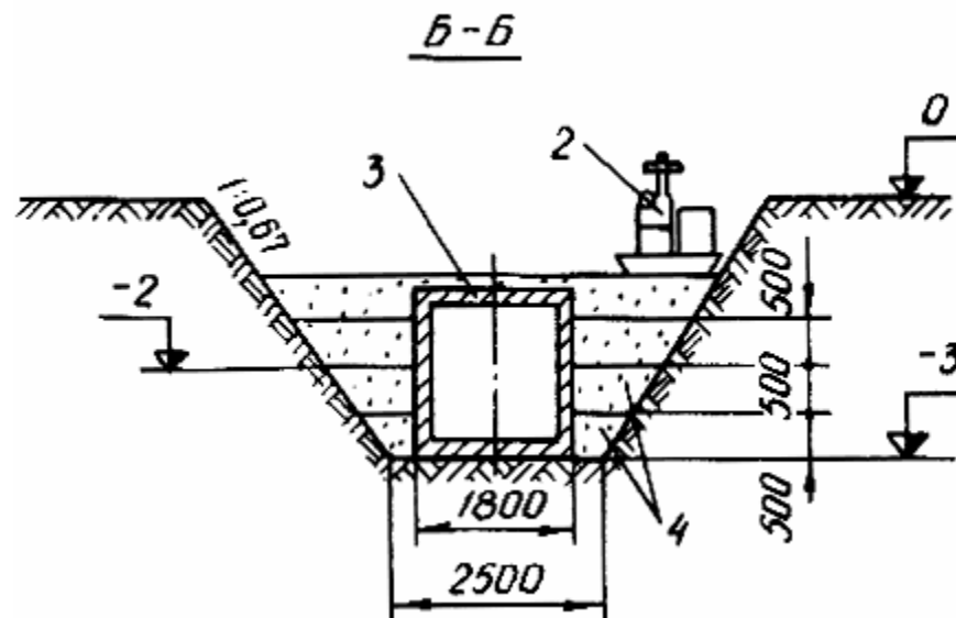
Рис.12. Схема уплотнения связного грунта I группы вибрационной плитой
