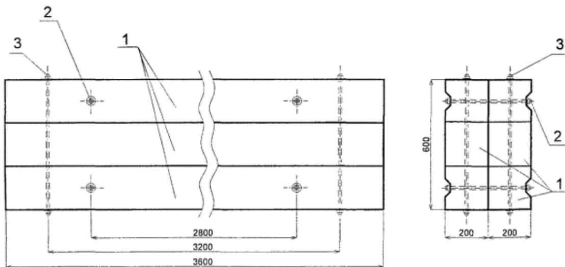
Рисунок 3 - Опорный пакет. Вариант 1. Набор из рельс
