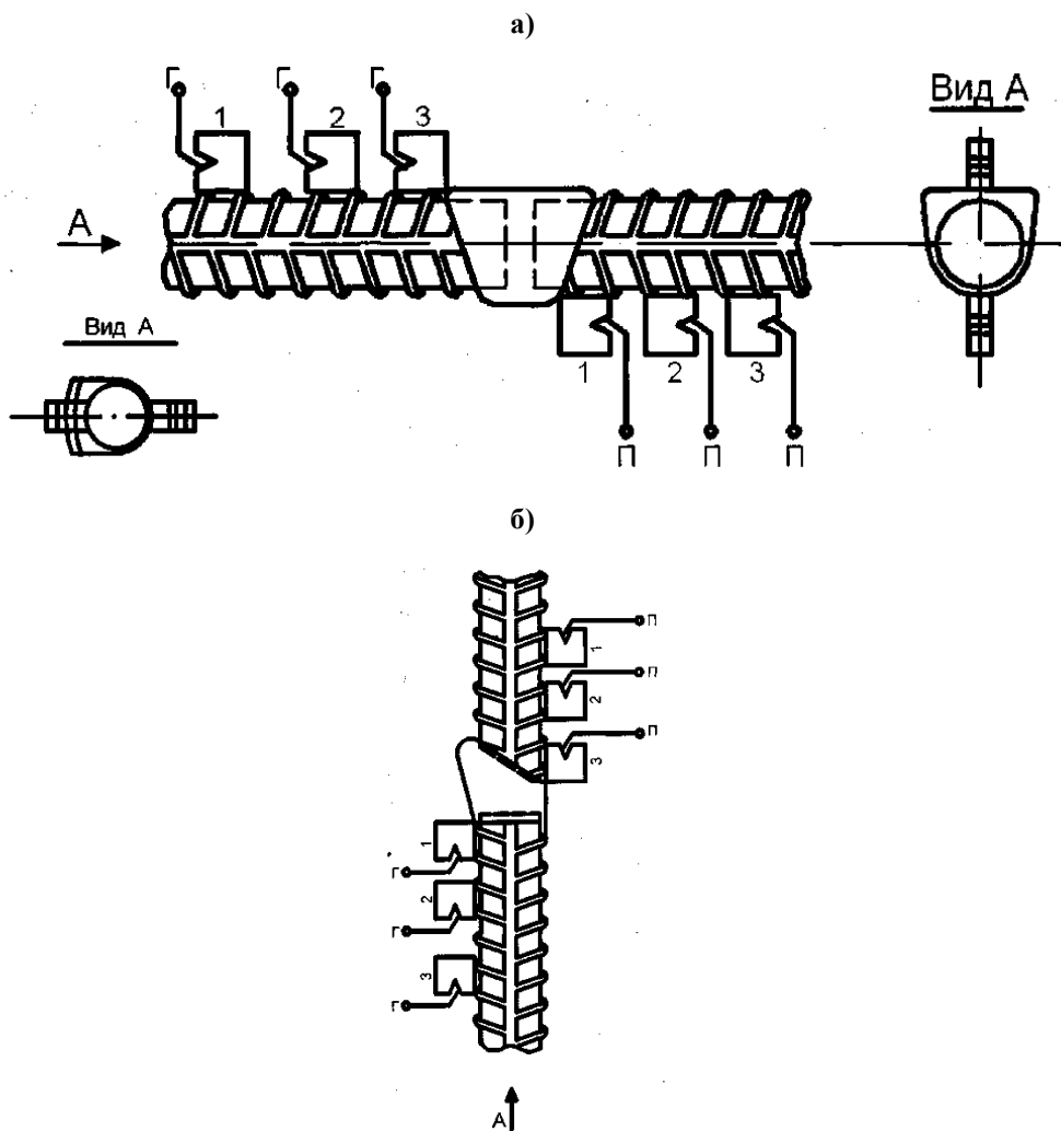
Рис. 6. Проведения контроля сварных соединений теньевым методом.
