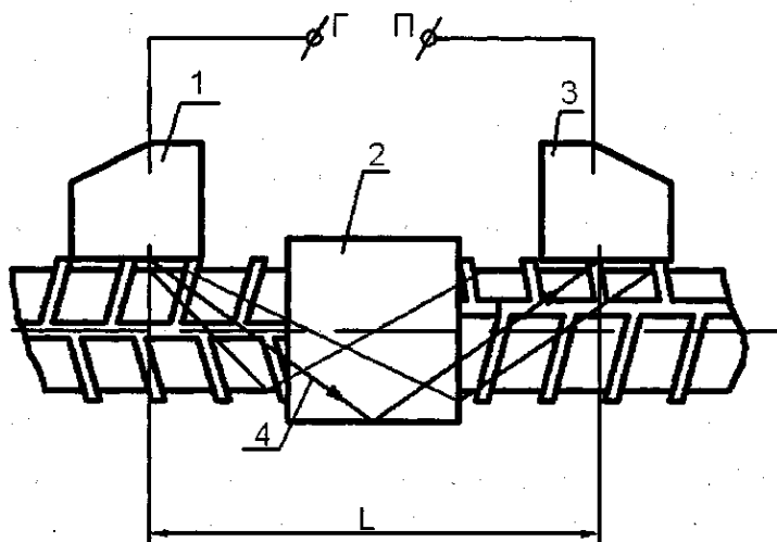
Рис. 2. Схема ультразвукового контроля сварного стыкового соединения арматурных стержней зеркально-теньевым методом.
