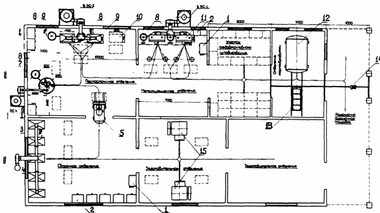
Рис.1. Примерная схема планировки и размещения оборудования цеха по изготовлению и антикоррозионной защите закладных деталей
