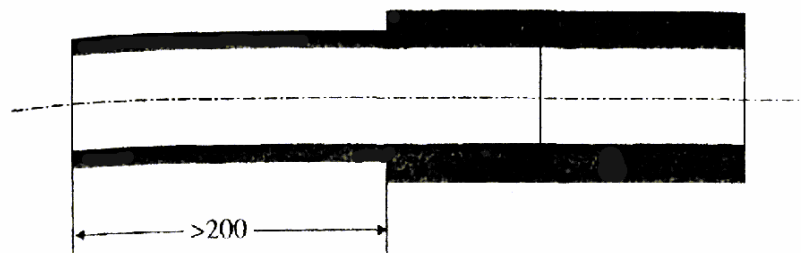
Рис. 8. Контрольное сварное соединение типа Р
