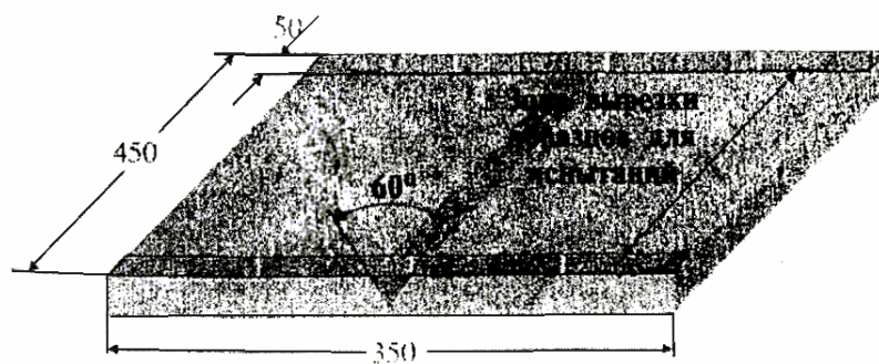
Рис. 9. Контрольные сварные соединения типов V; X
