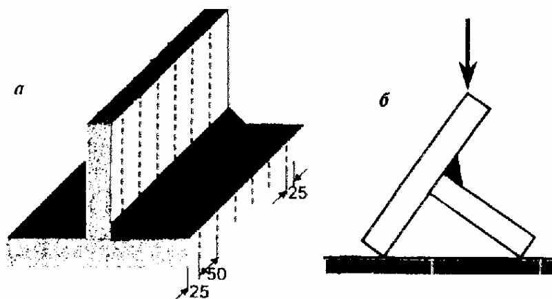
Рис. 11.2. Схема вырезки (а) и испытаний (б) на излом образцов из таврового контрольного сварного соединения листов
