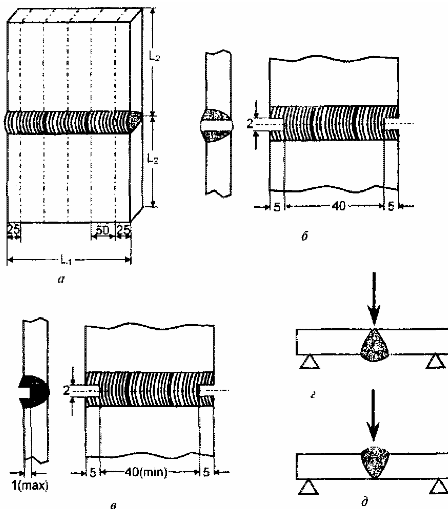
Рис. 11.1. Схемы вырезки (а), виды (б, в) и схемы испытаний на излом со стороны корня шва (з) и со стороны усиления шва (д) образцов из стыковых контрольных сварных соединений листов
