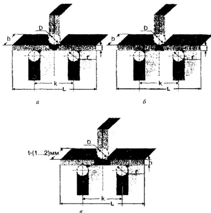
Рис. 10.1. Схемы испытаний на статический изгиб со стороны усиления шва (а), со стороны корня шва (б) и на боковой изгиб - изгиб «на ребро» (в) образцов из контрольных стыковых сварных соединений листов и труб
