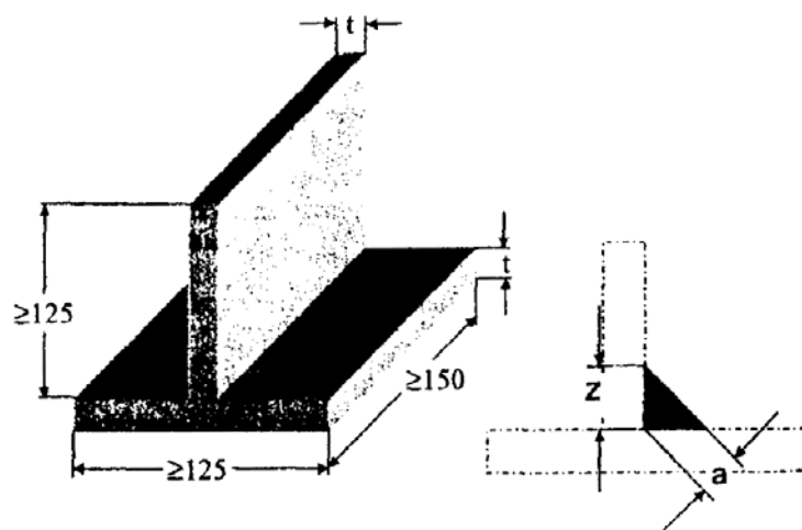
Рис. 4. Размеры деталей для тавровых контрольных сварных соединений листов
