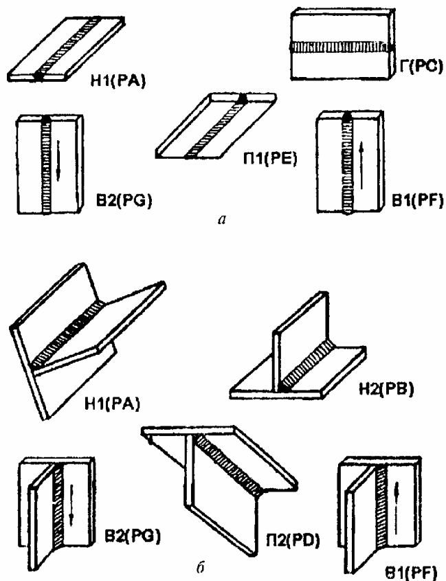
Рис. 1. Положения при сварке стыковых (а) и тавровых (б) соединений листов:
