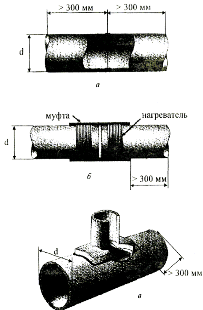
Рис. 7. Типы контрольных сварных соединений при сварке труб из полимерных материалов:
