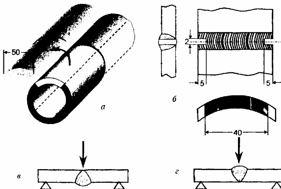
Рис. 11.3. Схемы вырезки (а), вид (б) и схемы испытаний на излом со стороны корня шва (в) и со стороны усиления шва (г) образцов из стыкового контрольного сварного соединения труб
