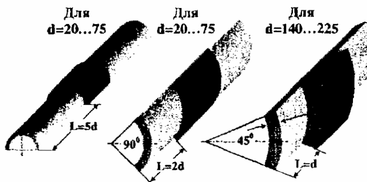
Рис. 13.1. Общий вид образцов-сегментов
