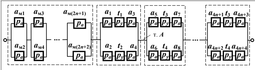
Рис. 4.24 – Расчётная модель функциональной надёжности магистральной сети с абсолютной ремонтопригодностью
