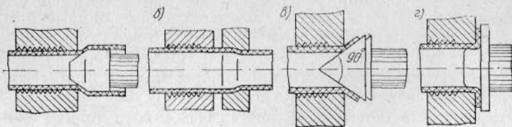
Рис. 47. Схемы выполнения раздачи а, отжима б и отбортовки в на концах труб
