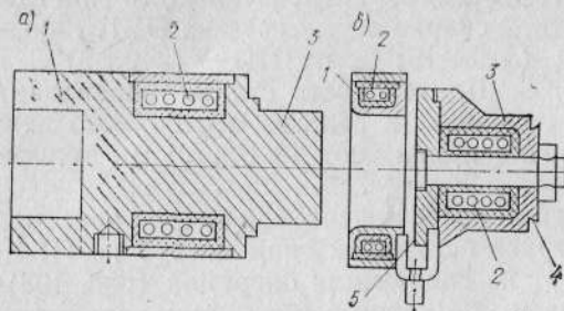
Рис. 104. Инструмент для контактной раструбной а и раструбно-стыковой б сварки 1 — гильза; 2 — электродспираль; 3 — донышко; 4 — поверхность для оплавления внутренней полки раструбного конца трубы; 5 — поверхность для оплавления торца гладкого конца трубы
