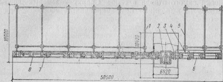
Рис. 62. Схема стационарной установки РУСТ-630 для сборки и сварки секций трубопроводов с D_y=80...600 мм
