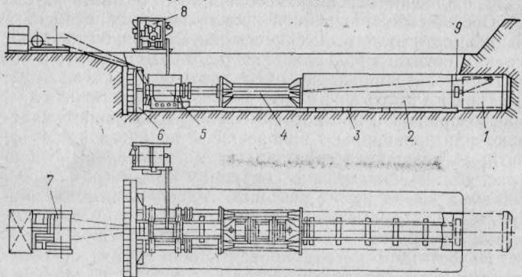
Рис. 88. Схема установки У-12,60 для бестрашшейной прокладки труб 1 — головка; 2 — патрон; 3 — направляющая патрона; 4 — вставка; 5 — гидро- домкрат; 6 — башмак; 7 — лебедка; 8 — привод гидравлический; 9 — челнок
