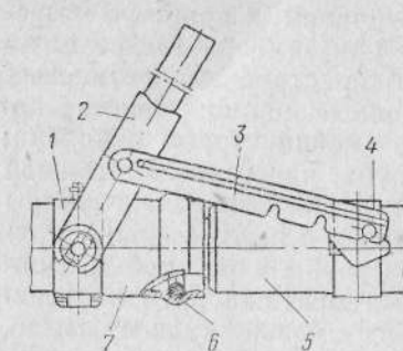
Рис. 106. Стыковочное устройство для монтажа труб внахлест на резиновых кольцах 1 — опорное кольцо; 2 — рычаг с захватом; 3 — захват; 4 — прижимное кольцо; 5 — гладкий конец трубы; 6 — резиновое кольцо; 7 — раструбный конец трубы
