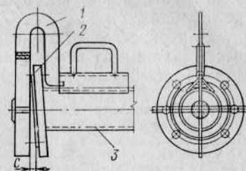
Рис. 57. Контрольный угольник
