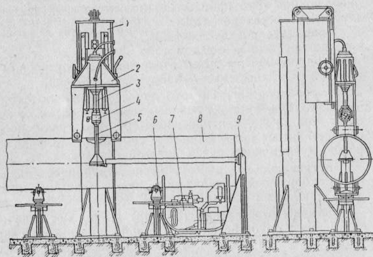
Рис. 49. Установка для вытяжки ответвлений в трубах 1 — станина; 2 — ползун; 3 — гидроцилиндр; 4 — быстроразъемный патрон; 5 — шток с пуансоном; 6 — стойка; 7 — гидростанция; 8 — труба; 9 — опора
