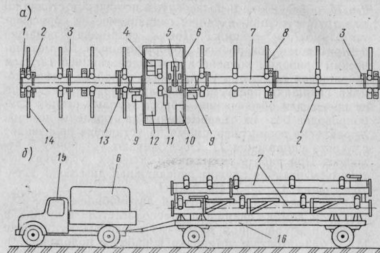
Рис. 63. Схема передвижной установки для сборки и сварки секций трубопроводов с D_y=80...600 мм в рабочем а) и транспортном б) положении
