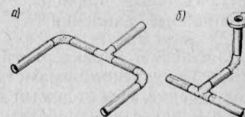
Рис. 2. Узел трубопровода а — плоский; б — пространственный
