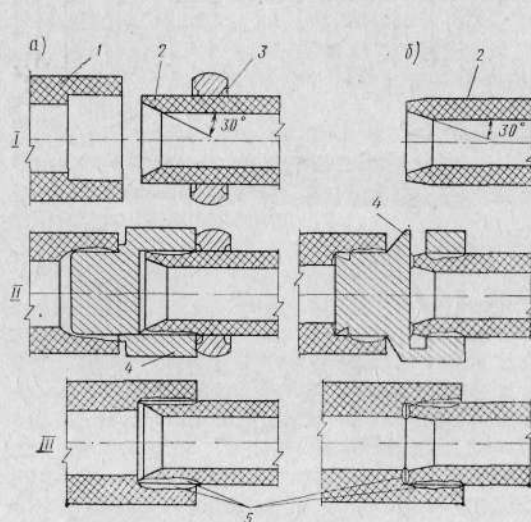
Рис. 103. Схема процесса контактной раструбной а и раструбно-стыковой б сварки труб и деталей I — подготовка, сборка и установка ограничительного хомута; II — оплавление свариваемых поверхностей; III — соединение и охлаждение сварного соединения; 1 — раструбный конец трубы; 2 — гладкий конец трубы; 3 — ограничительный хомут; 4 — нагревательный инструмент; 5 — сварной шов
