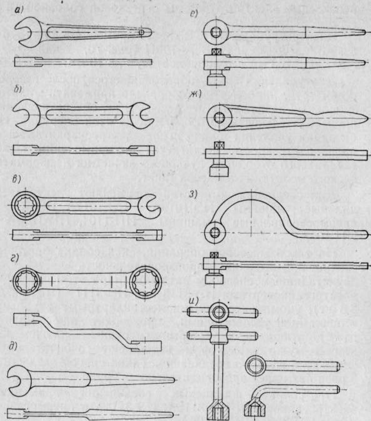
Рис. 71. Ручные гаечные ключи а — односторонний с открытым зевом; б — двусторонний с открытым зевом; в — комбинированный; г — кольцевой коленчатый; д — односторонний коленчатый; е — трещоточный коленчатый монтажный; ж — трещоточный алюминиевый монтажный; з — радиусный ключ-трещотка; и — торцовый
