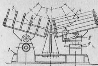
Рис. 56. Стенд для сборки секционных отводов с D_y = 300...1200 мм
