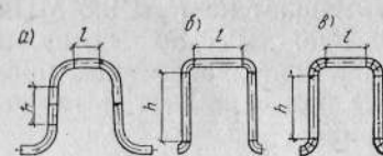
Рис. 22. П-образные компенсаторы. а — гнутые; б — с крутоизогнутыми отводами; в — со сварными отводами
