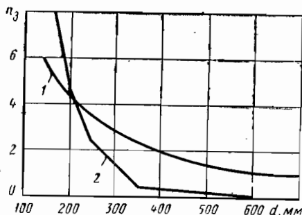
Рис. 6. Зависимость числа засорений n_з на 1 км в год от диаметра трубопровода d 1, 2 — статистические данные, относящиеся к разным районам города и периодам времени
