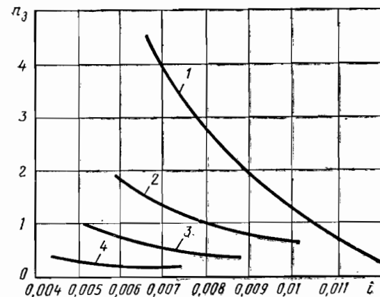
Рис. 7. Зависимость количества засорений n_з на 1 км в год от уклона i и диаметра трубопровода d (по данным НИИ КВОВ АКХ) 1 — d=150 мм; 2 — d=200 мм; 3 — d=250 мм; 4 — d=300 мм
