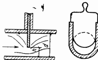
Рис. 19. Схема задвижки
