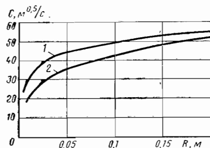
Рис. 4. Зависимости коэффициента C от гидравлического радиуса 1 — по формуле (16); 2 — по формулам (5) и (9)
