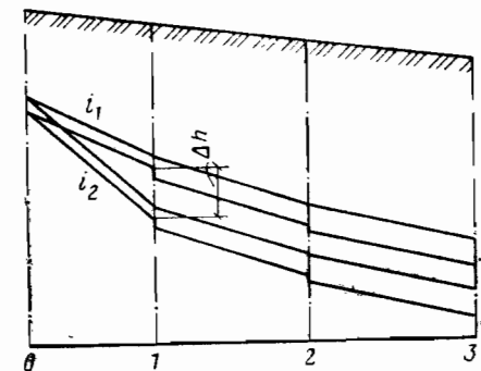
Рис. 13. Продольный профиль трубопровода
