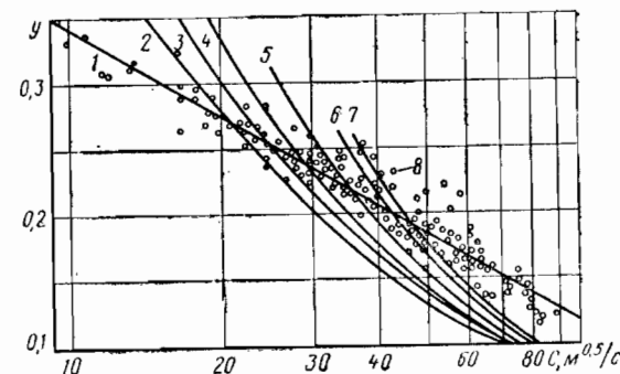
Рис. 3. Зависимости показателя степени y от коэффициента C
