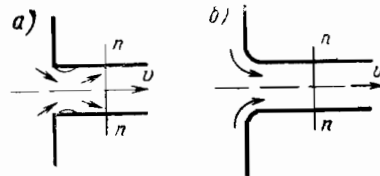
Рис. 16. Схема установки диафрагмы а — при изменении диаметра трубопровода; б — на трубопроводе постоянного диаметра
