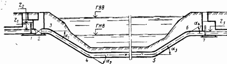
Рис. 21. Схема дюкера через реку
