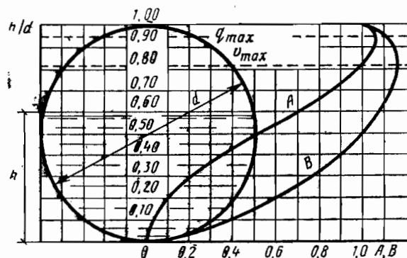
Рис. 12. Зависимость параметров A и B от степени наполнения трубопровода
