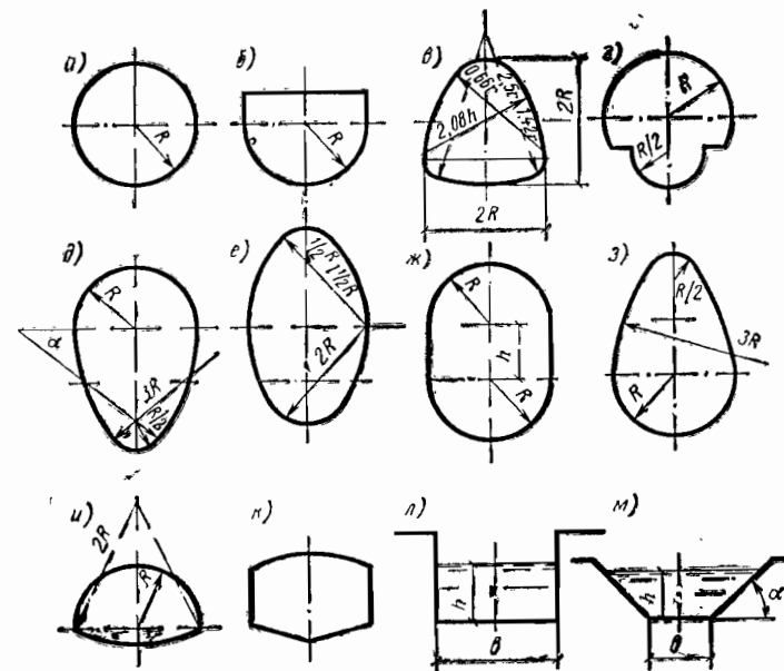
Рис. 5. Формы поперечного сечения труб
