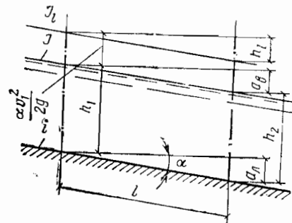
Рис. 1. Схема безнапорного потока
