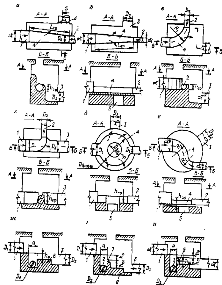
Рис. 7.1. Схема различных конструкций разделительных камер: а – с односторонним прямолинейным боковым водосливом; б – то же с двусторонним; в – то же с криволинейным и одним поворотом; г – с полигональным торцевым водосливом; д – с кольцевым водосливом; е – криволинейный боковой водослив с двумя поворотами; ж – донный слив; з – с разделительной стенкой; и – то же с отверстием в ней; 1 и 2 – подводящий и отводящий коллекторы; 3 – сбрасывающий коллектор; 4 – лоток; 5 – отверстия; 6 – нижний бьеф; 7 – разделительная стенка
