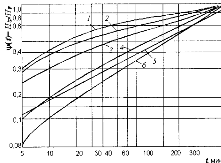
Рис. 2.10. Средние кривые редукции осадков для некоторых районов России при p_{об} \leq 25\% : 1 – возвышенности ЕТС, запад Урала; 2 – север ЕТС и Западной Сибири; 3 – побережье Белого моря; 4 – побережье Охотского моря; 5 – побережье Татарского пролива; 6 – восточное побережье Камчатки
