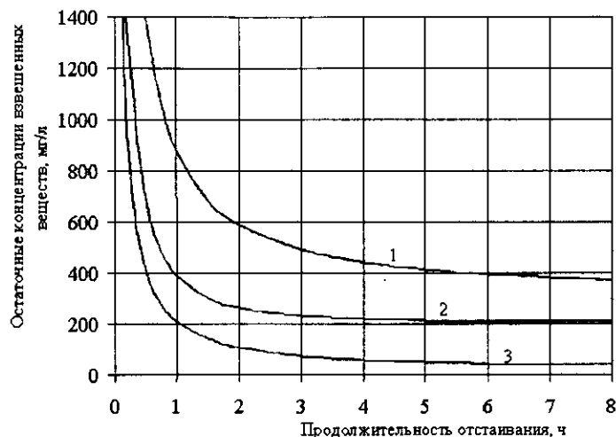
Рис. 9.12. Кинетика отстаивания поверхностного стока промышленных предприятий: 1 – дождевой сток нефтехимических предприятий; 2 – то же машиностроительного завода; 3 – талого стока нефтехимических предприятий
