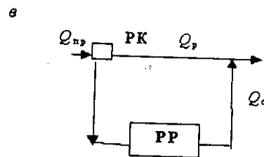
Рис. 7.6. Схемы подключения регулирующих резервуаров (РР) к дождевой сети: а – проточные с поступлением всего расхода к резервуару; б – с разделительной камерой (РК) и с насосной станцией (НС) для опорожнения; в – с самотечным трубопроводом для опорожнения
