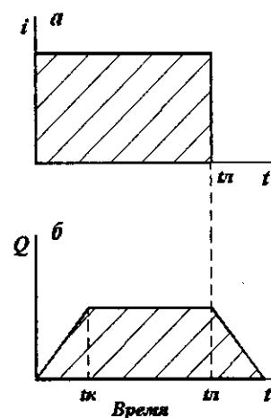
Рис. 2.2. Ход осадков ( i ) и стока ( Q ) во времени: а — гистограмма; б — гидрограф
