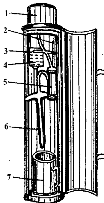
Рис. 1.2. Плувиограф типа П-2: 1 — приемный сосуд; 2 — шток; 3 — перо; 4 — барабан с бумажной лентой; 5 — измерительный цилиндр; 6 — сифонная трубка; 7 — сосуд, в который переливается вода из измерительного цилиндра
