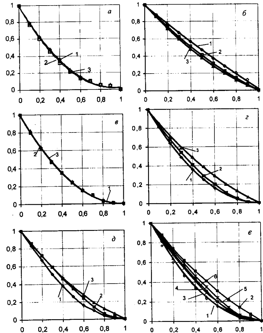
Рис. 7.9. Зависимость коэффициента регулирования \alpha от коэффициента объема емкости \beta для различных типов дождей: а – первого; б – второго; в – третьего; г – четвертого; д – пятого; е – для пяти дождей разных типов при t_k/T = 0,4 (кривые 1–5) и для обобщенного гидрографа (кривая 6); для зависимостей а–д: 1 – при t_k/T = 0,2 ; 2 – при t_k/T = 0,4 ; 3 – при t_k/T = 0,5
