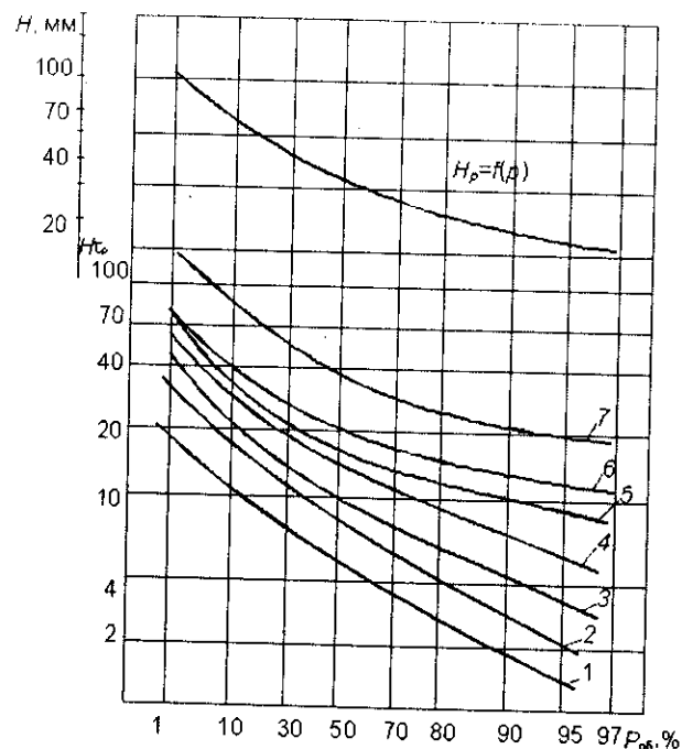
Рис. 2.8. Эмпирические кривые обеспеченности наибольших в году осадков H_p = f(p_{06}) и слоев осадков H_\tau = f_\tau(p_{06}) за интервалы времени 5(1), 10(2), 20(3), 60(4), 150(5), 300(6) и 2880(7) мин в те же годы наблюдений
