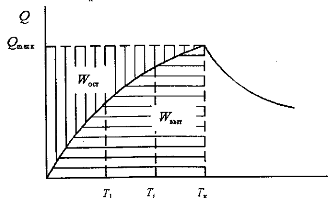
Рис. 4.5. Расчетная схема к определению свободной емкости коллектора
