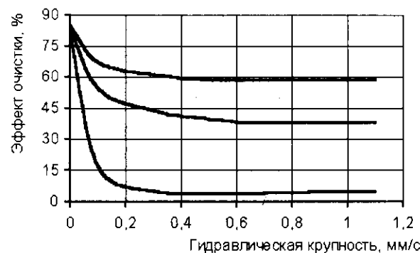
Рис. 9.10. Обобщенные данные кинетики осаждения взвешенных веществ дождевого стока с городских территорий Харькова
