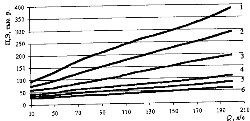
Рис. 9.17. Приведенные и эксплуатационные затраты сооружений по очистке дождевых вод: 1, 2, 3 – приведенные затраты для 3, 2, 1-й ступеней фильтрации соответственно, тыс. р.; 4, 5, 6 – эксплуатационные затраты для 3, 2, 1-й ступеней фильтрации соответственно, тыс. р.
