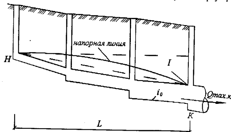
Рис. 4.4. Напорная схема работы коллектора при его заполнении
