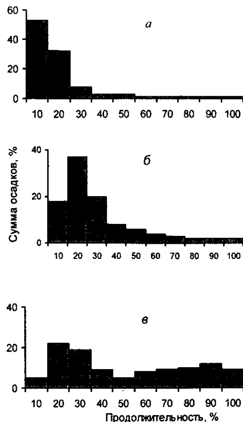
Рис. 2.16. Гистограмма для ливней I типа: 10%-ной (а), 50%-ной (б) и 90%-ной (в) вероятности
