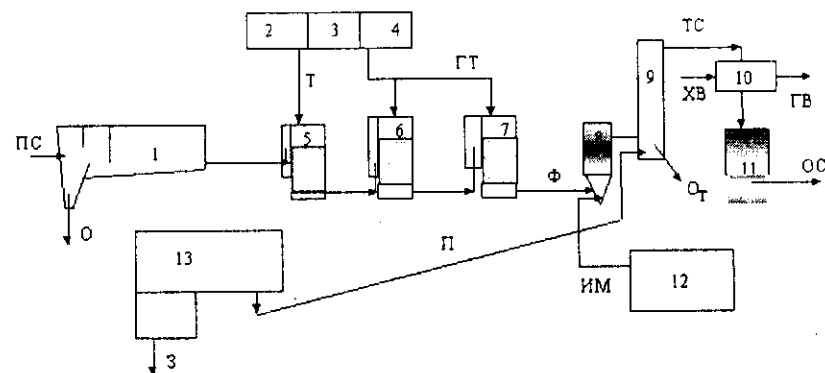
Рис. 10.2. Технологическая схема очистки поверхностного стока предприятий медеплавильной промышленности:
