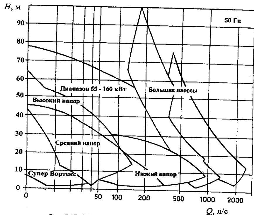
Рис. 7.17. Область применения насосов "Сарлин"
