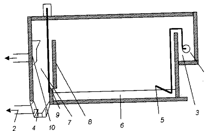
Рис. 7.11. Конструкция регулирующего резервуара: 1 – подающий трубопровод; 2 – трубопровод опорожнения; 3 – галерея задвижек; 4 – прямик трубопровода опорожнения; 5 – насадки; 6 – лотки опорожнения; 7 – канал опорожнения; 8 – поперечная перегородка; 9 – шиберы; 10 – аварийный сброс
