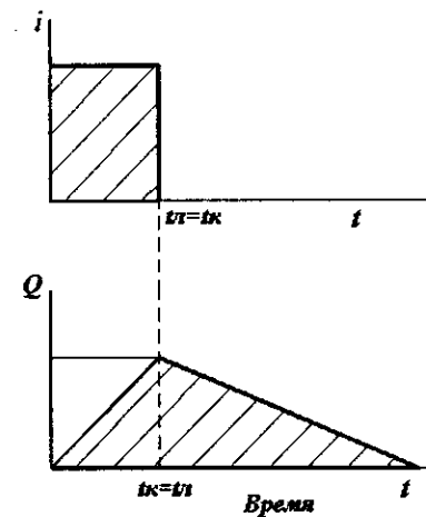
Рис. 2.3. Осадки ( i ) и сток ( Q ) при t_k = t_L
