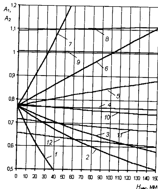
Рис. 2.13. Изменение параметров A_1 (кривые 1-7 соответственно при i_n = 0,005; 0,01; 0,03; 0,05; 0,1 и 0,5 \% ); A_2 (кривые 8-12 соответственно при i_{\text{ос}} = 0,42 или q = 70; 0,36 или 60; 0,18 или 30; 0,12 или 20; 0,06 мм/мин или 10 л/с · га)
