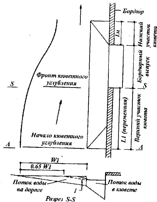
Рис. 6.5. Поток воды на участке дороги перед бордюрным впуском с кюветом (гидравлический уклон равен поперечному уклону)
