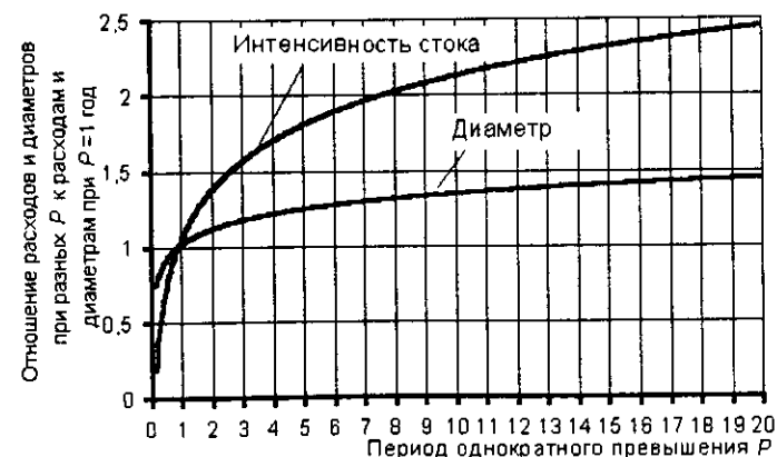
Рис. 8.4. Зависимость относительной интенсивности выпадения дождя и диаметров труб от периода однократного превышения P
