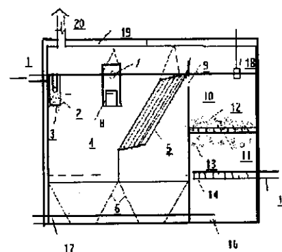
Рис. 9.8. Установка очистки сточных вод: 1 – подвод сточных вод; 2 – пескоулавливающий бункер; 3 – полупогружная перегородка; 4 – отстойная зона; 5 – тонкослойный блок; 6 – приямок для осадка; 7 – поворотная труба; 8 – емкость для нефтепродуктов; 9 – водослив; 10 – фильтр с плавающей загрузкой; 11 – решетка; 12 – щебень; 13 – плавающая загрузка; 14 – дренаж большого сопротивления; 15 – отвод очищенных сточных вод; 16 – дренаж малого сопротивления; 17 – отвод промывных вод; 18 – поплавковый указатель уровня; 19 – утепленная крышка; 20 – вентиляционный патрубок
