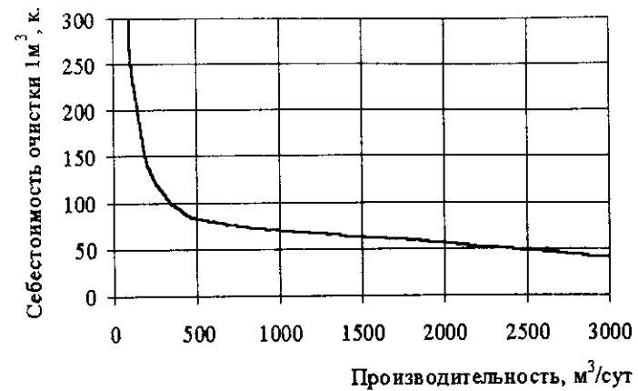
Рис. 9.14. Зависимость себестоимости очистки поверхностного стока от суточной производительности очистных сооружений
