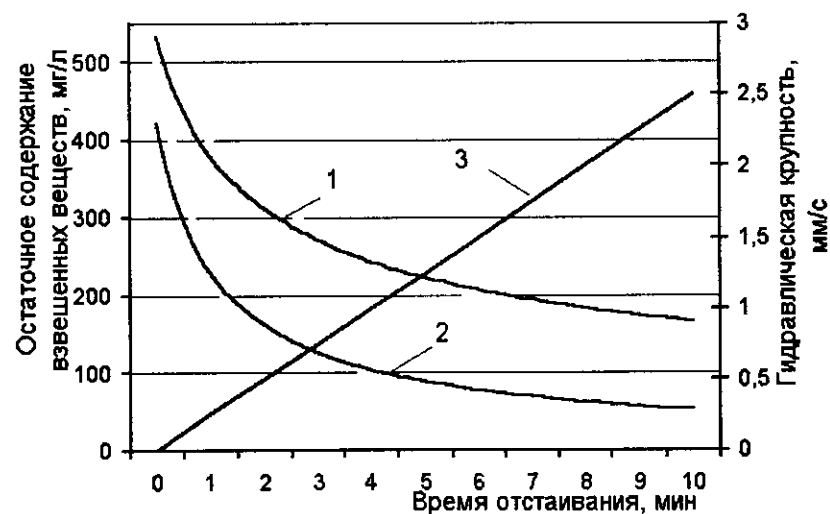
Рис. 9.9. Зависимость остаточного содержания взвешенных веществ и гидравлической крупности от времени отстаивания при реагентной обработке поверхностных сточных вод: 1 – зависимость остаточной концентрации взвешенных веществ от времени отстаивания при обработке воды Al_2(SO_4)_3 , дозой 30 мг/л; 2 – зависимость остаточной концентрации взвешенных веществ при обработке воды Al_2(SO_4)_3 (20 мг/л) и ПАА (1 мг/л), 3 – зависимость гидравлической крупности (охватывающей скорости) от времени отстаивания
