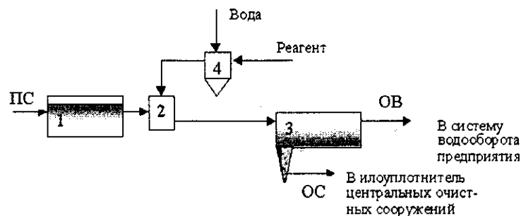
Рис. 10.1. Технологическая схема отведения и очистки поверхностного стока предприятий цветной металлургии: 1 - усреднитель; 2 - смеситель; 3 - отстойник; 4 - реагентное хозяйство; ПС - поверхностный сток; ОВ - осветленные воды; ОС - осадок
