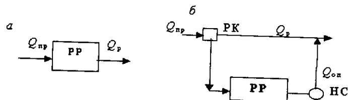
Рис. 7.6. Схемы подключения регулирующих резервуаров (РР) к дождевой сети: а – проточные с поступлением всего расхода к резервуару; б – с разделительной камерой (РК) и с насосной станцией (НС) для опорожнения; в – с самотечным трубопроводом для опорожнения
