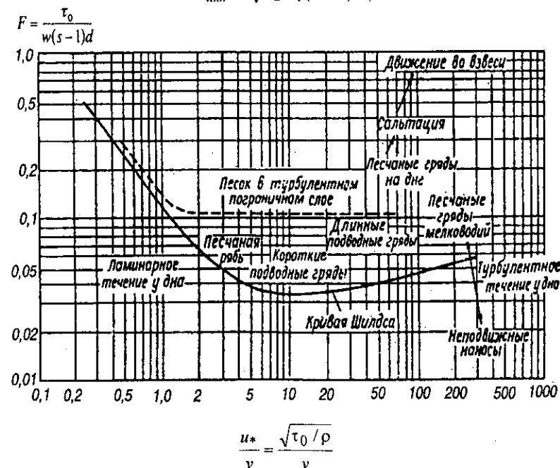
Рис. 4.7. Диаграмма для оценки характера движения несвязных частиц в потоке
