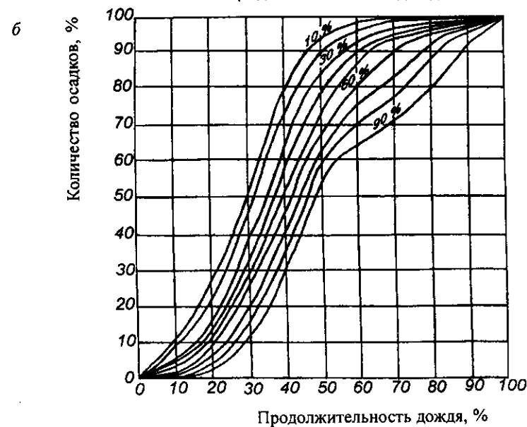
Рис. 2.15. Ход выпадения дождей различной вероятности с максимумом интенсивности в следующих четвертях их продолжительности: I (a), II (б), III (в) и IV (г)
