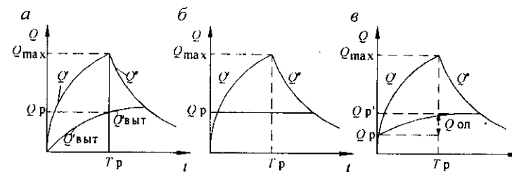
Рис. 7.8. Расчетные схемы для определения объемов регулирующих резервуаров:
