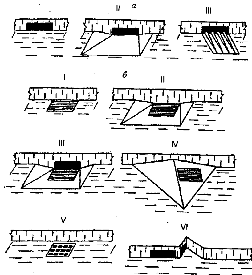
Рис. 6.4. Бордюрные (а) и кюветные (б) выпуски: I – выпуск, расположенный вровень с поверхностью дороги; II – то же, ниже поверхности дороги; III – то же, отклоняющийся или комбинированный; IV – банкетный выпуск; V – с перфорированной решеткой; VI – бордюрный выпуск с отступом
