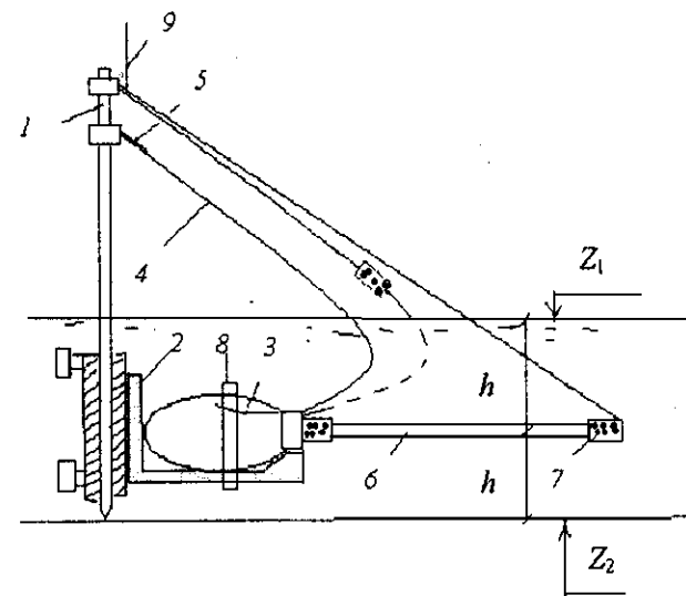
Рис. 8.1. Схема устройства пробоотборника:
