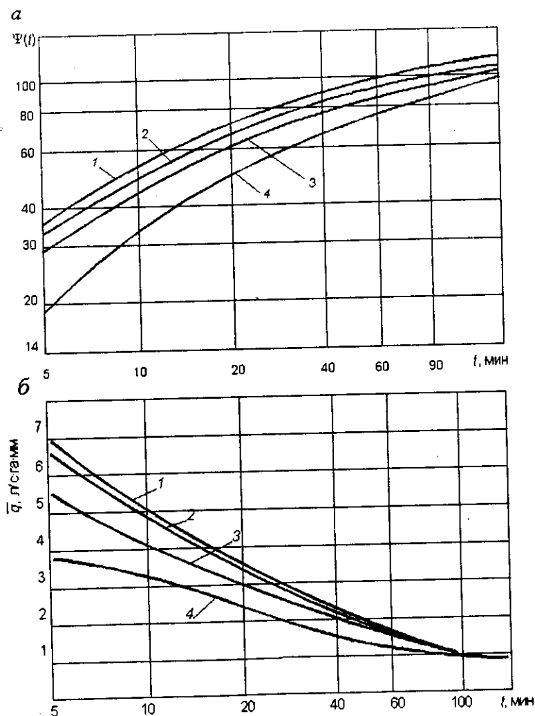
Рис. 2.11. Кривые редукции слоя \psi(t) (а) и средних интенсивностей \bar{q} = \psi(t)/t (б) осадков, выраженные в долях от равнообеспеченных суточных осадков для 10-го района (побережье Финского залива и Карельский перешеек):
