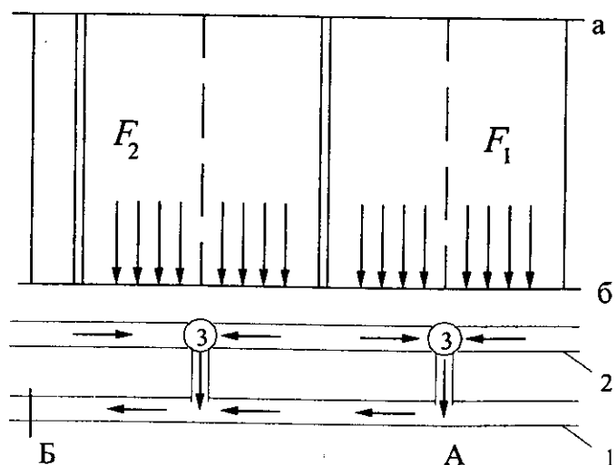
Рис. 2.4. Схема дождевого стока с площади бассейна F в коллектор: 1 — водосток; 2 — лоток; 3 — дождеприемник
