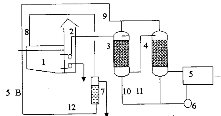
Рис. 9.6. Технологическая схема очистки поверхностных стоков:
