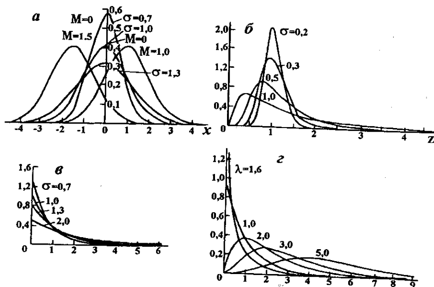
Рис. 1.5. Формы кривых различных распределений вероятностей: а – нормальное распределение с различными средними значениями M и дисперсиями \sigma ; б – логарифмически-нормальное распределение; в – показательное распределение; з – гамма-распределение ( \lambda – параметр гамма-функции)
