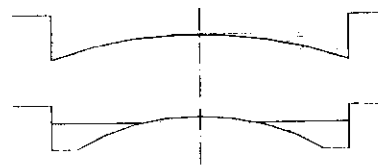
Рис. 4.2. Поперечные сечения лотков мостовых
