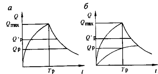
Рис. 7.10. Схемы определения объемов резервуаров при двойном регулировании:
