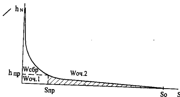
Рис. 4.12. Принципиальная схема зависимости слоя дождевого стока от количества раз его повторения в году и составляющие стока W_r = W_{оч} + W_{сбр} , направляемого на очистные сооружения и на сброс в водоемы
