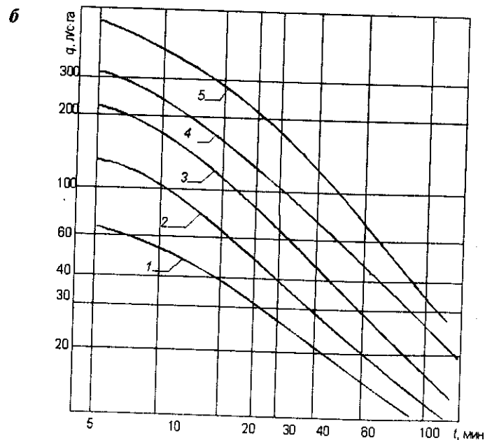
Рис. 2.7. Средние интенсивности дождя за периоды времени t по данным гидрометеослужбы для Москвы (а) и Санкт-Петербурга (б): 1-4 – соответственно при p = 0,5; 1,0; 10 и 100 лет
