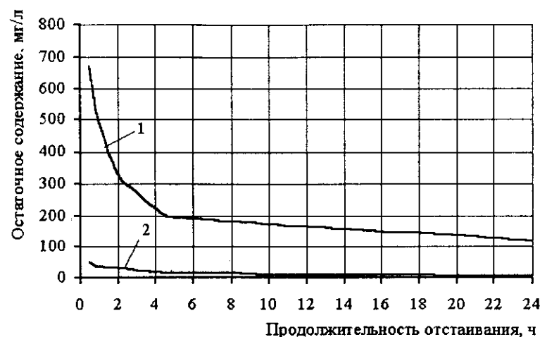
Рис. 9.11. Кинетика осаждения взвешенных веществ и удаления нефтепродуктов из городских дождевых вод Санкт-Петербурга: 1 — остаточное содержание взвешенных веществ, мг/л; 2 — то же нефтепродуктов, мг/л
