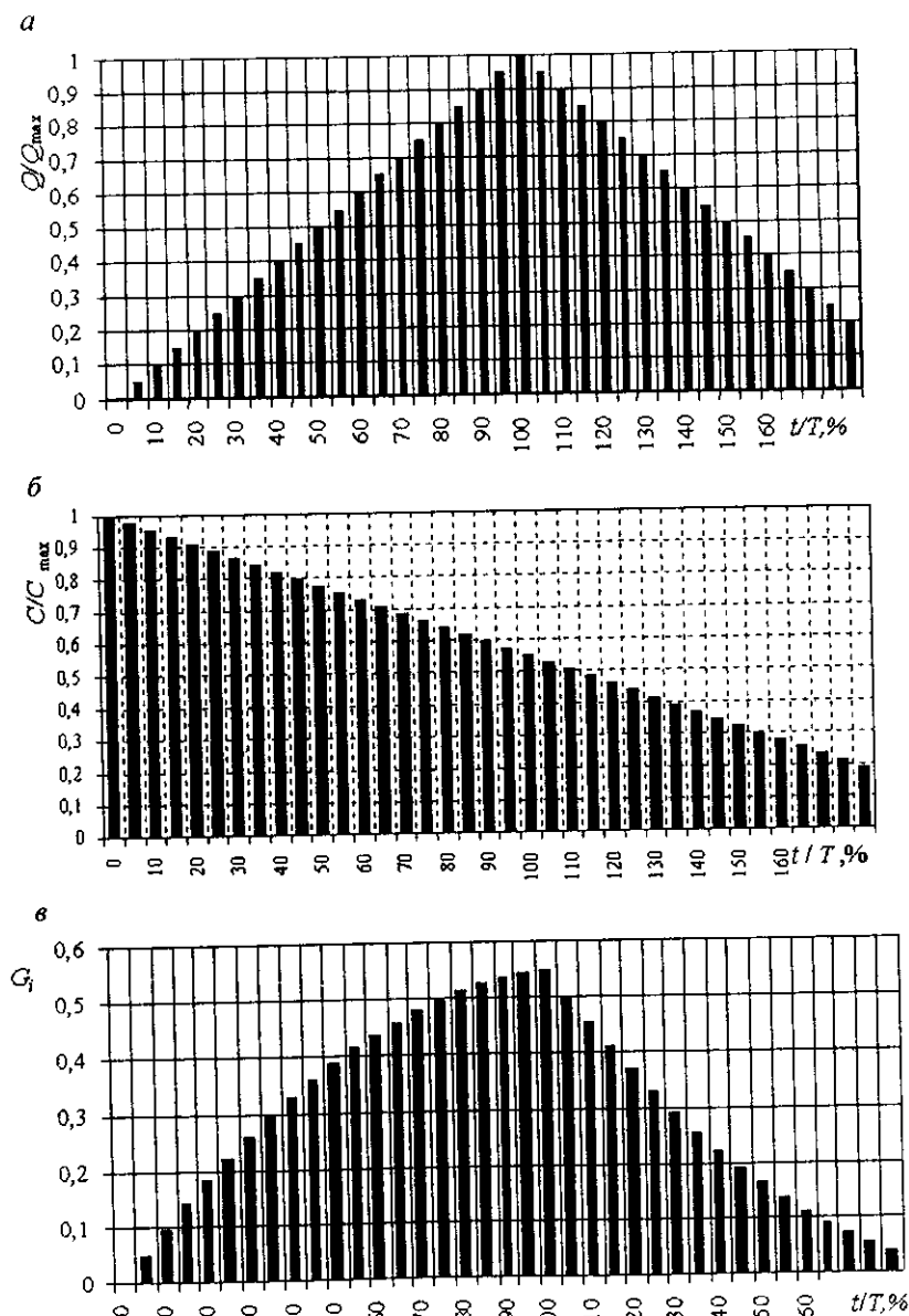
Рис. 8.2. Относительные гидрограф (а), полугидрограф (б) и количество загрязнений (в) по ходу дождя
