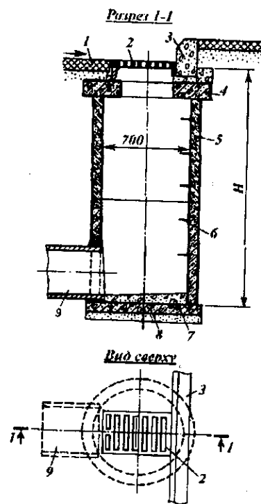
Рис. 6.2. Дождеприемник из сборных железобетонных элементов: 1 – проезжая часть, покрытая асфальтом; 2 – решетка; 3 – бордюрный камень; 4 – плита перекрытия; 5 – кольца стеновые; 6 – ходовые скобы; 7 – бетон; 8 – плита днища; 9 – соединительная труба
