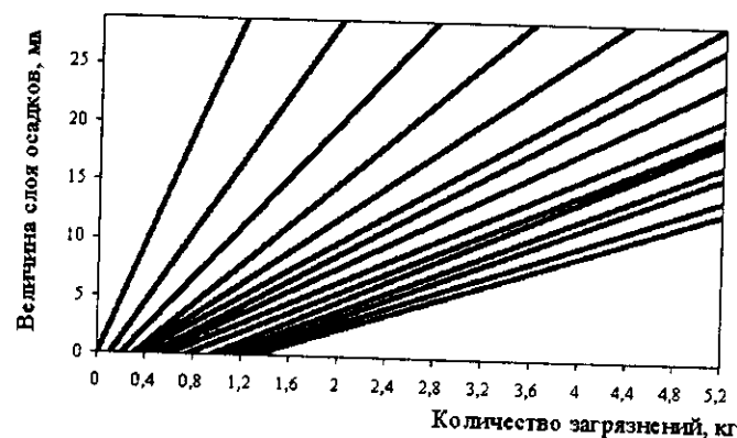
Рис. 8.3. Зависимость количества (кг) выносимых с 1 га загрязнений от слоя осадков (мм) и продолжительности периода сухой погоды (сут)
