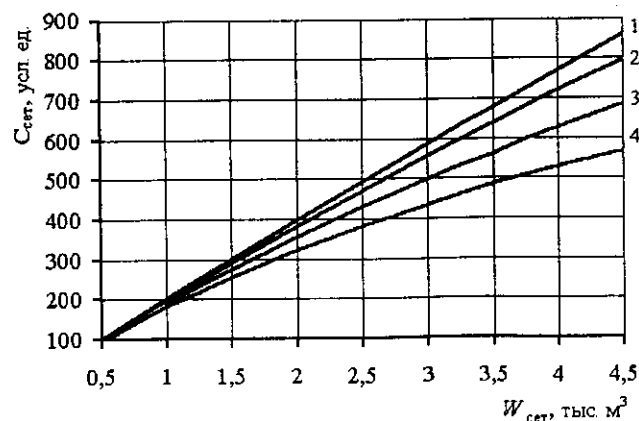
Рис. 9.16. Капитальные затраты на строительство дождевой сети в зависимости от объема коллектора и времени концентрации стока: 1 – при T_0 = 90 мин; 2 – при T_0 = 60 мин; 3 – при T_0 = 40 мин; 4 – при T_0 = 30 мин
