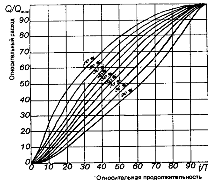
Рис. 2.17. Обобщенный график хода выпадения дождей различной вероятности
