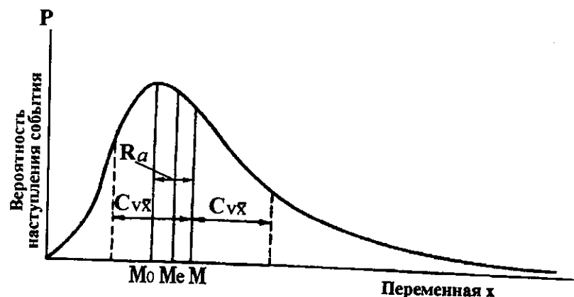
Рис. 1.7. Распределение вероятностей
