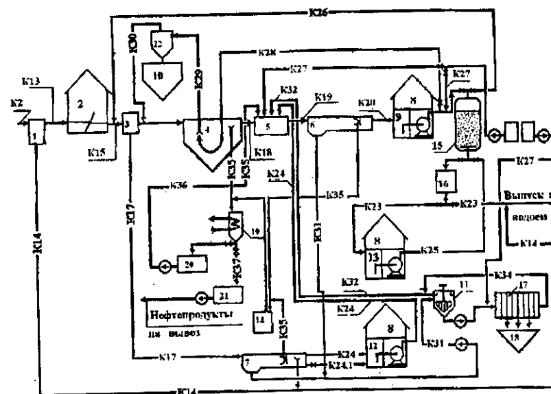
Рис. 9.1. Технологическая схема очистки дождевого стока для г. Самары: 1 – разделительная камера № 1; 2 – здание решеток; 3 – разделительная камера № 2; 4 – песколовка; 5 – смеситель; 6 – отстойник; 7 – аккумулирующий резервуар-отстойник; 8 – насосная станция; 9 – приемный резервуар осветленной воды; 10 – бункер для песка; 11 – уплотнитель осадка; 12 – приемный резервуар сточных вод из аккумулирующих резервуаров-отстойников; 13 – резервуар фильтрованной сточной воды для промывки фильтров; 14 – камера насосов перекачки плавающих веществ; 15 – напорный зернистый фильтр; 16 – установка УФ-обеззараживания; 17 – фильтр-пресс; 18 – бункер для обезвоженного осадка; 19 – разделочный бак; 20 – приемный бак подтоварной воды; 21 – бак обезвоженных нефтепродуктов; 22 – гидроциклон. Трубопроводы: K2 – городской коллектор дождевой канализации; K13 – дождевая вода, поступающая на очистные сооружения; K14 – сброс дождевой воды без очистки в водоем; K15 – сточная вода решеток; K16 – сточная вода, поступающая по дождевой сети на очистные сооружения в сухой период; K17 – сточная вода, направляемая в аккумулирующий резервуар-отстойник; K18 – сточная вода после песколовки; K19 – сточная вода после смесителя; K20 – сточная вода после отстойника; K21 – подача сточной воды на доочистку фильтрованием; K22 – фильтрованная вода; K23 – очищенная вода; K24 – подача сточной воды из аккумулирующего резервуара накопителя на промывку фильтров; K24.1 – то же при опорожнении; K25 – подача очищенной воды на промывку фильтров; K26 – загрязненная промывная вода; K27 – подача коагулянта (флокулянта); K28 – подача рабочей жидкости к гидроэлеватору песка; K29 – пескопровод; K30 – возврат воды от установки обезвоживания песка; K31 – влажный осадок; K32 – надосадочная вода; K33 – сгущенный осадок; K34 – фильтрат; K35 – обводненные нефтепродукты; K36 – подтоварная вода; K37 – нефтепродукты; K38 – аварийный перелив
