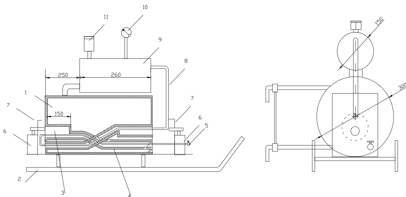
Рис. 4.6 – Аппарат для отогревания замерзших водоразборных колонок и трубопроводов:
