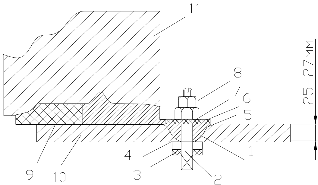
Рис. 4.3 – Заделка расточенного отверстия в чугунной трубе
