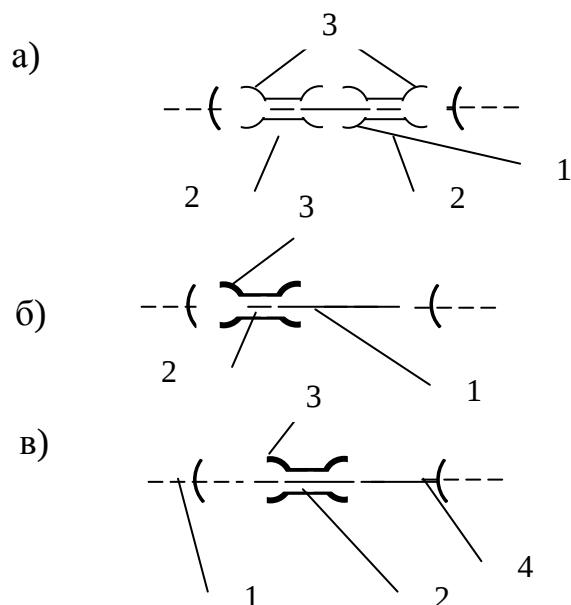
Рис. 4.4 – Ремонт треснутой или разорванной трубы:
