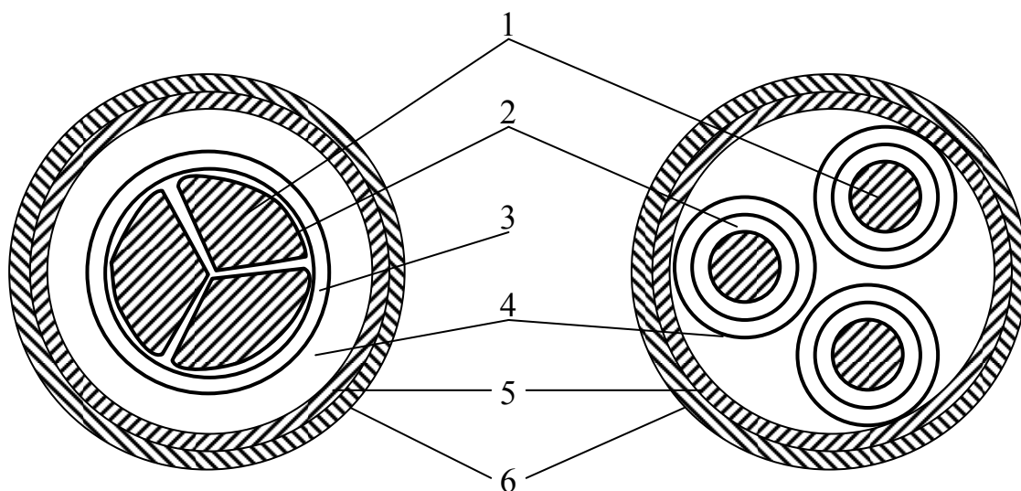
Кабель на напряжение 1...10кВ с бум.изоляцией
