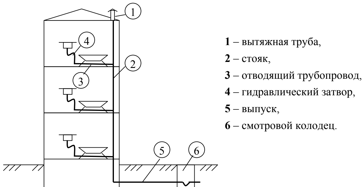
Рисунок 20 – Схема сбора и отвода стоков из здания
