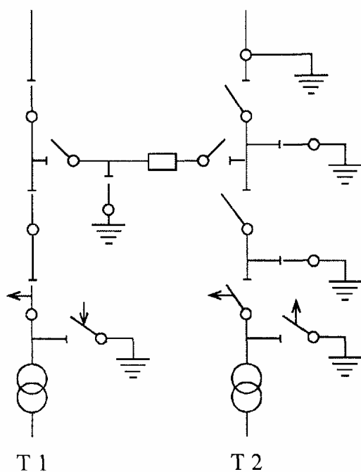
Рис. 4. Подстанция по схеме мостика. Пример установки заземлений при работе на линейном разъединителе трансформатора № 2 и на выключателе перемычки
