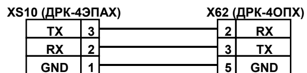
Рис. 2. Подключение ДРК-4ЭПАХ к ДРК-4ОПХ
