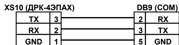
Рис. 1. Подключение ДРК-4ЭПАХ к компьютеру
