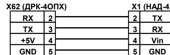
Рис. 2. Подключение НАД-4 к ДРК-4ОПХ
