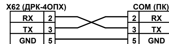
Рис. 1. Подключение ДРК-4ОПХ к компьютеру
