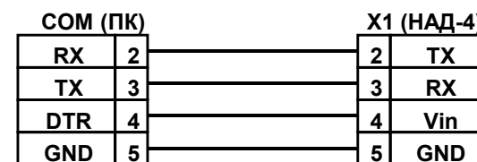
Рис. 3. Подключение НАД-4 к компьютеру
