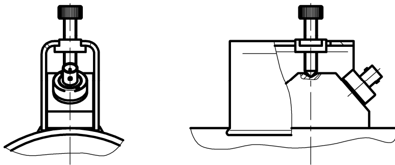
Крепление накладных ППЗ на трубопроводе (исполнение Н1)
