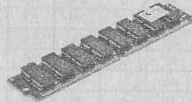
Рис. Е.2. Модуль памяти SIMM 72pin 16Mb EDO
