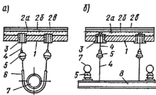
Рис. 3. Пример подвесок типа шпильки для крепления технологических трубопроводов a — одиночного; б — нескольких; 1 — железобетонная конструкция; 2 a , б , в — конструкция пола ( a — бетонное основание пола; б — химически стойкая гидроизоляция, в — покрытие пола); 3 — диэлектрическая гильза; 4 — металлическая тяга; 5 — изолятор; 6 — изоляционная прокладка; 7 — трубопровод; 8 — поддерживающая конструкция
