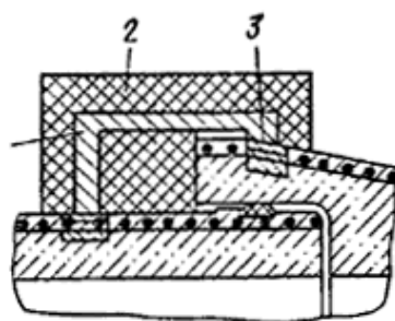
Рис. 2. Общий вид перемишки между арматурой смежных секций труб
