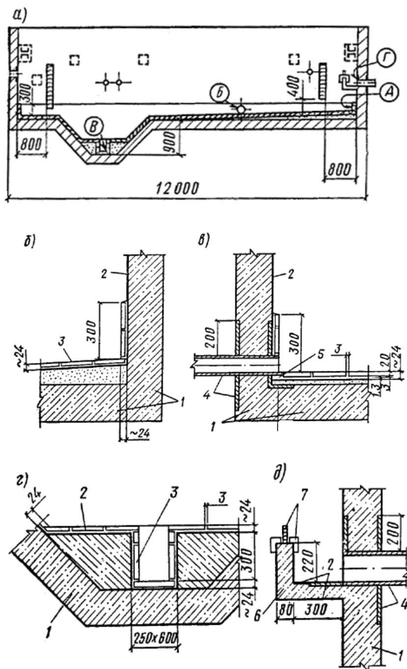
Рис. 3. Нефтеловушка (перекрытие — съемные деревянные щиты)
