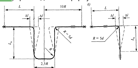
Рисунок 1 — Устройство П-образного (а) и Г-образного (б) компенсаторов
