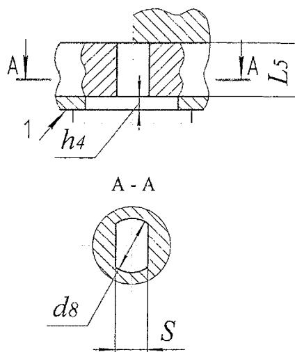
Рисунок 15 – Приводы с плоской головкой
