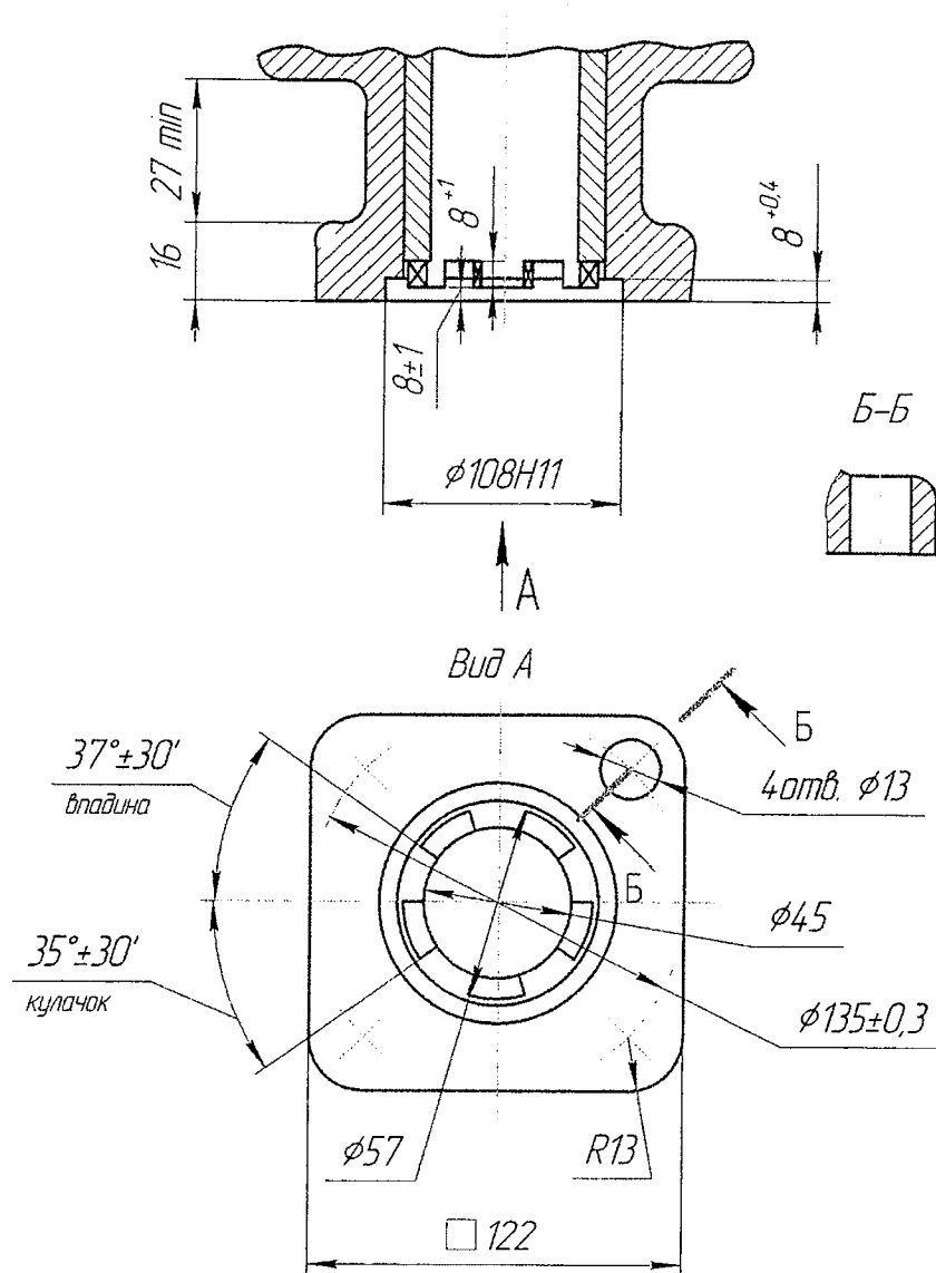
Рисунок А.9 – Присоединение привода типа Б
