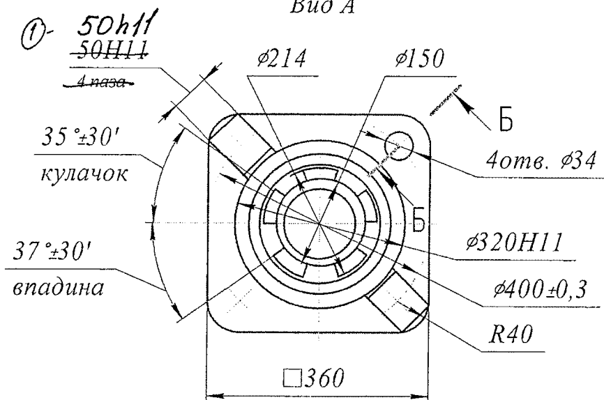
Рисунок А.13 – Присоединение привода типа Д
