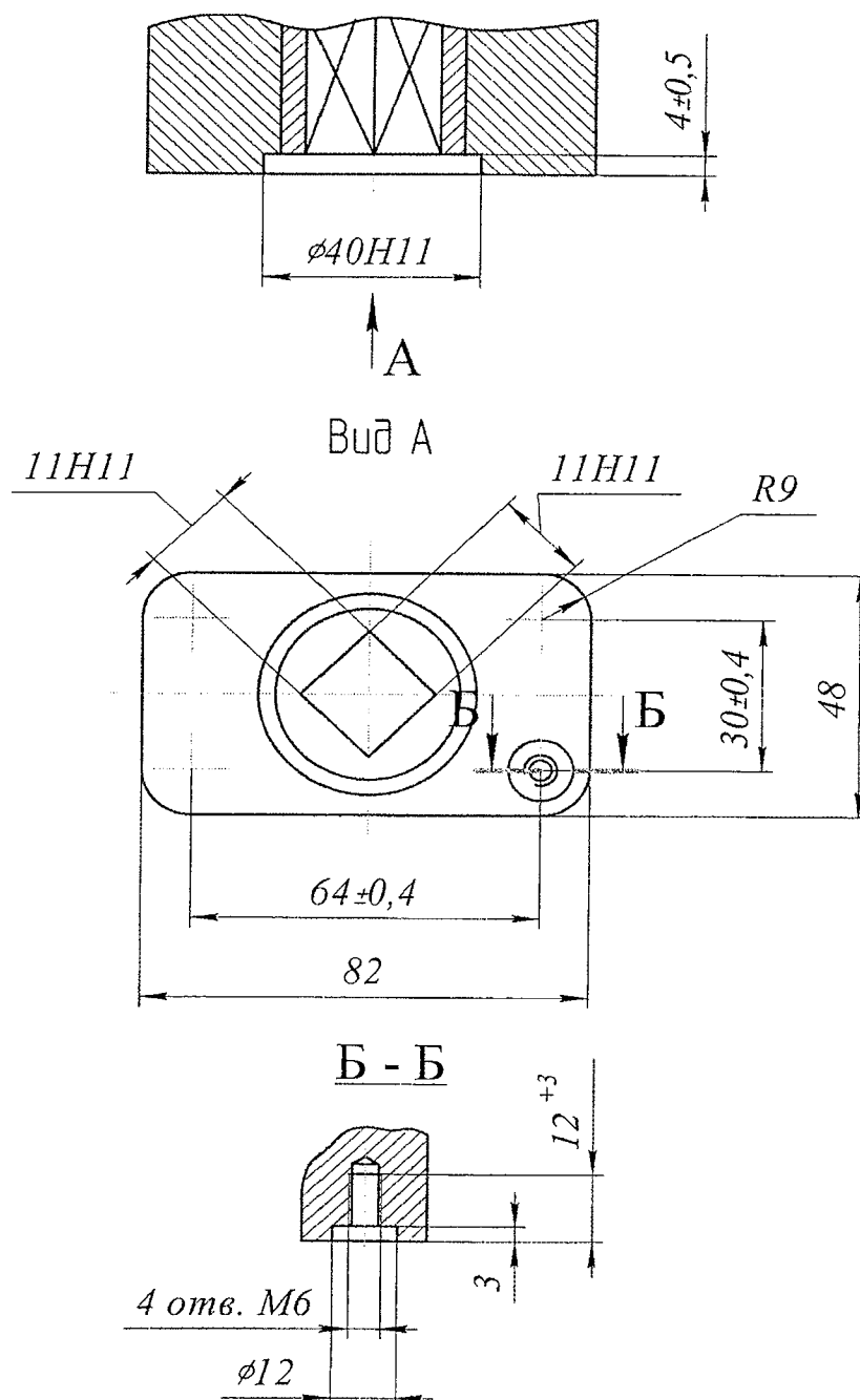
Рисунок А.1 – Присоединение привода типа МЧ
