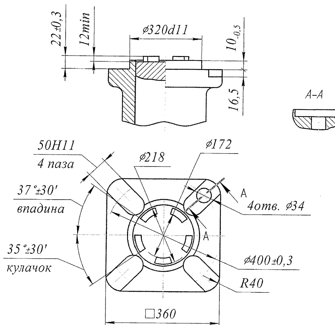
Рисунок А.14 – Ответное присоединение трубопроводной арматуры типа Д
