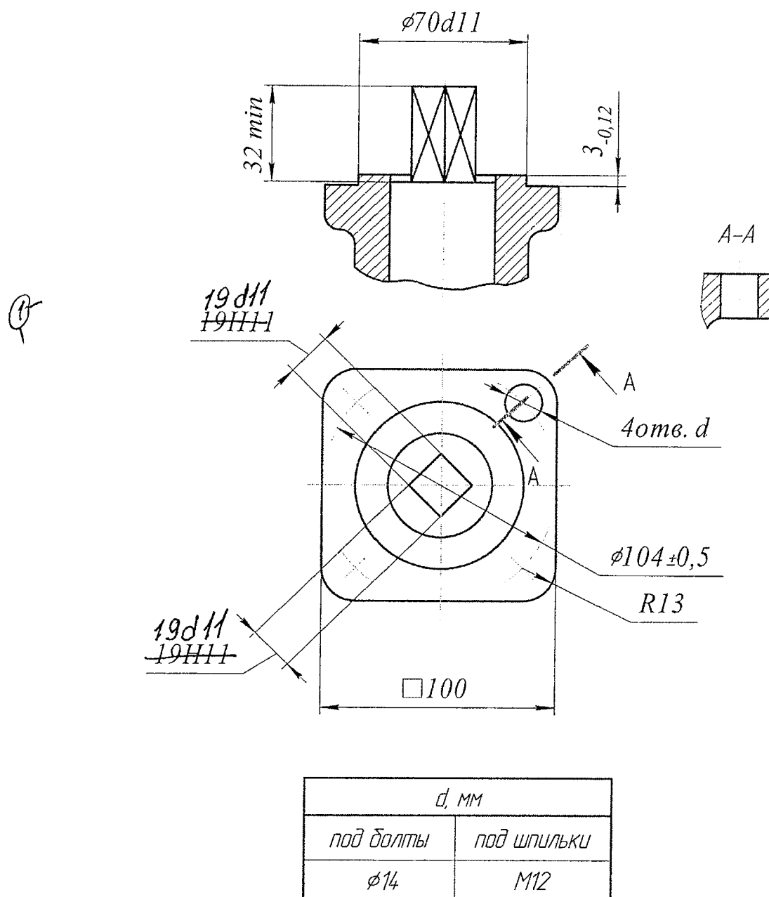
Рисунок А.6 – Ответное присоединение трубопроводной арматуры типа АЧ
