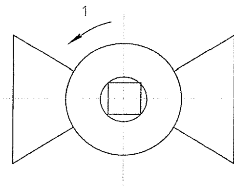
Рисунок 13 – Положение параллельной квадратной головки на закрытой арматуре
