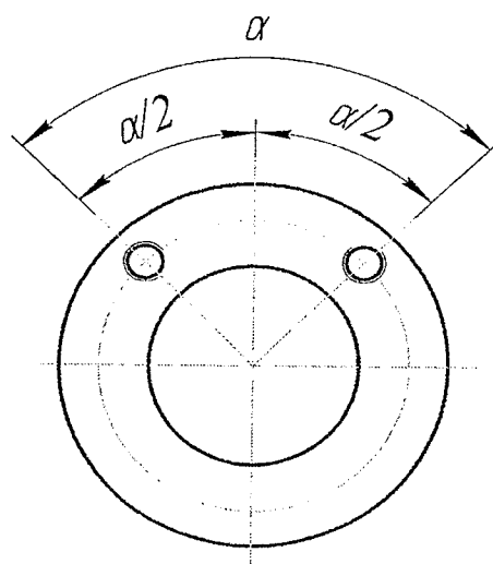
Рисунок 3 – Расположение отверстий для типов присоединений F03–F60
