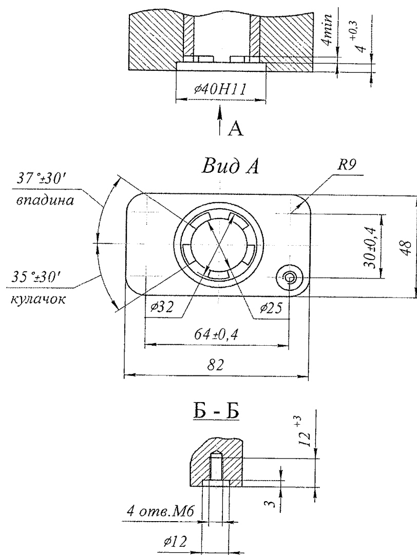
Рисунок А.3 – Присоединение привода типа МК
