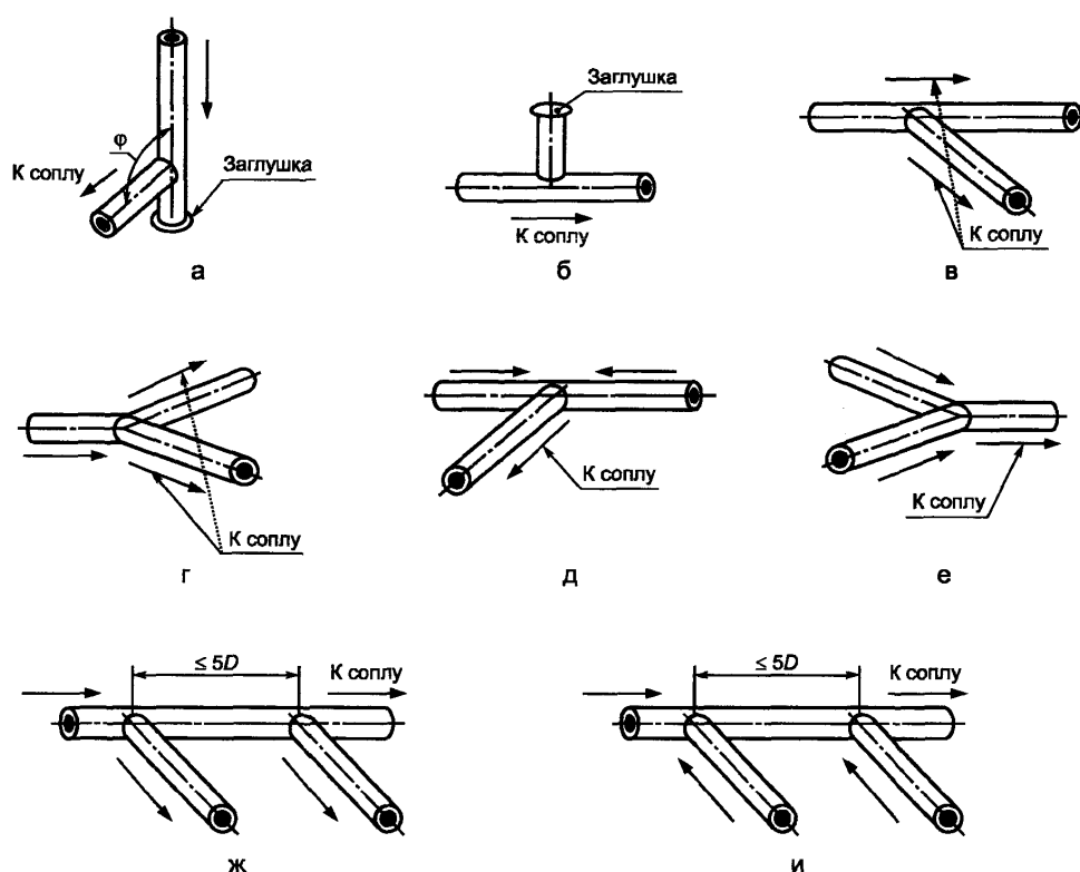
Рисунок А.2 - Тройники
