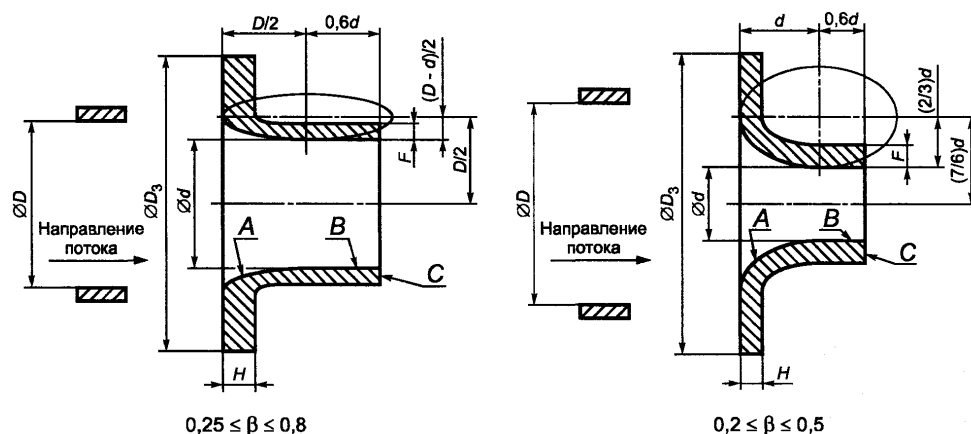
Рисунок 2 - Эллипсное сопло
