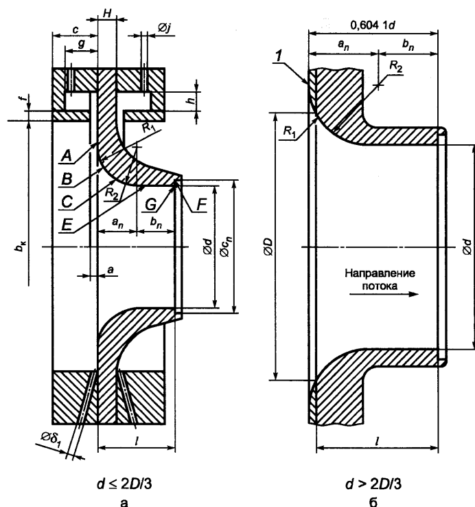
1 - отсекаемая часть сопла Рисунок 1 - Сопло ИСА 1932
