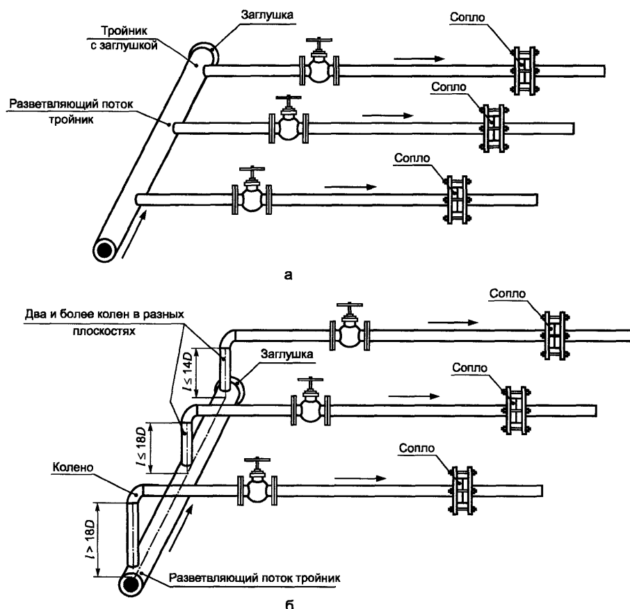
Рисунок 5 - Схемы коллектора
