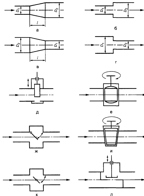
Рисунок А.3 - Переходные участки и запорная арматура
