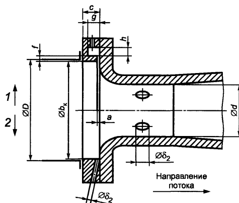
1 - с кольцевой щелью; 2 - с отдельным отверстием
