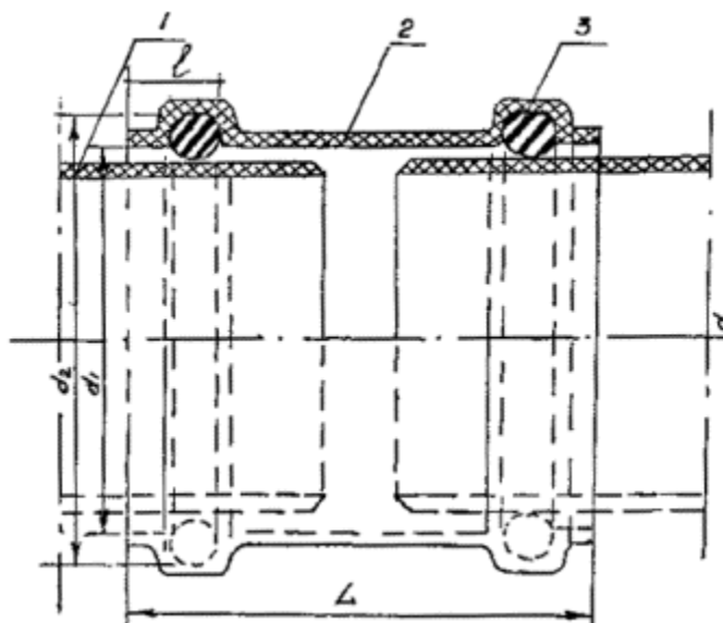
Рис. 3б. Соединение канализационных труб из ПВХ на муфте из ПВХ с уплотнением резиновыми кольцами круглого сечения:
