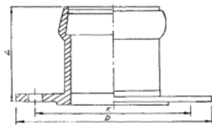
Фланец - раструб Е – КS
