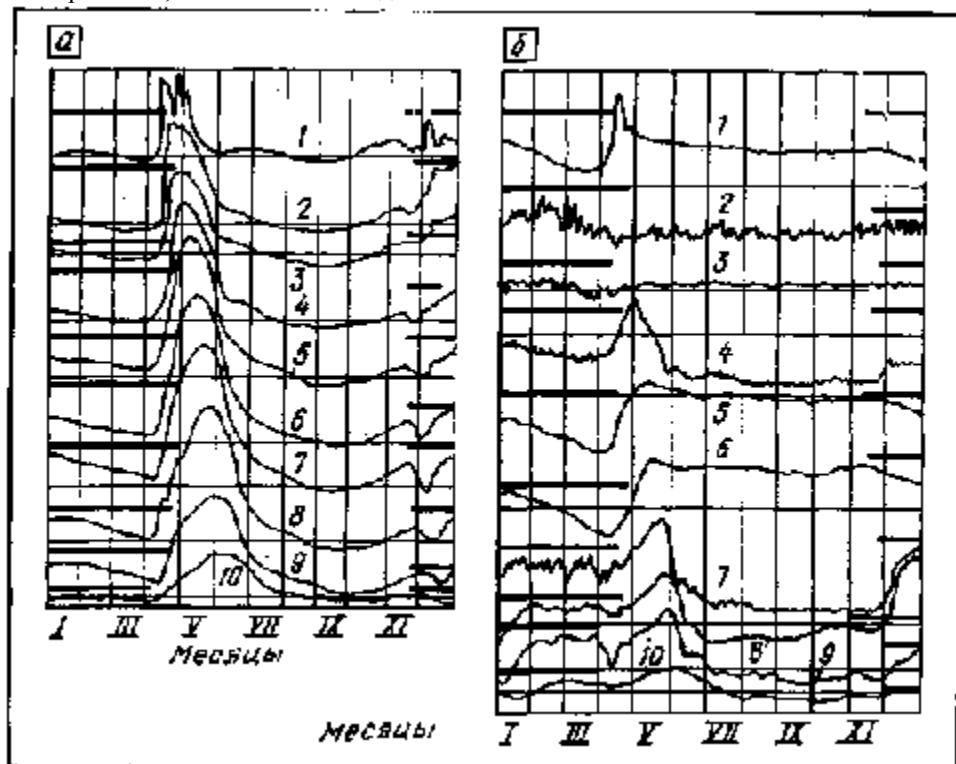
Рис. 2. Графики колебания уровня в Волге до строительства водохранилищ (а) и после строительства (б) (по М. И. Львовичу) 1 — Калинин; 2 — Андропов; 3 — Ярославль; 4 — Горький; 5 — Вязовые; 6 — Тетюши; 7 — Куйбышев; 8 — Саратов; 9 — Волгоград; 10 — Астрахань
