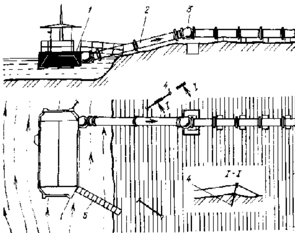
Рис. 16. Водозабор с плавучей насосной станцией заводского изготовления НСП-0,5/10
