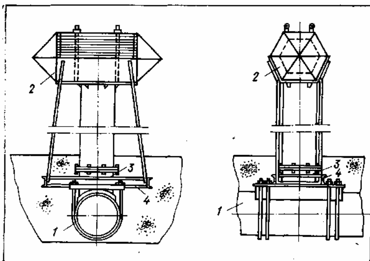
Рис. 39. Дополнительный оголовок на водозаборе из Амуре 1 — самотечный трубопровод; 2 — оголовок; 3 — патрубок; 4 — опорная рама
