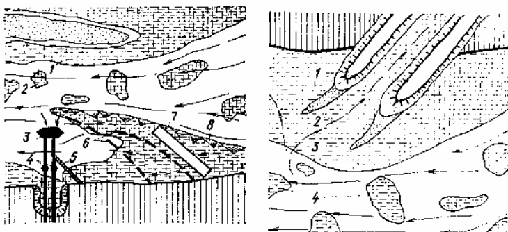
Рис. 48. Шуголедовая обстановка на русловом водозаборе из Оби в предледо-ставный период (ноябрь 1975 г.) 1 — зоны устойчивого ледостава; 2 — шуговые ковры; 3 — основной водоприемник; 4 — дополнительные водоприемные отверстия; 5 — система пневмозащиты; 6 — наплавные буны; 7 — лихтер; 8 — тросы; ———— поверхностные течения; - - - - -глубинные течения
