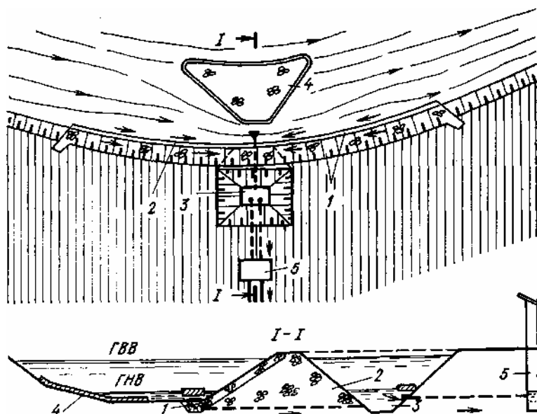
Рис. 79. Водозабор с фильтрующим водоприемником на маловодной реке
