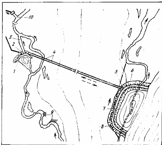
Рис. 46. Приплотинный водозабор на р. Алей с буферным водохранилищем
