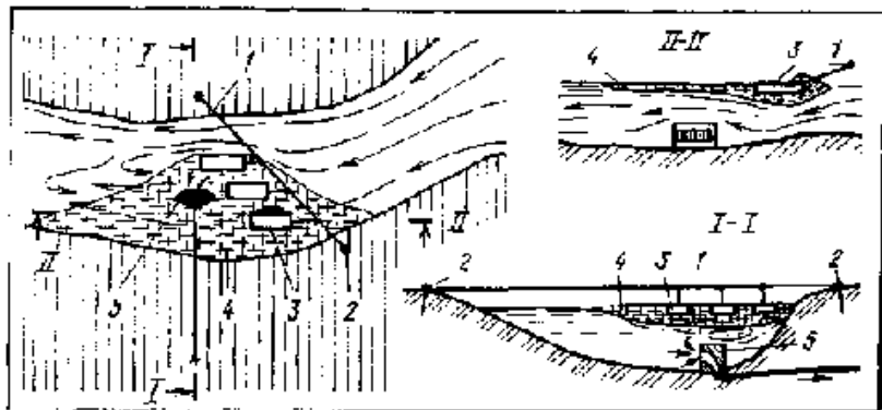
Рис. 58. Применение плотов для ускорения ледостава на малых реках
