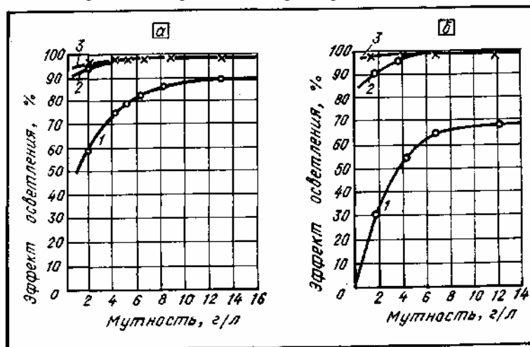
Рис. 77. Эффективность применения флокулянтов для обработки высокомутных вод а — на горных реках; б — на равнинных реках; 1 — безреагентное отстаивание; 2 — с введением ПАА; 3 — с введением ВА-2
