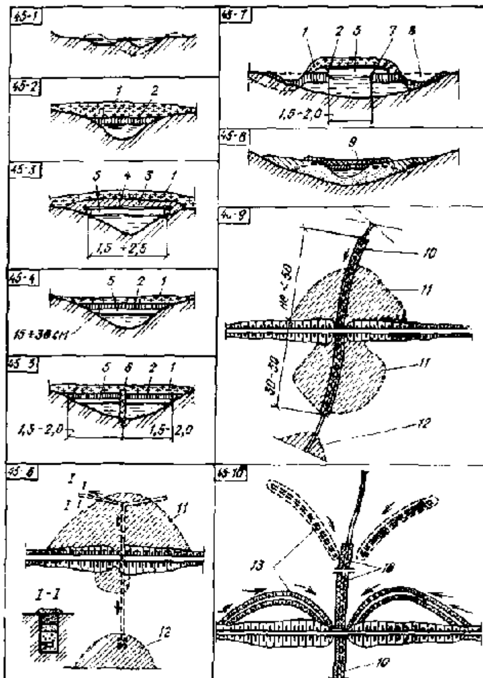
Рис. 45. Противоналедные устройства на малых реках
