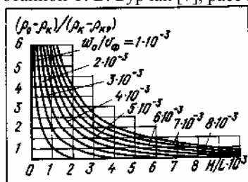
Рис. 87. Номограмма к расчету предварительных отстойников
