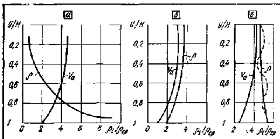
Рис. 4. Распределение мутности по глубине реки в бытовом створе а — насыщенность наносами придонного слоя; б — уменьшение насыщенности по глубине; в — равновесная насыщенность
