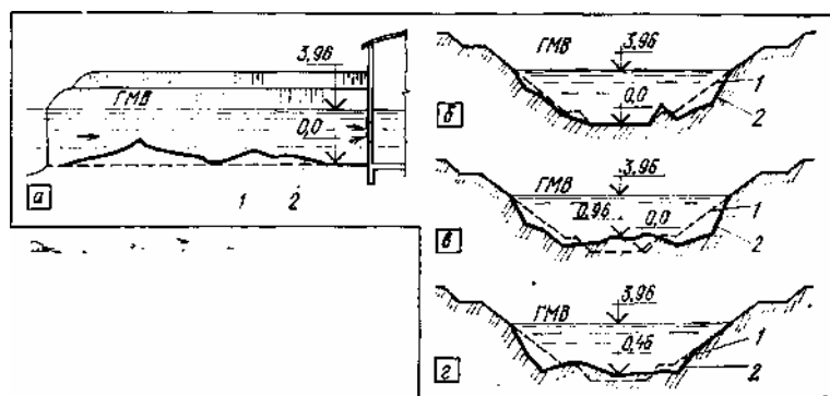
Рис. 26. Водоприемный ковш на р. Чулым
