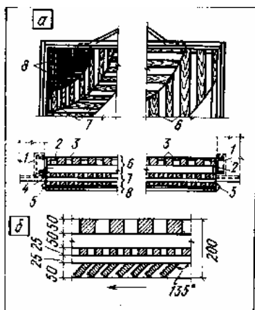
Рис. 33. Пакетно-реечные рыбозащитные кассеты (по В. Н. Ереснову)
