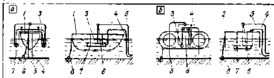
Рис. 17. Временный плавучий водозабор с погружными насосами
