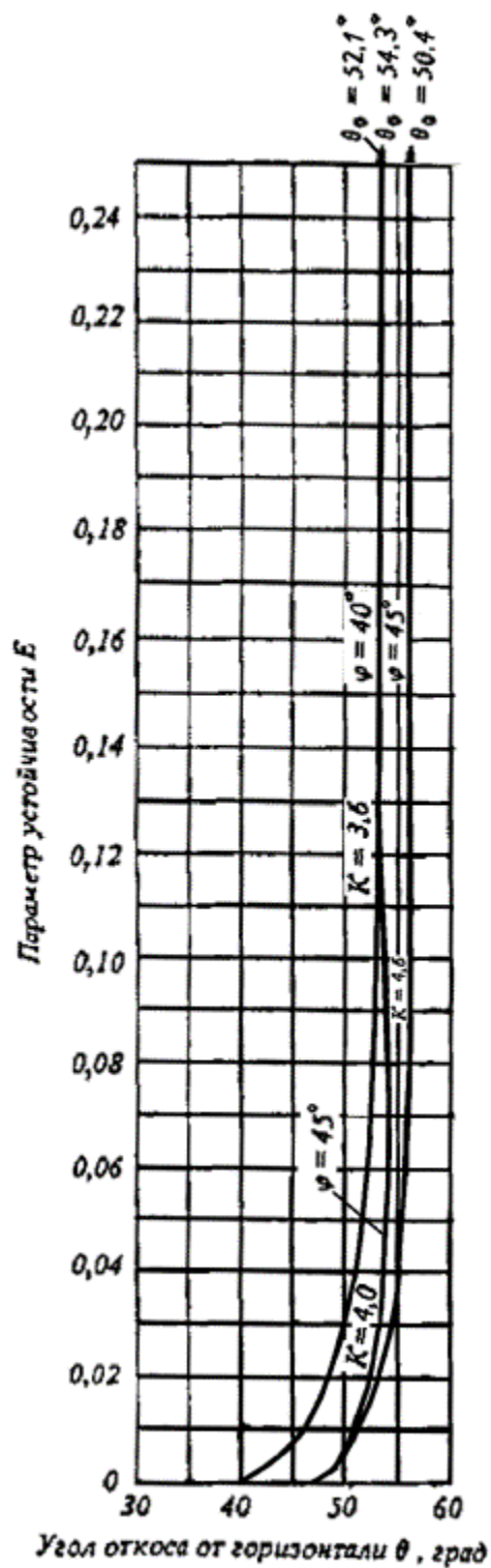
Черт. 5. Графики для определения крутизны откоса при 3 < K < 5
