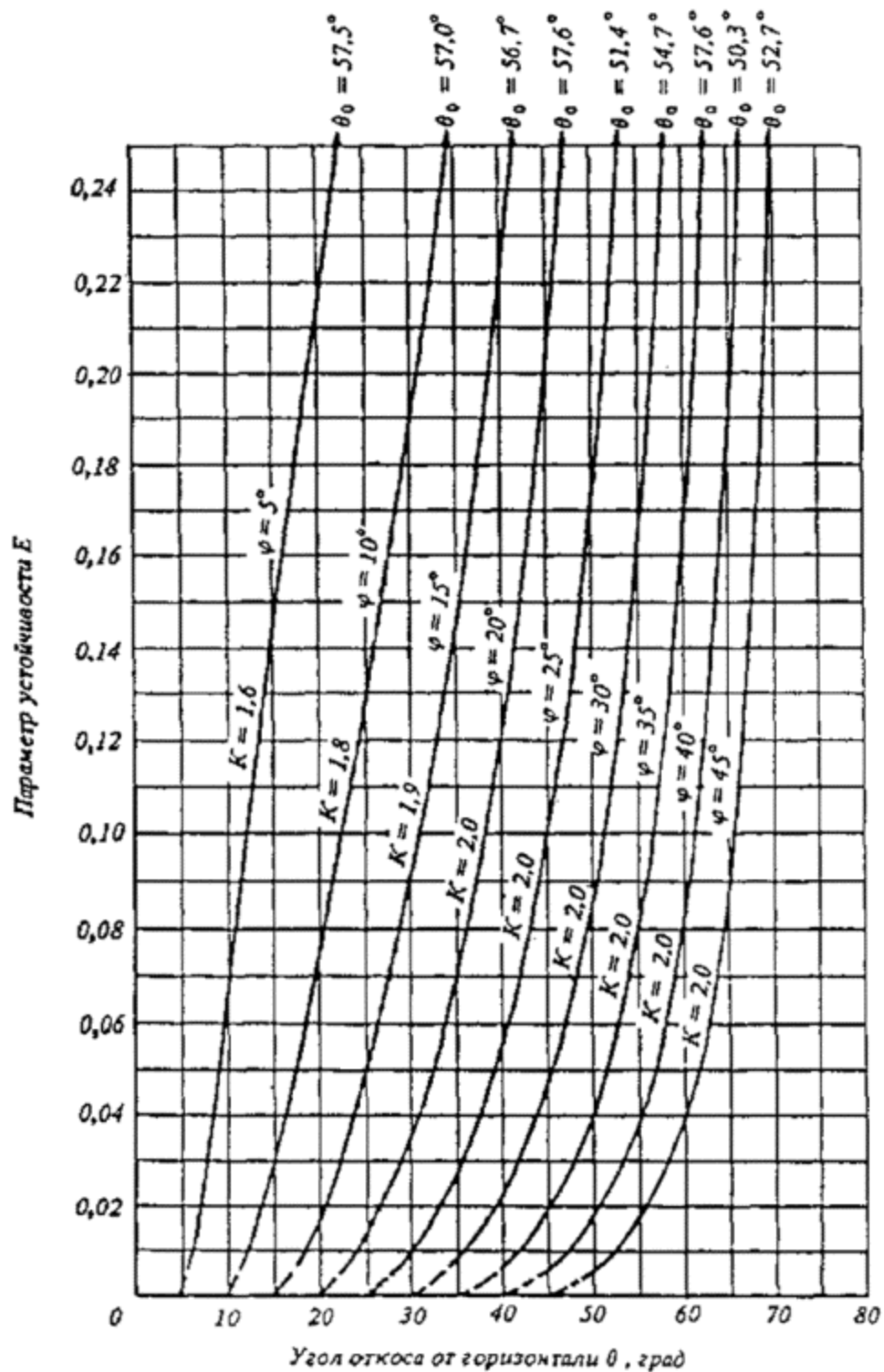
Черт. 3. Графики для определения крутизны откоса при 1 < K < 1
