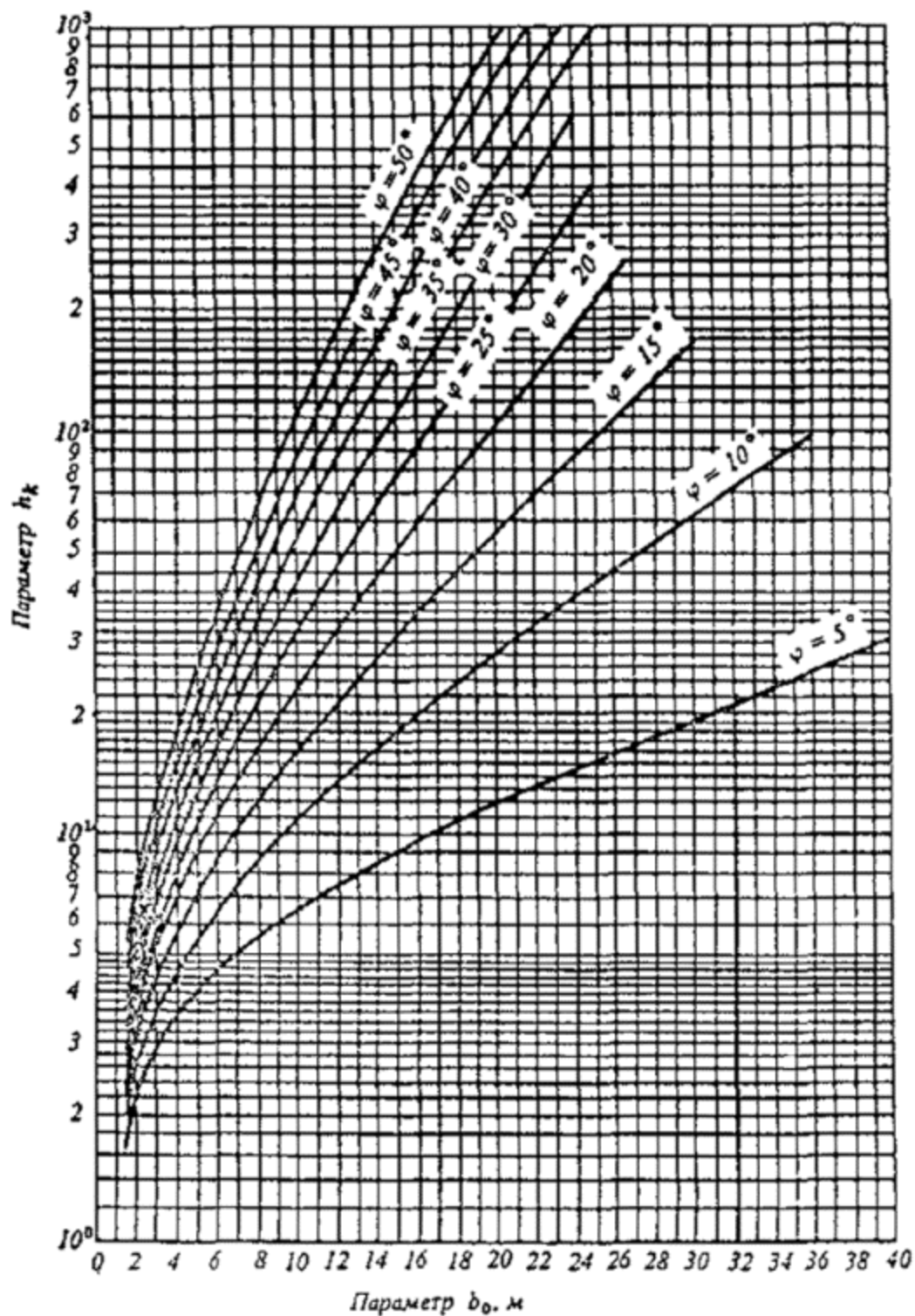
Черт. 6. Графики для определения параметра b_0
