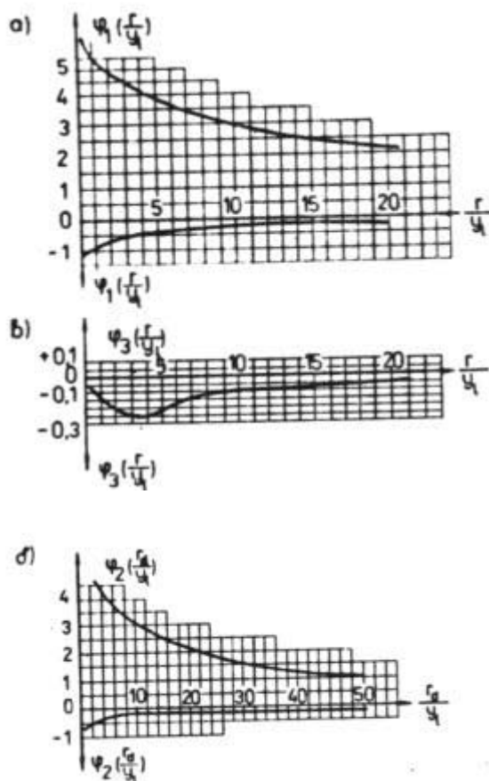
Черт. 5. Графики функций
