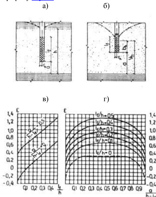
Черт. 3. К расчету сопротивления скважин на гидрологическое несовершенство а, б - схемы несовершенных скважин в напорном и безнапорном пластах; а, г - графики для определения e
