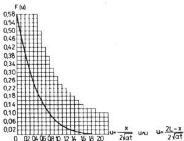
Черт. 1. График функции F(u)
