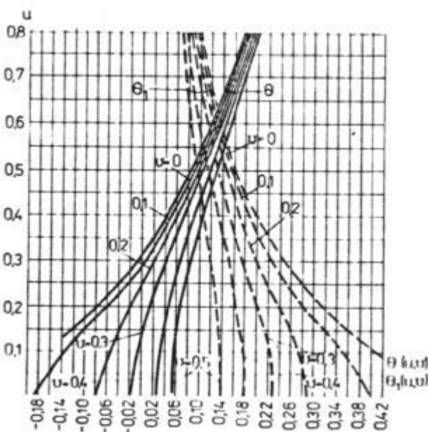
Черт. 4. Графики функций Q(u, v) и Q_1(u, v)
