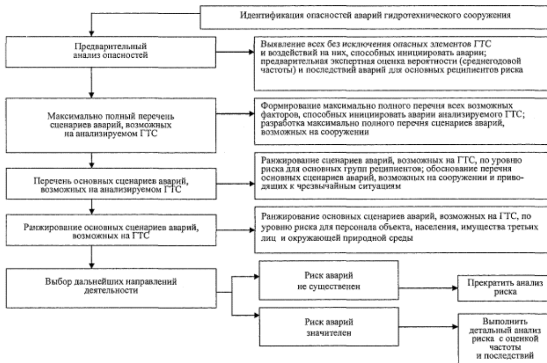
Рис. 3. Основные шаги процедуры идентификации опасностей
