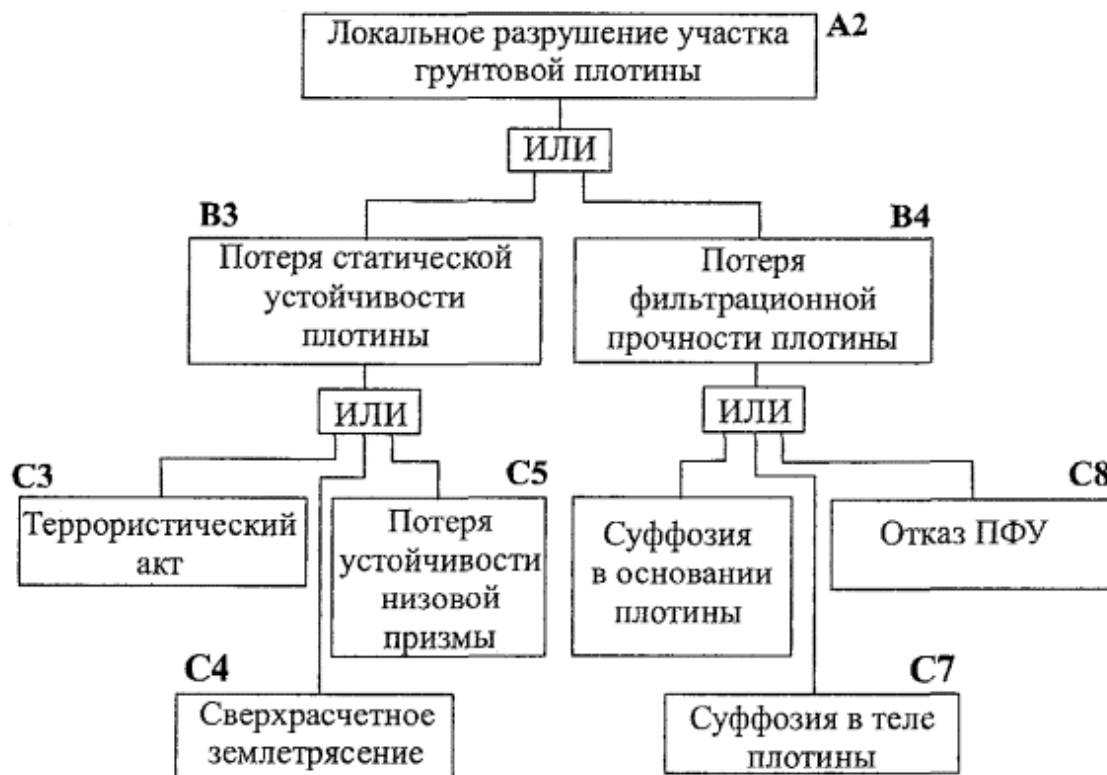
Рис. П.2.3. «Дерево отказов» для сценария аварии A2
