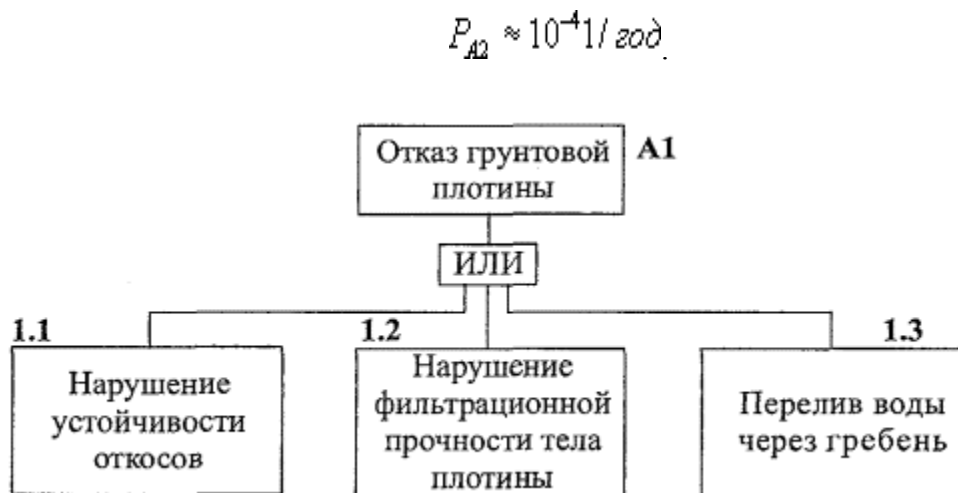
Рис. П.2.8. «Дерево отказов» для грунтовой плотины НГТУ (сценарий A1)
