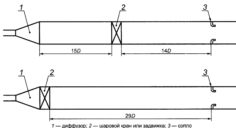
Рисунок 6 - Схема расположения шарового крана или задвижки при \beta = 0,6
