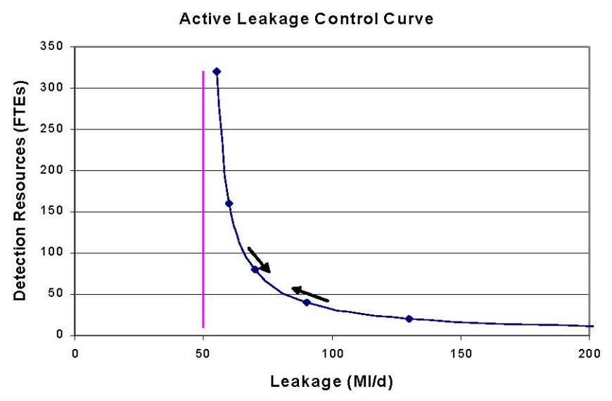
Иллюстрация 3 Активная кривая контроля утечки
