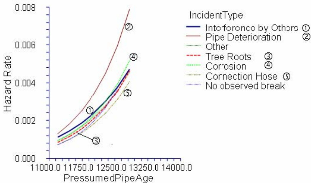
Иллюстрация 4. Заговор нормы опасности, типом инцидента.
