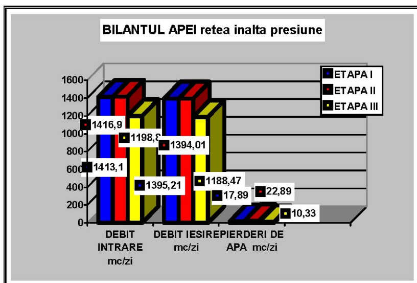
Иллюстрация 6. Водный баланс в высоком давлении (10 уровней) сеть
