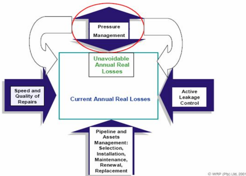
Иллюстрация 1: четыре составляющих диаграммы со вторичными влияниями давления
