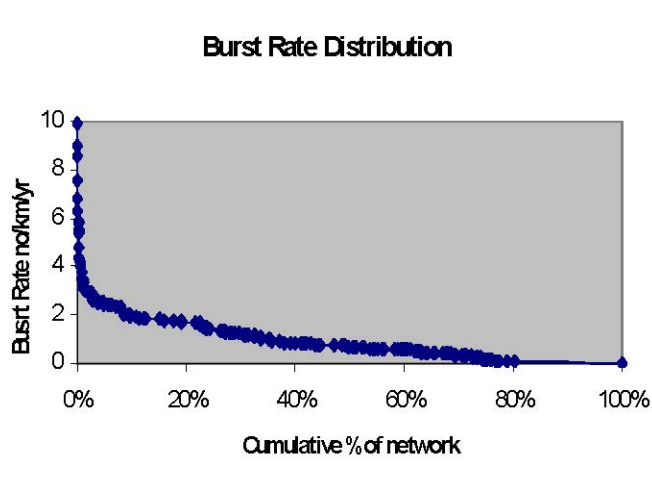
Иллюстрация 5 – Распределение Нормы Взрыва
