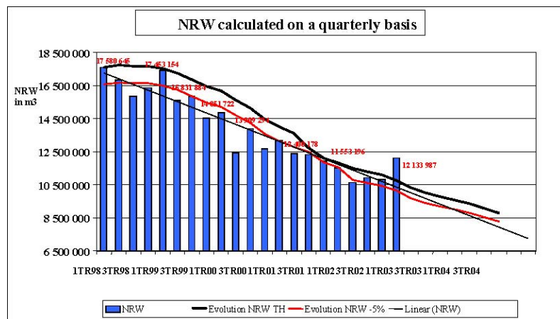
Иллюстрация 5: моделирование NRW в проекте, включая больше чем 10 компонентов (Источник: IWA 2004 – Марракеш – Касабланкский Случай)
