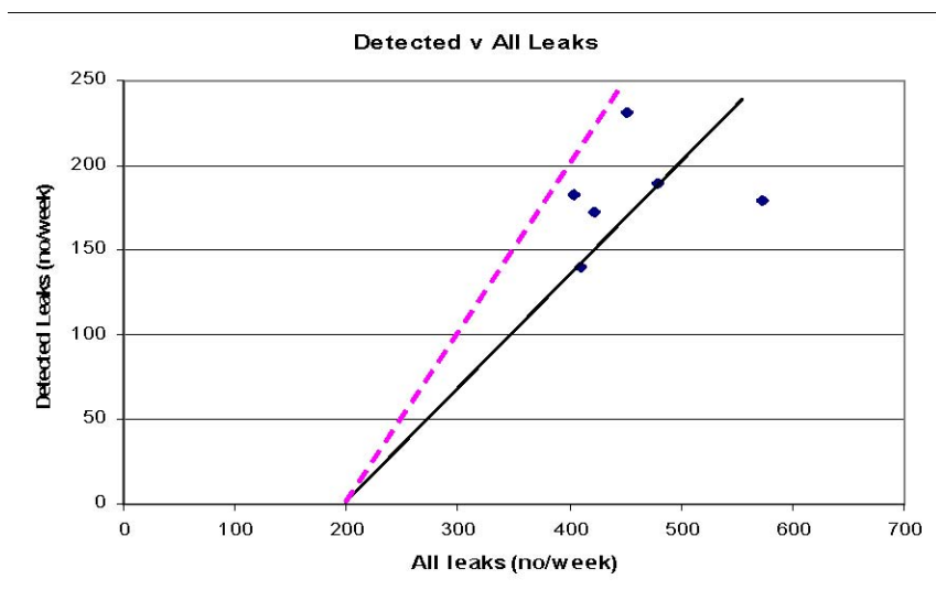
Иллюстрация 8 Сравнение превентивного обнаружения просачивается к общему количеству восстановленных утечек - Социологическое исследование 2
