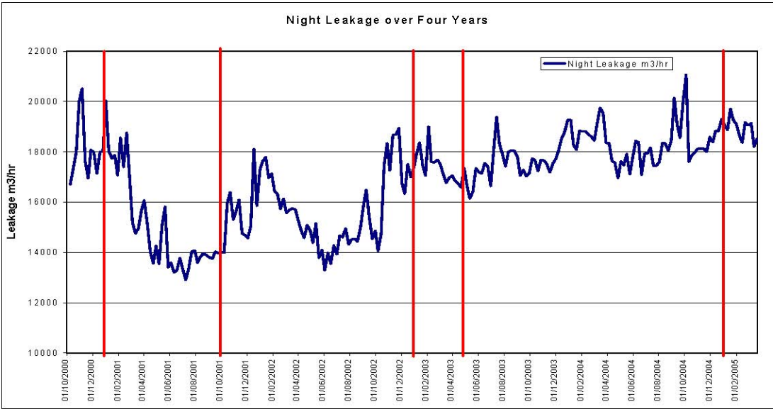
Иллюстрация 4 Отобранные периоды Стола деятельности обнаружения утечки 1 Результат обнаружения в течение четырех периодов – 2001-2004
