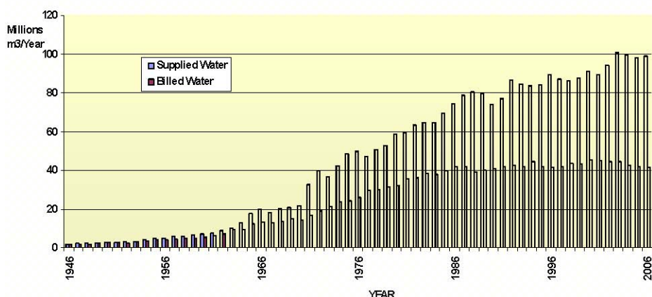
Иллюстрация 1. Поставляемая и объявленная вода в течение периода 1946-2006
