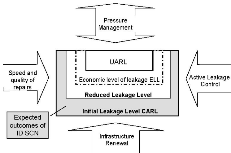
Иллюстрация 3 сокращение Утечки подхода IWA
