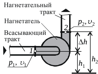
Рис. 1.11. Характеристики насоса
