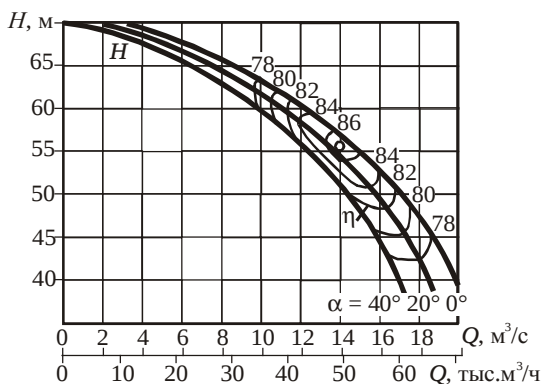
Рис. 1.16. Графическая характеристика насоса 2000ВР-16/63-А при разном угле наклона лопаток а направляющего аппарата
