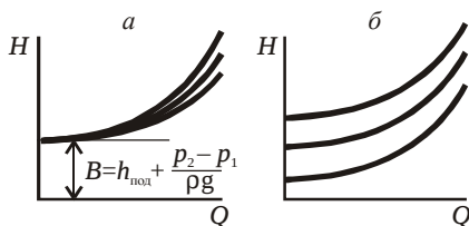
Рис. 2.2. Изменение напорной характеристики сети: а – при изменении коэффициента местного сопротивления; б – при изменении давления в точке нагнетания
