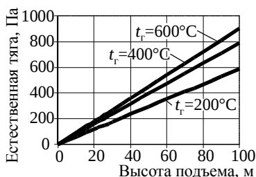
Рис. 2.7. Естественная тяга
