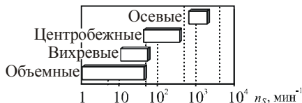
Рис. 4.11. Коэффициент быстроходности насосов
