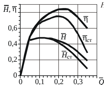
Рис. 4.28. Безразмерная характеристика серии вентиляторов Ц4-76
