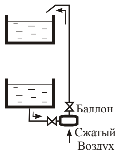
Рис. 1.10. Пневмо-подъемник
