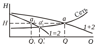
Рис. 3.10. Совместная и индивидуальная работа параллельных нагнетателей
