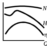
Рис. 5.7. Типичная характеристика осевого нагнетателя
