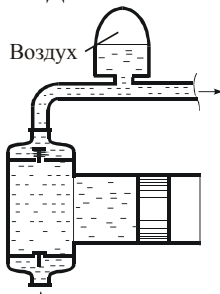
Рис. 6.14. Воздушный колпак на нагнетательном трубопроводе
