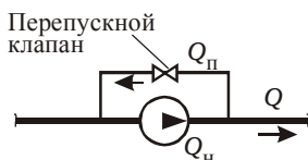
Рис. 4.19. Перепуск среды
