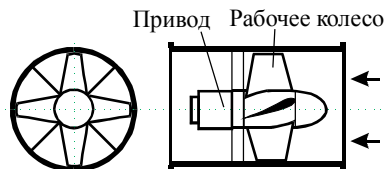
Рис. 1.3. Осевой нагнетатель
