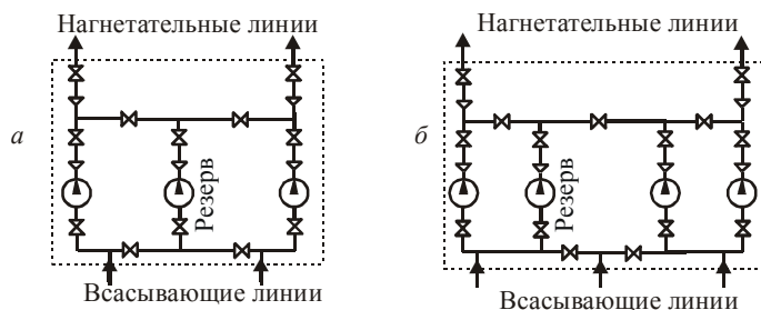
Рис. 7.9. Схема насосной станции:
