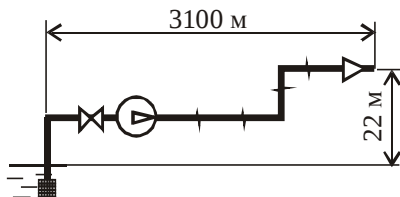
Рис. 2.4. Водопроводная сеть
