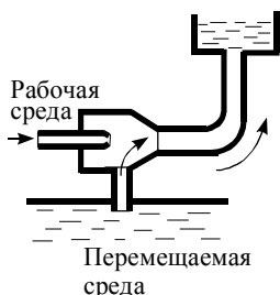
Рис. 1.8. Струйный насос
