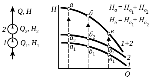
Рис. 3.16. Суммарная напорная характеристика установки из последовательных нагнетателей
