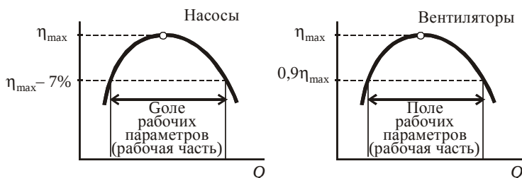
Рис. 1.15. Поле рабочих параметров нагнетателей
