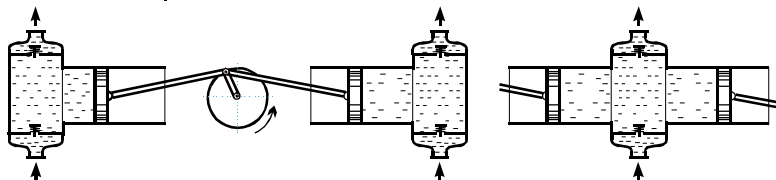
Рис. 6.3. Двухпоршневой насос
