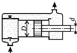
Рис. 6.12. Насос с дифференциальным поршнем
