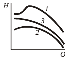
Рис. 4.30. Типичные напорные характеристики вентиляторов: 1 – низкоскоростных; 2, 3 – высокоскоростных
