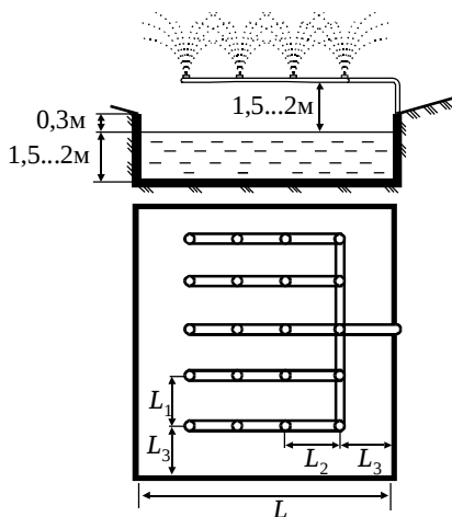
Рис. 7.15. Брызгательный бассейн
