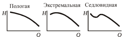
Рис. 1.17. Напорная характеристика динамических нагнетателей
