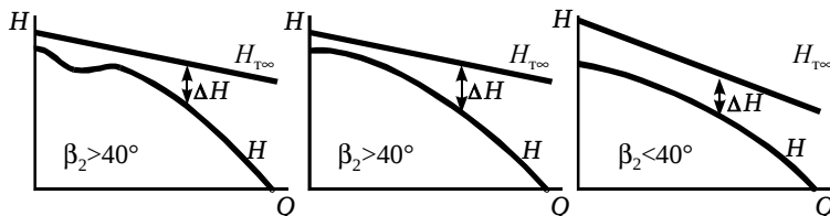
Рис. 4.8. Действительная напорная характеристика динамических нагнетателей
