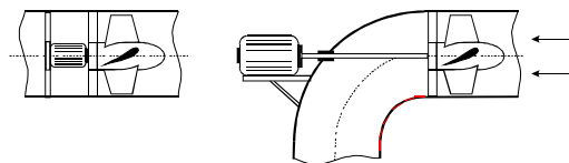
Рис. 5.3. Компоновка осевого нагнетателя с приводом
