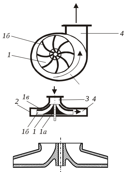
Рис. 4.1. Центробежный нагнетатель:
