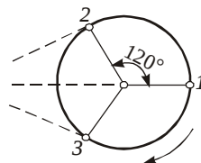
Рис. 6.11. Крепление штоков в трехпоршневом насосе
