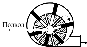
Рис. 6.25. Пластинчатый роторный насос с внутренней подачей
