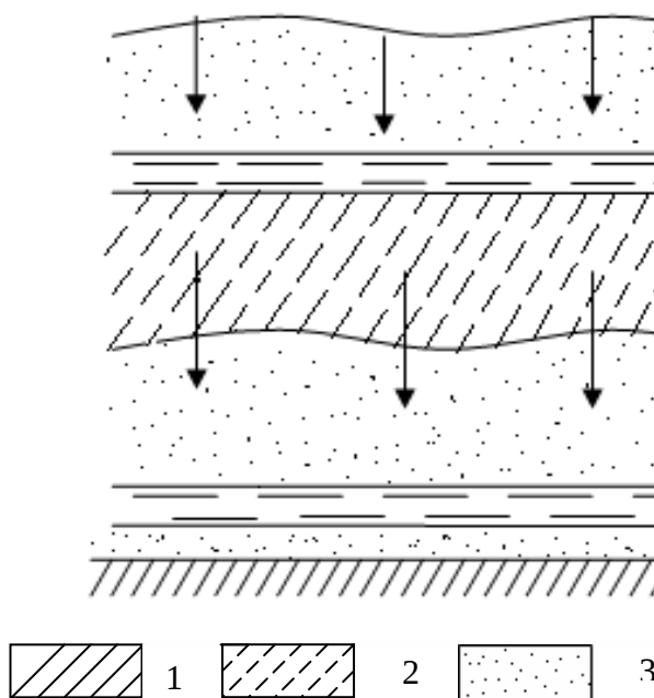
Рис. 1. Схема залегания верховодки на слабопроницаемом водоупоре:
