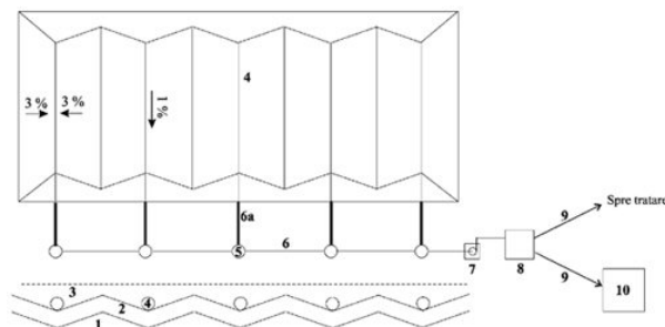
Schema sistemului de colectare a levigatului
