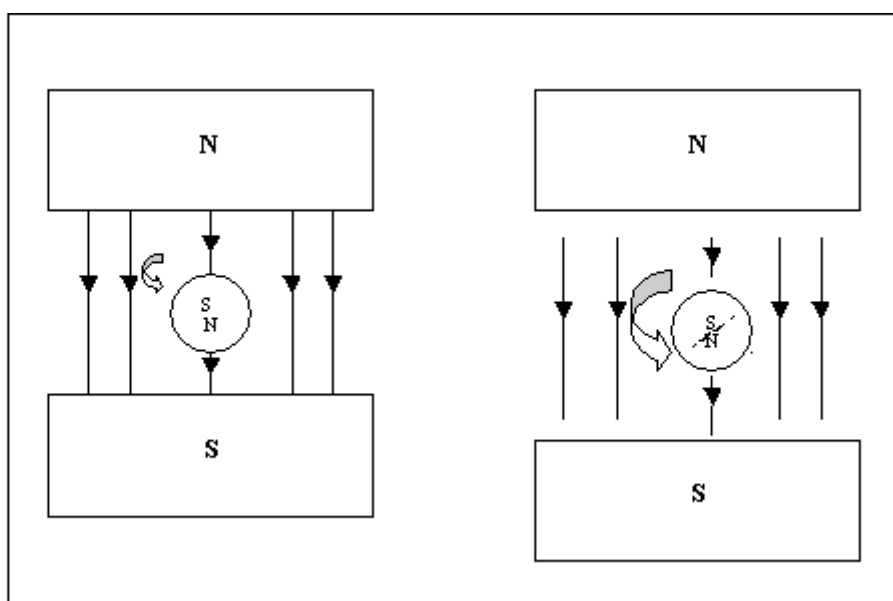
Рис.4. Схема воздействия внешнего постоянного магнитного поля на 2-х и 4-х полюсную магнитную муфту счётчика воды.
