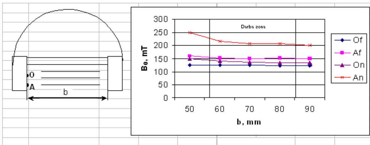
Рис. 7. Влияние расстояния между магнитами (b) на магнитную индукцию ( B_0 ).
