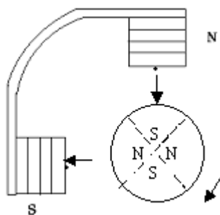
Рис.6. Вариант воздействия внешнего магнитного поля на 4-х полюсную магнитную муфту счетчика воды.
