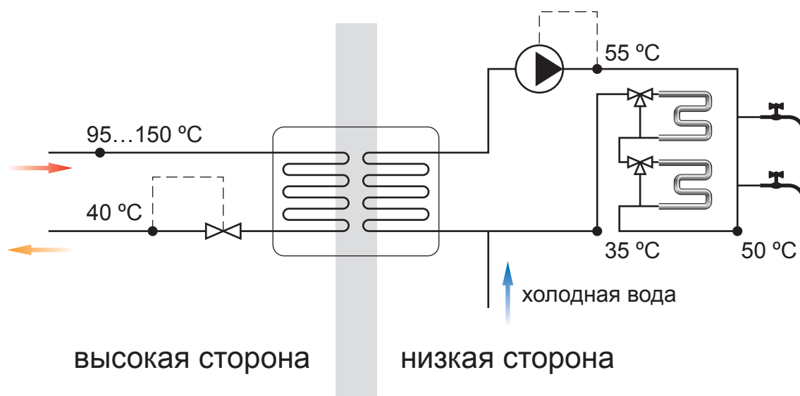
Рис. 6 Независимая система ГВС
