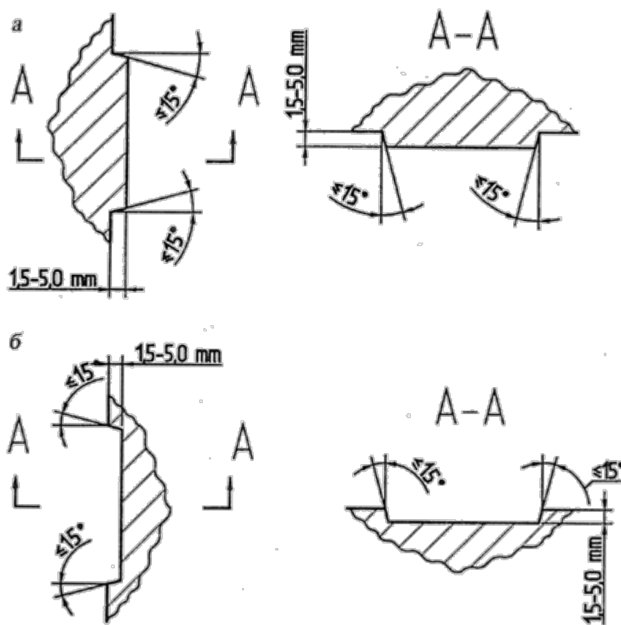
Рис.1 Скосы краев и впадин: а) выступы: б) впадины
