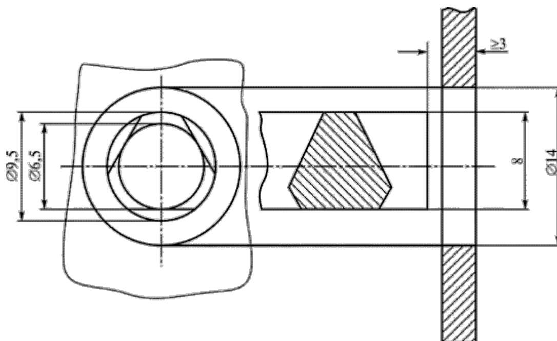
Рис. Треугольная замочная скважина. Размеры указаны в миллиметрах
