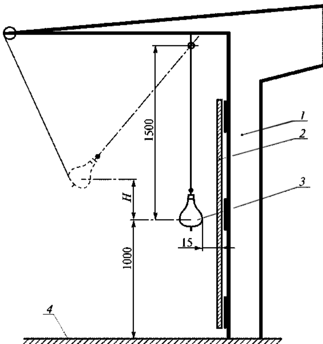
Рис. 1. Испытательный стенд: 1 - рама; 2 - испытываемая стеклянная панель; 3 - маятник; 4 - уровень пола, относящийся к испытываемой стеклянной панели; H - высота панели
