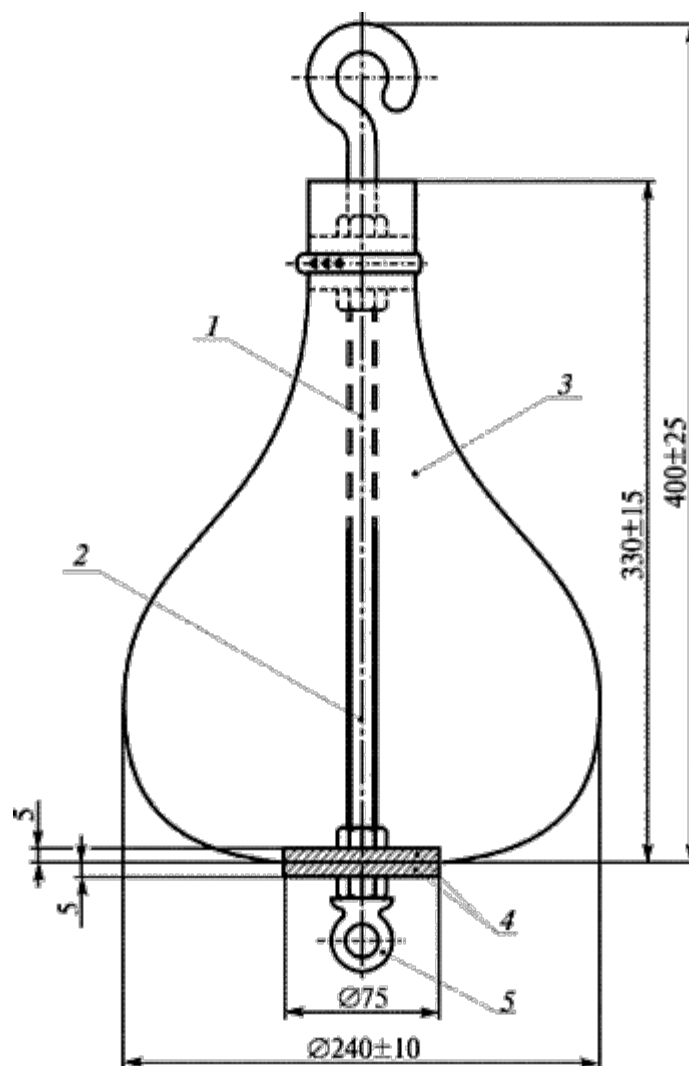
Рис. 3. Маятник для нежесткого удара:
