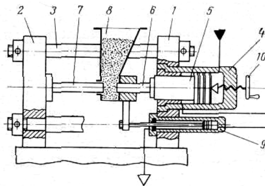
Рис. 5.2 Гидравлическая таблеточная машина:
