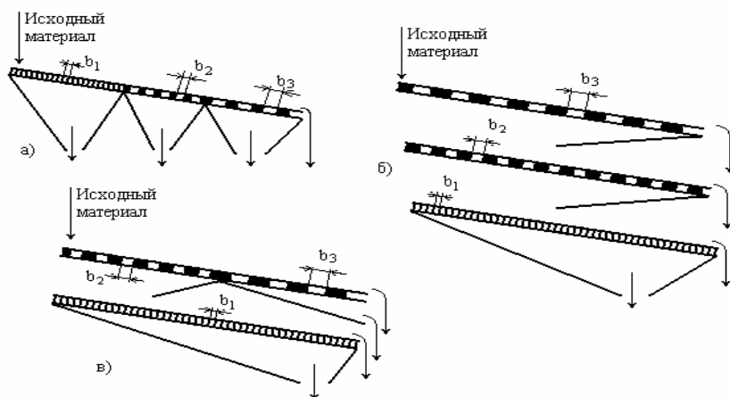
Рис. 4.5 Схемы грохочения
