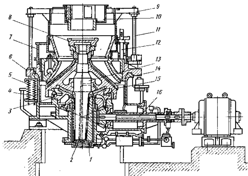
Рис. 3.5 Дробилка КМД с консольным валом
