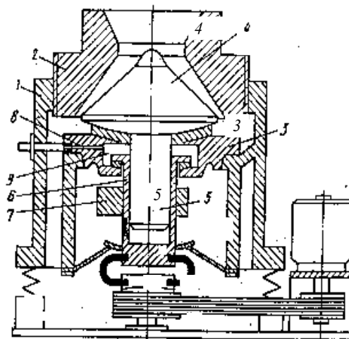
Рис. 3.7 Конусная инерционная дробилка
