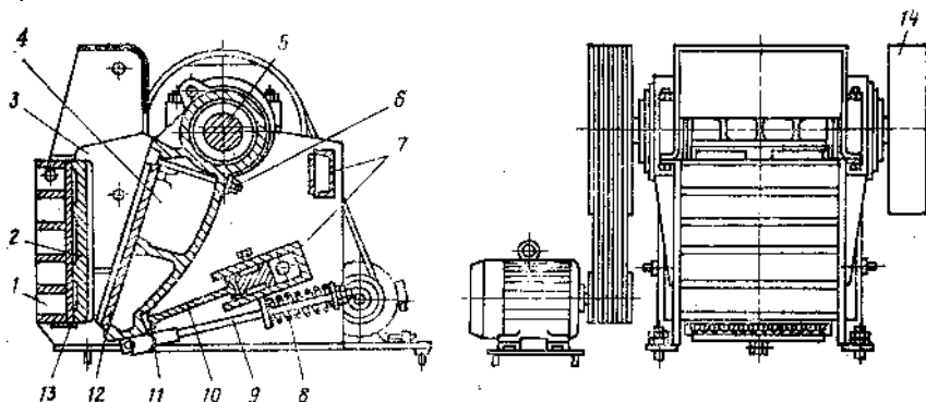
Рис. 3.2. Дробилка ЩДС
