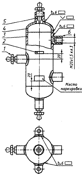
1 — пробка; 2 — ушко; 3 — обечайка; 4 — днище; 5 — штуцер; 6 — штуцер
