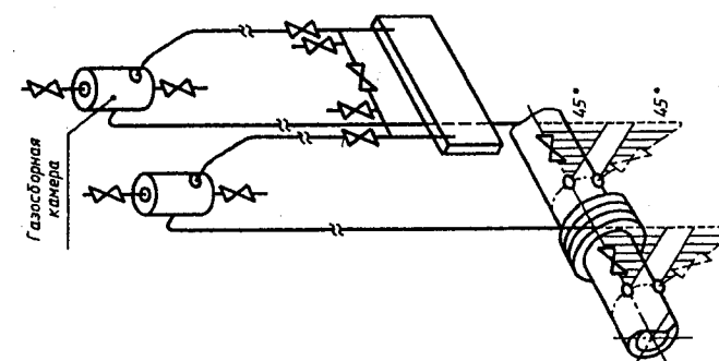
Рисунок В.16 — Дифманометр над трубопроводом
