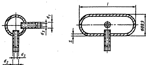
Рисунок 1 — Уравнительные сосуды, рекомендуемые [1]
