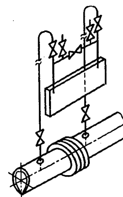
Рисунок В.1 — Дифманометр над трубопроводом
