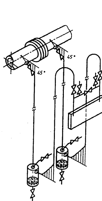
Рисунок В.10 — Дифманометр под трубопроводом (вариант)
