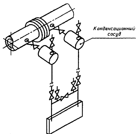
Рисунок В.5 — Дифманометр под трубопроводом
