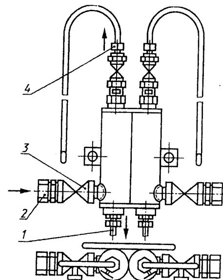
1 — выходной патрубок; 2 — входной патрубок; 3 — кран; 4 — вентиляционный патрубок
