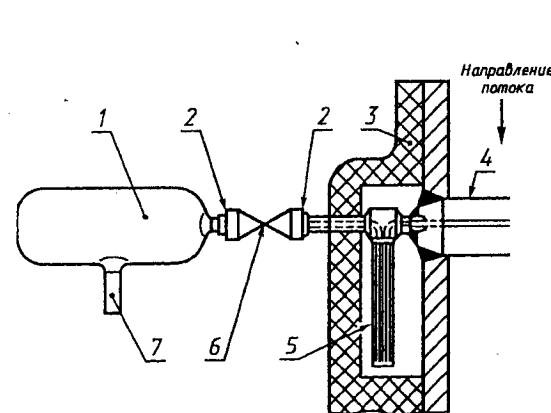
1 — конденсационный сосуд; 2 — сварные соединения; 3 — изоляция; 4 — сужающее устройство; 5 — ловушка; 6 — кран; 7 — соединительная трубка Рисунок 4 — Монтаж аппаратуры для пара высокого давления и высокой температуры на вертикальном трубопроводе
