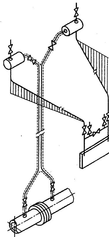
Рисунок В.7 — Дифманометр над трубопроводом
