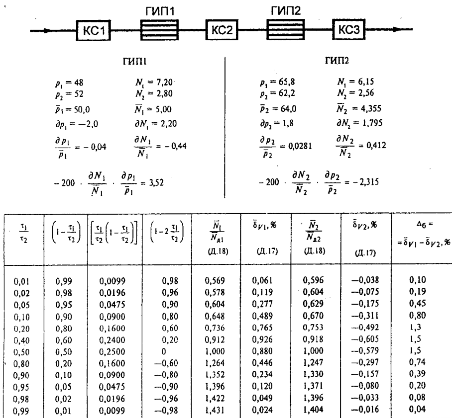
Рисунок Д.1 — Схема участка трубопровода и расчет дополнительной систематической погрешности ГИП
