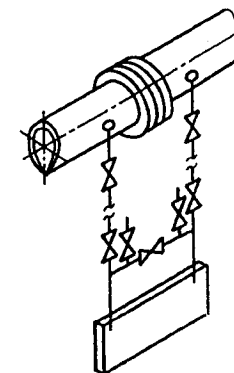
Рисунок В.2 — Дифманометр под трубопроводом
