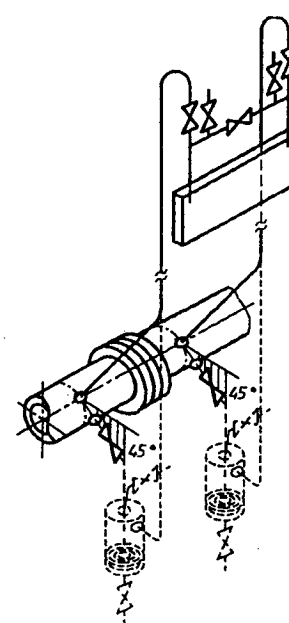
Рисунок В.11 — Дифманометр над трубопроводом (два варианта)
