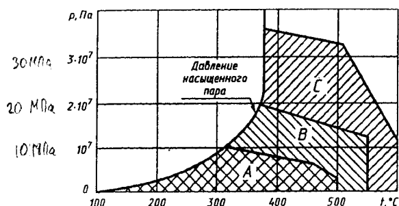
Рисунок 2 — Область применения уравнительных сосудов
