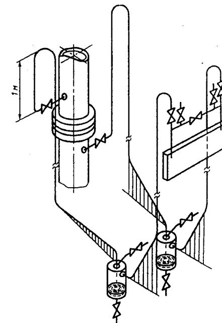
Рисунок В.12 — Дифманометр ниже отверстий для отбора давления. Вертикальный трубопровод
