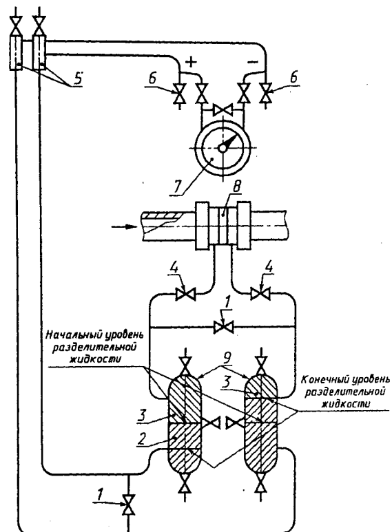
1 — уравнительный вентиль; 2 — разделительная жидкость; 3 — контролируемая жидкость; 4 — запорный вентиль; 5 — газосборник; 6 — продувочный вентиль; 7 — дифференциальный манометр; 8 — сужающее устройство; 9 — разделительный сосуд Рисунок Б.8
