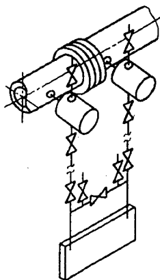
Рисунок В.6 — Дифманометр под трубопроводом (вариант)
