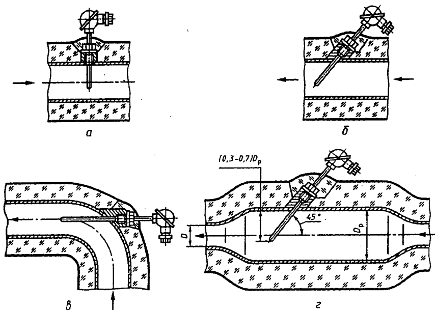
Рисунок 11 — Схема установки чувствительного преобразователя термометра
