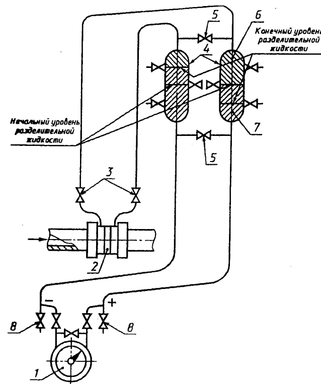
1 — дифференциальный манометр; 2 — сужающее устройство; 3 — запорный вентиль сужающего устройства; 4 — разделительный сосуд; 5 — уравнительный вентиль; 6 — контролируемый газ; 7 — разделительная жидкость; 8 — продувочный вентиль
