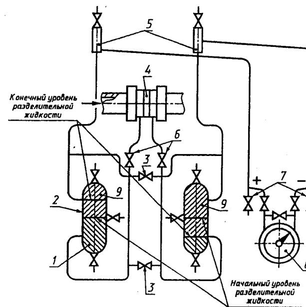
1 — контролируемая жидкость; 2 — разделительный сосуд; 3 — уравнительный вентиль; 4 — сужающее устройство; 5 — газосборник; 6 — запорный вентиль; 7 — продувочный вентиль; 8 — дифференциальный манометр; 9 — разделительная жидкость Рисунок Б.9
