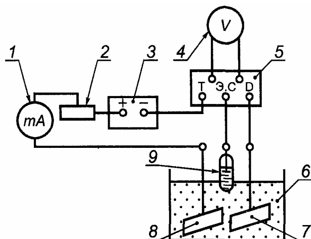
"Рис. Б.1. Схема установки для определения плотности катодного тока"
