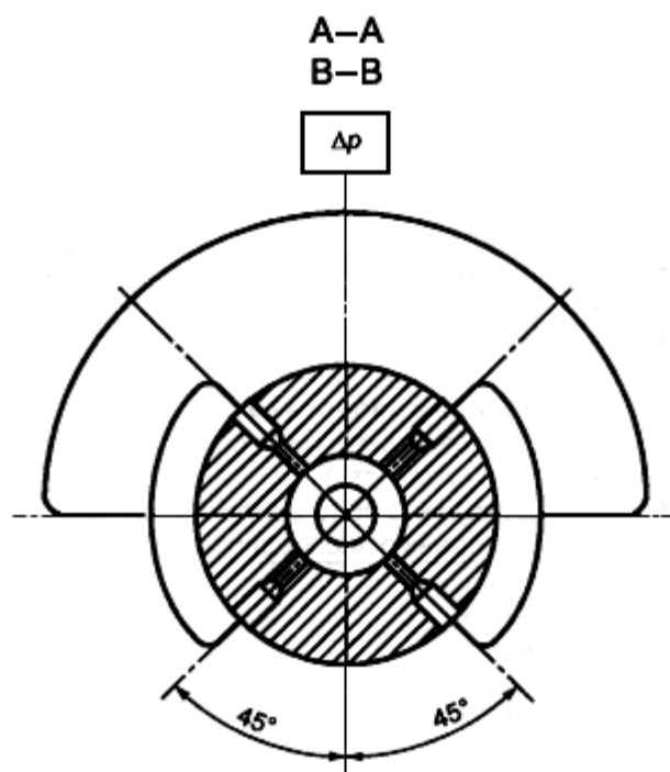
а) Сечение А-А (до СУ) и сечение В-В (после СУ).
