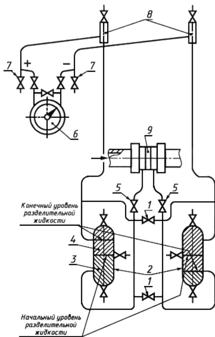
1 - уравнильный вентиль; 2 - разделительный сосуд; 3 - измеряемая жидкость; 4 - разделительная жидкость; 5 - кран; 6 - ППД; 7 - продувочный вентиль; 8 - газосборник; 9 - СУ
