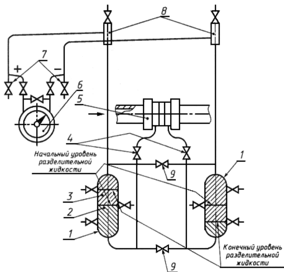
1 - разделительный сосуд; 2 - измеряемая жидкость; 3 - разделительная жидкость; 4 - кран; 5 - СУ; 6 - ППД; 7 - продувочный вентиль; 8 - газосборник; 9 - уравнильный вентиль
