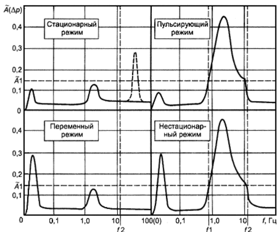
Рисунок Ж.1 - Характерные виды АЧС \tilde{A}(f) на диафрагме при нестационарном потоке природного газа
