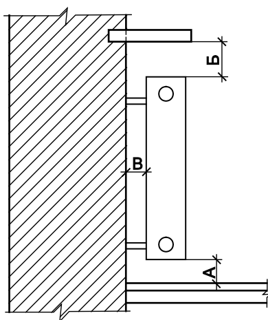
А, Б, В — расстояния от отопительного прибора до строительных конструкций
