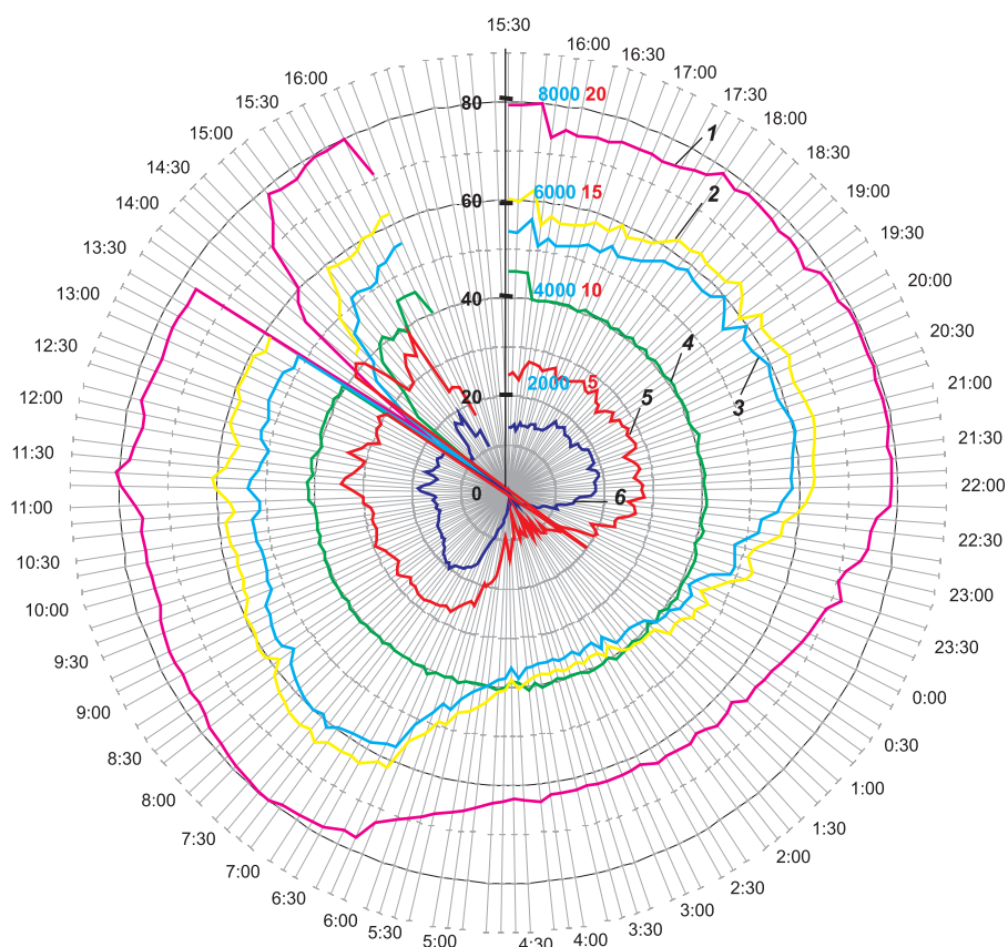
Рис. 5.11. Характеристики режимов совместной работы системы ПРВ от насосной станции № 25А
