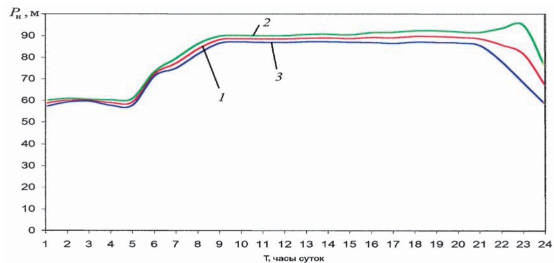
Рис. 5.19. Изменение давления на выходе насосной станции № 25А, P_n = f(T) :
