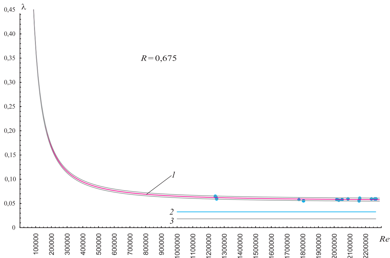
Рис. 3.46. Регрессионная зависимость \lambda = f(Re) с доверительным интервалом регрессии P = 95 \% для водовода диаметром 1600 мм ( L = 6\,558 м): 1 — по формуле (3.39); 2 — по Альтшулю; 3 — по Шевелеву
