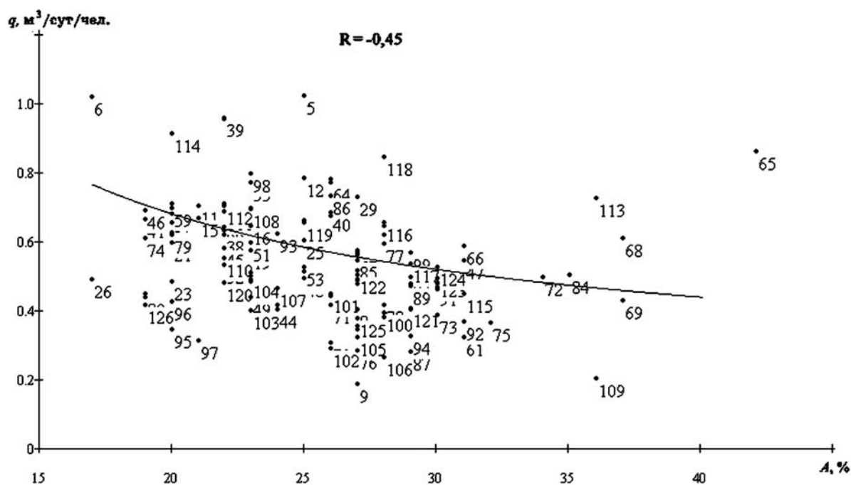
Рис. 4.11. Корреляционная зависимость удельного среднесуточного водопотребления от среднегодового альбеда
