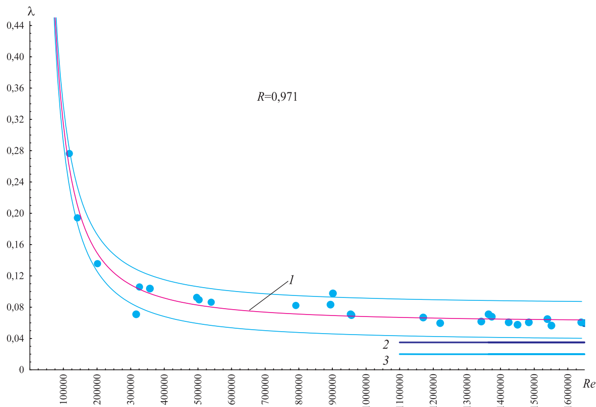
Рис. 3.33. Регрессионная зависимость \lambda = f(Re) с доверительным интервалом регрессии P = 95\% (водовод диаметром 1200 мм; L = 14\,902 м): 1 — по формуле (3.13); 2 — по Альтшулю; 3 — по Шевелеву
