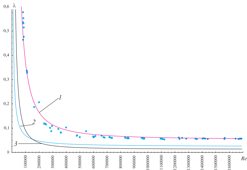
Рис. 3.56. Зависимость \lambda = f(Re, \bar{\Delta}) : 1 — по формуле (3.58) при \bar{\Delta} = 0,01468 ; 2 — по формуле (3.58) при \bar{\Delta} = 0,0003582 ; 3 — по (3.1) Ф.А. Шевелева
