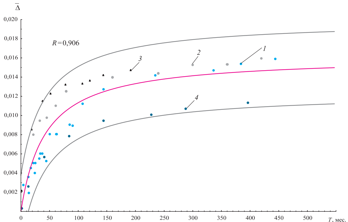
Рис. 3.58. Изменение величины относительной макрошероховатости \bar{\Delta} = f(T) для водоводов диаметром 1200–1600 мм: 1 — d=1200 (эксплуатация 37 лет); 2 — d=1400 (эксплуатация 35 лет); 3 — d=1400 (эксплуатация 16 лет); 4 — d=1600 (эксплуатация 33 года); 1, 2, 4 — источник воды — Северский Донец; 3 — источник воды — Днепр
