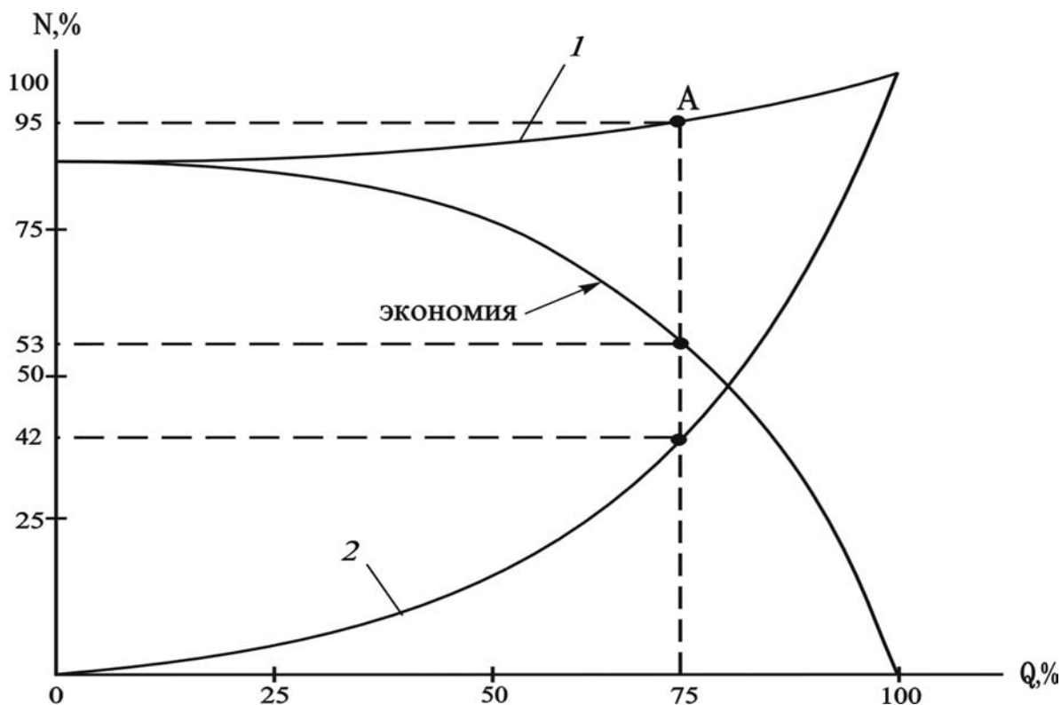
Рис. 5.7. Экономия электроэнергии при регулировании насоса с помощью преобразователя частоты:
