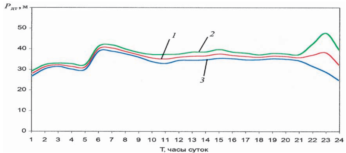
Рис. 5.20. Изменение давления в диктующей точке, P_{\text{дт}} = f(T) :
