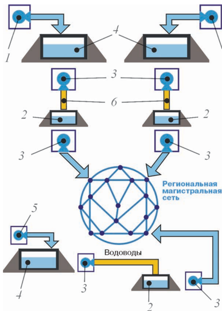
Рис. 5.1. Пример распространенной структуры водоснабжения: 1 — выходные станции 2-го подъема; 2 — зональные резервуары; 3 — насосные станции; 4 — региональные резервуары; 5 — выходная станция; 3-го подъема; 6 — водоводы
