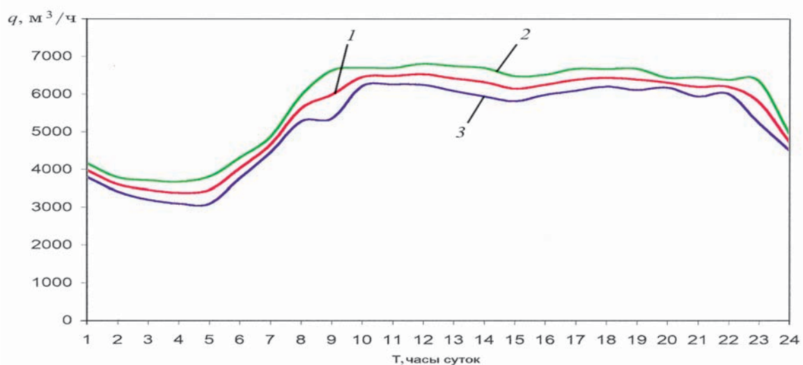
Рис. 5.21. Изменение водопотребления Алексеевского жилого массива от насосной станции № 25А, q = f(T) : а – будние дни; б – суббота; в – воскресенье; 1 – q_{\text{ср}} ; 2 – q_{\text{ср}} + \sigma ; 3 – q_{\text{ср}} - \sigma
