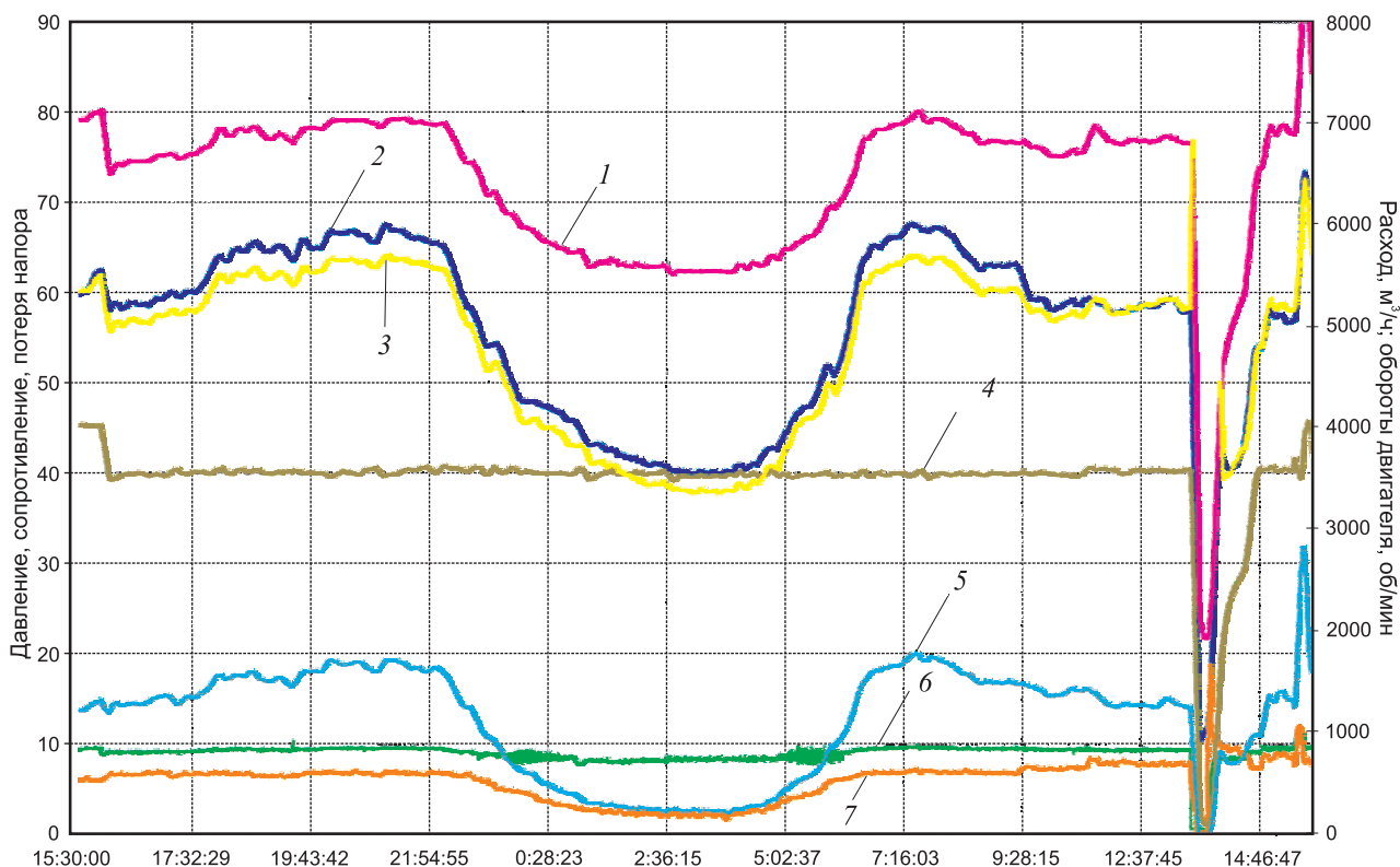
Рис. 5.9. Автоматическое управление системой ПРВ от насосной станции № 25А на жилые массивы
