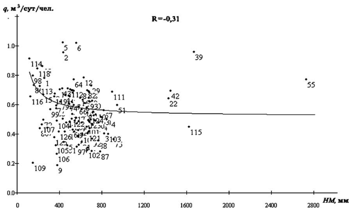
Рис. 4.14. Корреляционная зависимость удельного среднесуточного водопотребления от среднегодового количества осадков
