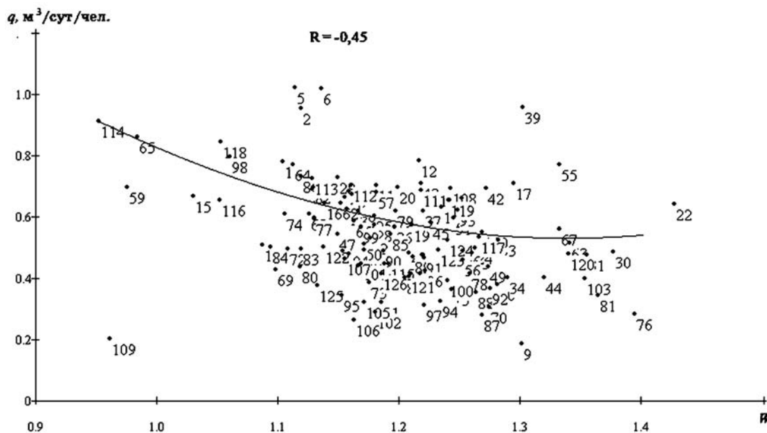
Рис. 4.15. Корреляционная зависимость удельного среднесуточного водопотребления от отношения объема среднегодового водосбора осадков, выпавших на всей площади застройки города, к общей жилой его площади
