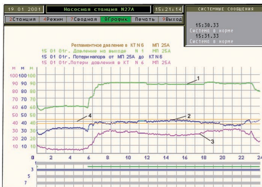
Рис. 6.12. Видеокادر изменения напоров на выходе насосной станции № 25А Харькова и в контрольной точке сети при регулировании по диктующей точке:
