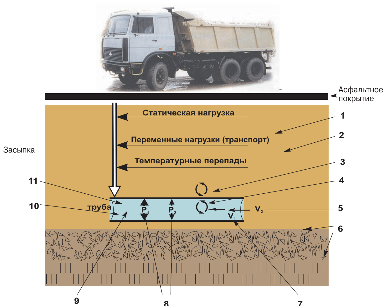
Рис. 6.24. Схема многофакторного влияния на водораспределительную сеть во время ее эксплуатации:
