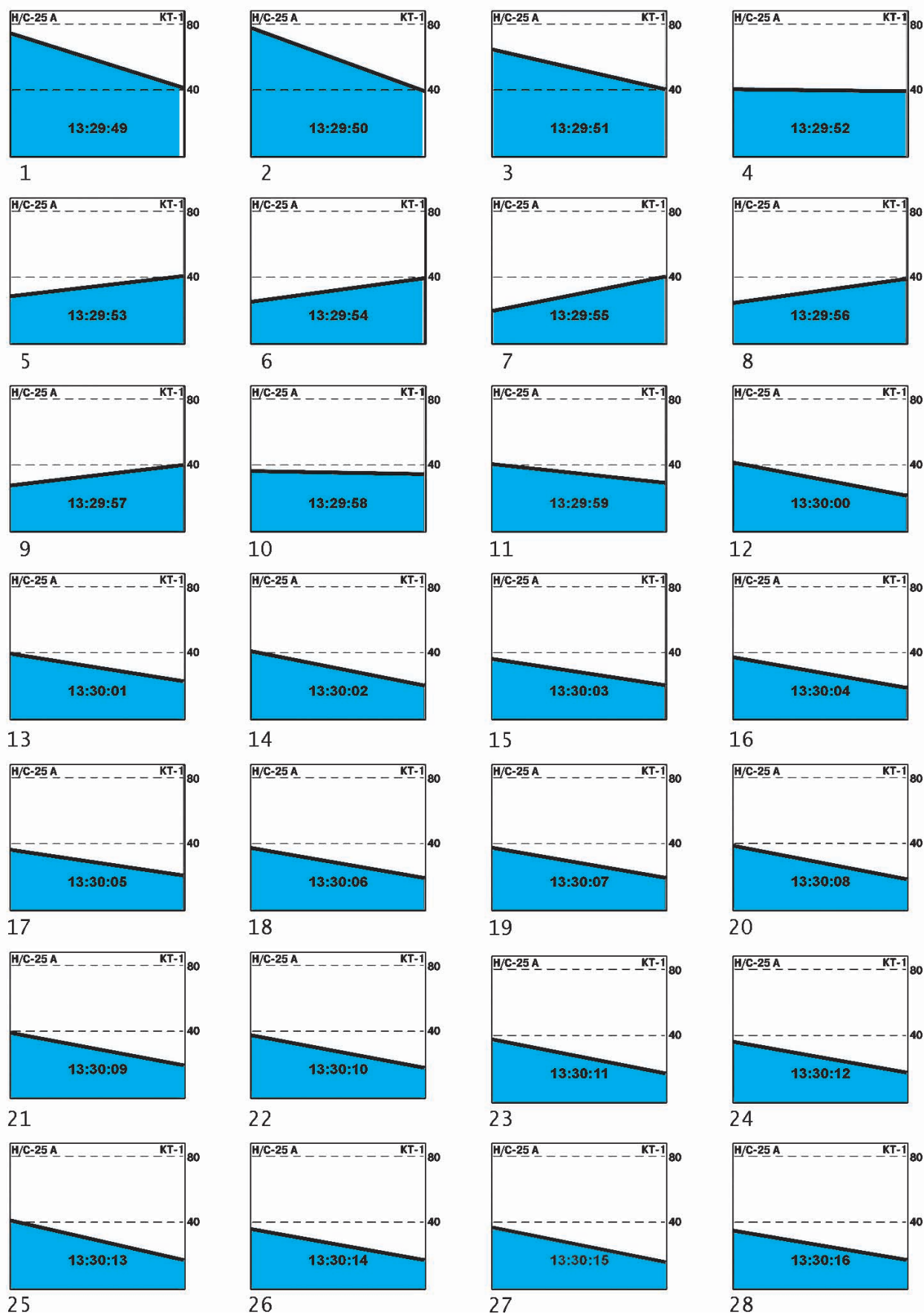
Рис. 6.37. Диаграммы измерений напоров на водосети при отключении насосной станции № 25А от электроэнергетики (гидроударе). Диктующая точка — КТ № 1
