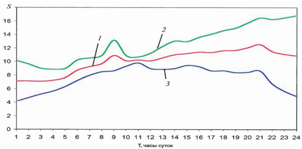
Рис. 5.22. Изменение гидравлического сопротивления системы ПРВ Алексеевского жилого массива от насосной станции № 25А, S = f(T) , для q_{cp} : а — будние дни; б — суббота; в — воскресенье; 1 — S_{cp} ; 2 — S_{cp} + \sigma ; 3 — S_{cp} - \sigma
