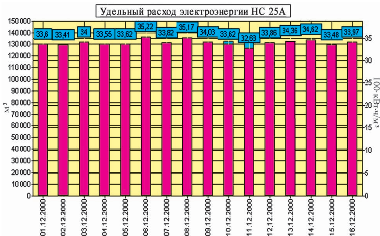
Рис. 6.18. Видеокадр диаграммы удельных расходов электроэнергии по насосной станции за 16 суток декабря 2000 г.
