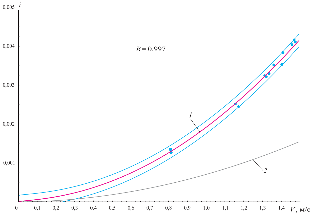
Рис. 3.47. Регрессионная зависимость i=f(V) для водовода диаметром 1600 мм; L = 6558 м с доверительным интервалом регрессии P = 95\% : 1 — по формуле (3.43); 2 — по Шевелеву
