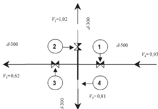
Рис. 6.8. Узел водосети
