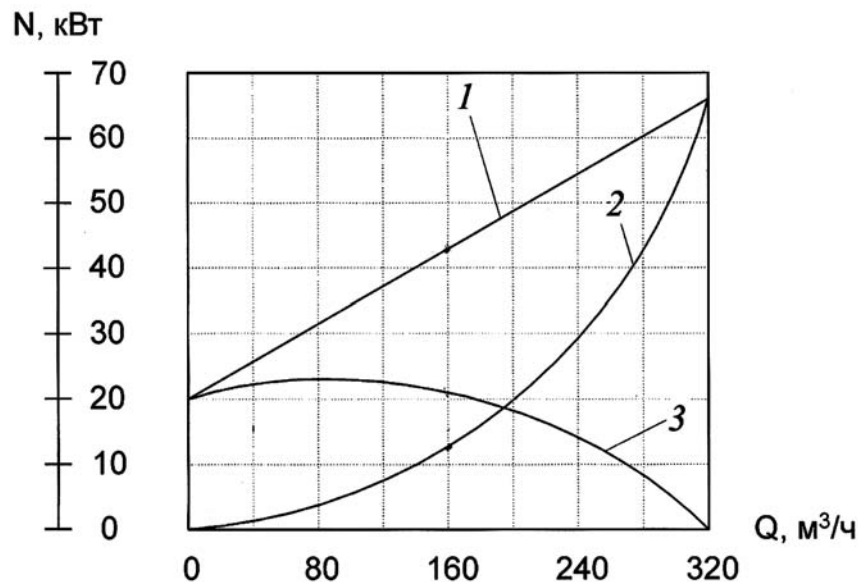
Рис. 5.8. Потребление мощности при различных способах регулирования скорости вращения насосов:
