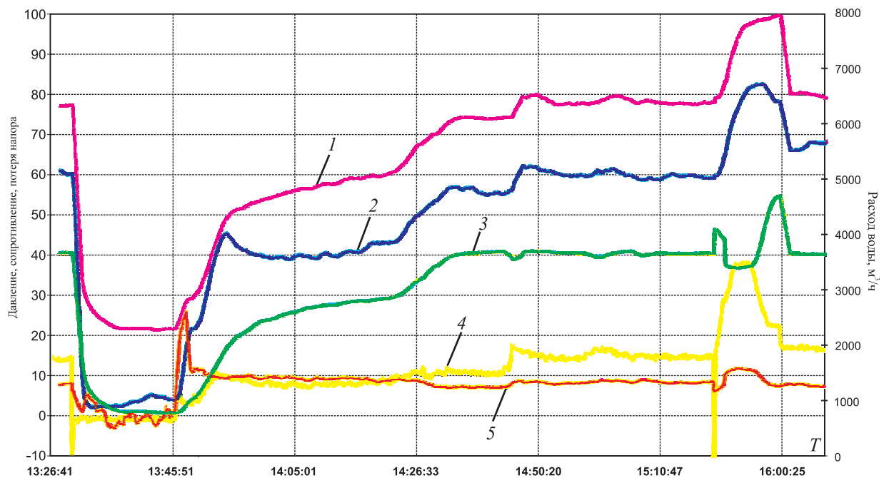
Рис. 5.16. Фрагмент изменения режимов в системе ПРВ от насосной станции № 25А в период гидроудара (13:29:48,1 – 13:30:00) и аварии (15:25:00 – 15:30:00):
