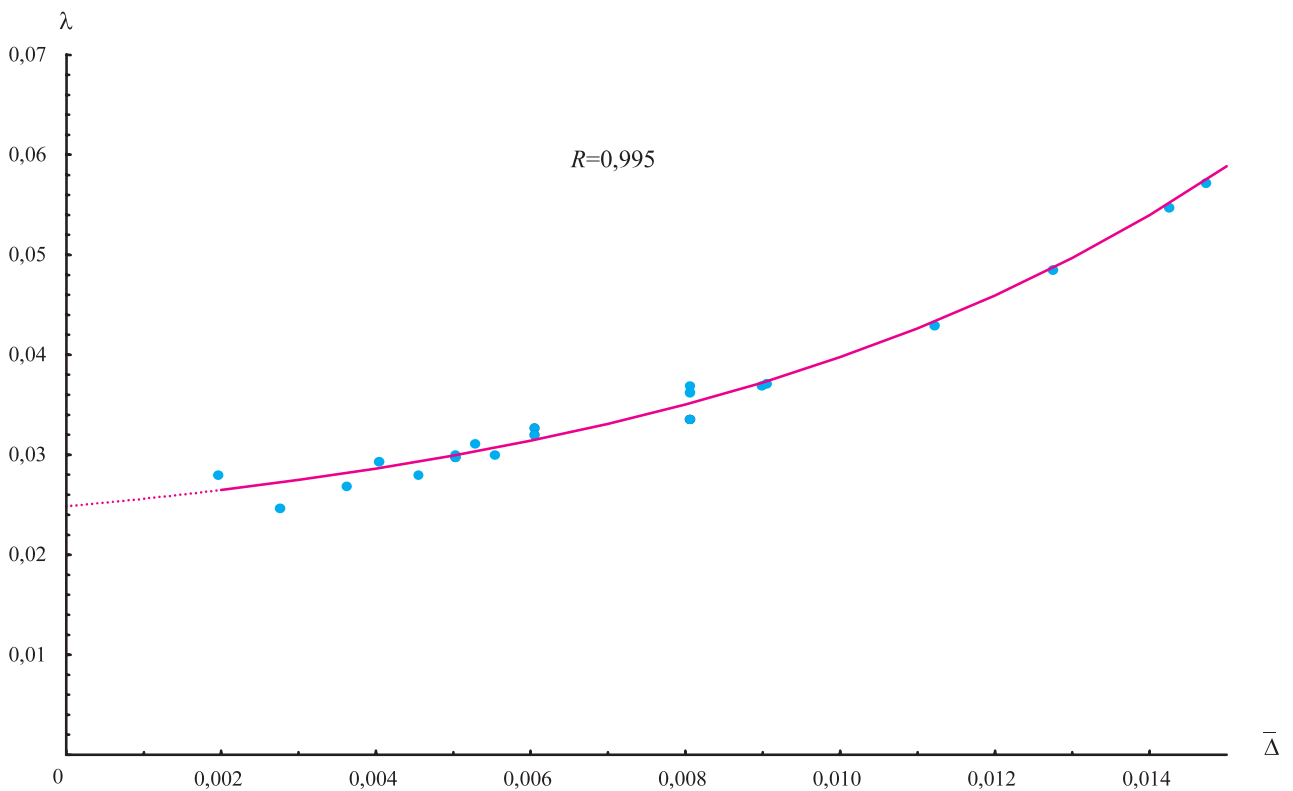
Рис. 3.35. Регрессионная зависимость \lambda = f(\bar{\lambda}) с доверительным интервалом регрессии P = 95 \% (водовод диаметром 1200 мм; L = 14\,902 м)
