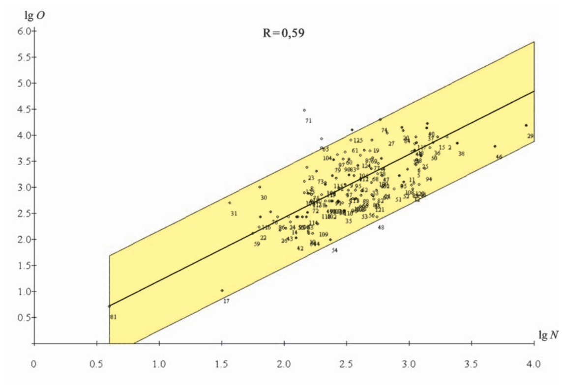
Рис. 4.20. Корреляционная зависимость между ореолом загрязнения и численностью населения
