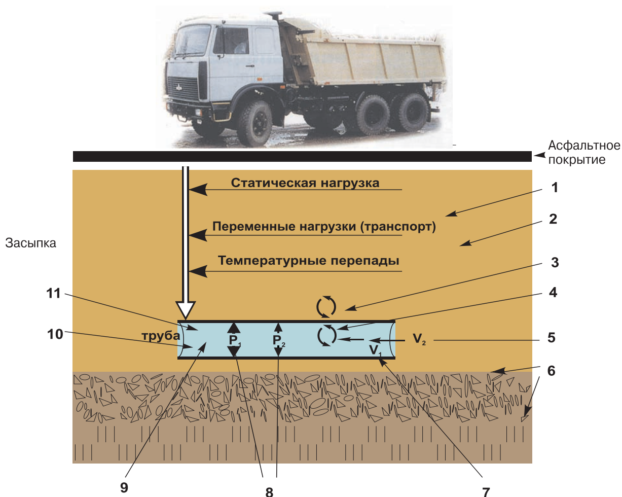
Рис. 6.24. Схема многофакторного влияния на водораспределительную сеть во время ее эксплуатации: 1 — влажность грунта; 2 — электрические поля (потенциал); 3 — наружная коррозия; 4 — внутренняя биохимическая коррозия; 5 — изменение скорости потока воды; 6 — характеристика грунта; 7 — материал трубы; 8 — изменение внутреннего давления; 9 — температура воды; 10 — наличие кислорода в воде; 11 — pH воды
