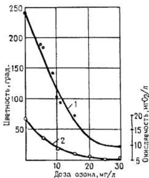
Рис. 7. Эффективность очистки цветных вод озонированием (г. Приморско-Ахтарск Краснодарского края):
